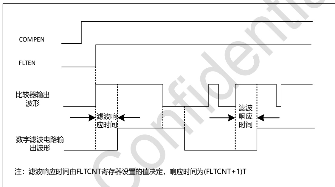
图 15-2 COMP 滤波示意图
