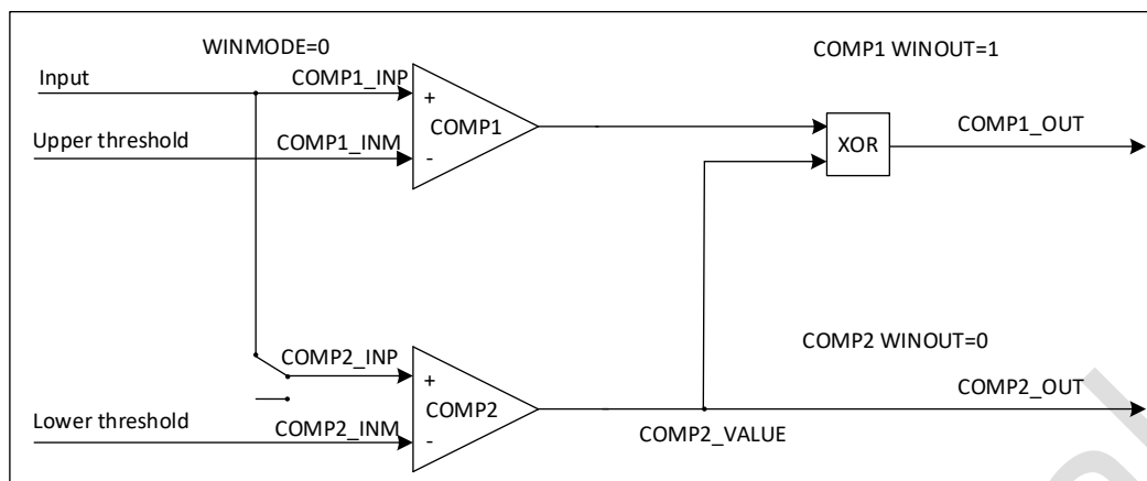
图 15-4 窗口比较器
