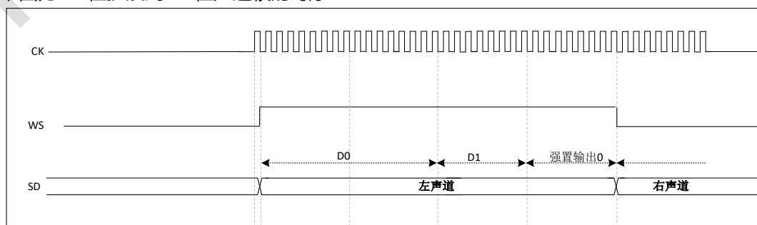
图 34-22 I²S MSB 对齐标准(16 位扩展到 32 位, CKPOL=0)
