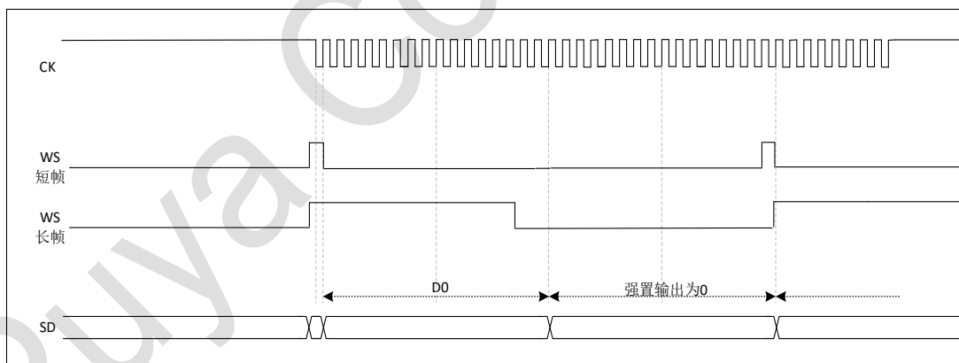
图 34-33 I²S PCM 标准 (16 位扩展到 32 位, CKPOL=1)
