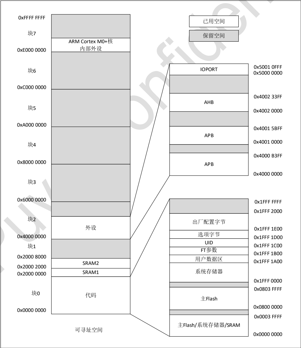
图 3-2 存储器映射
