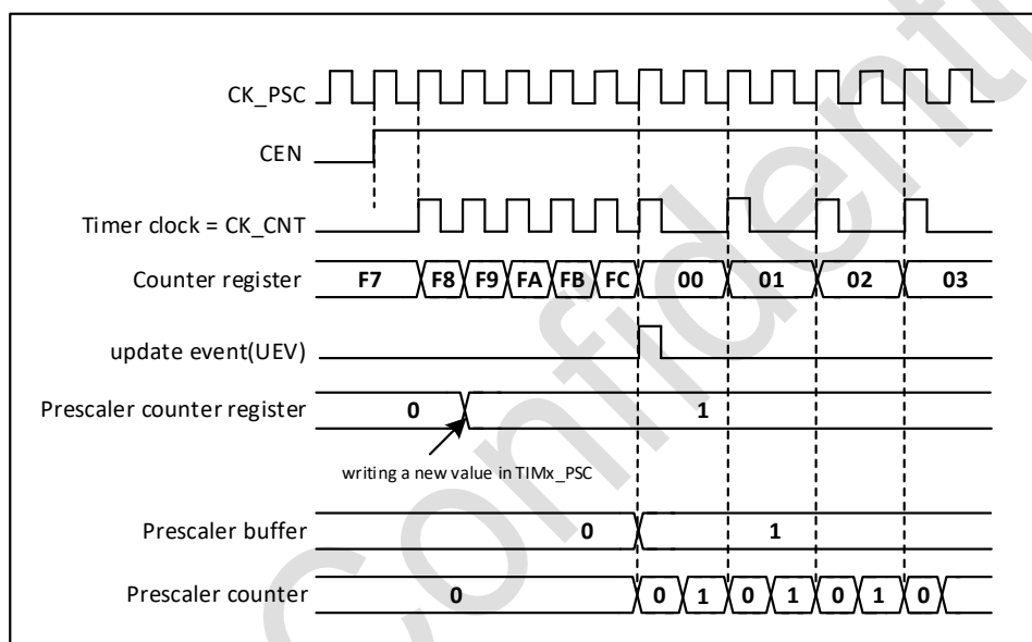
图 22-2 预分频器分频由 1 变为 2 时的计数器时序图
