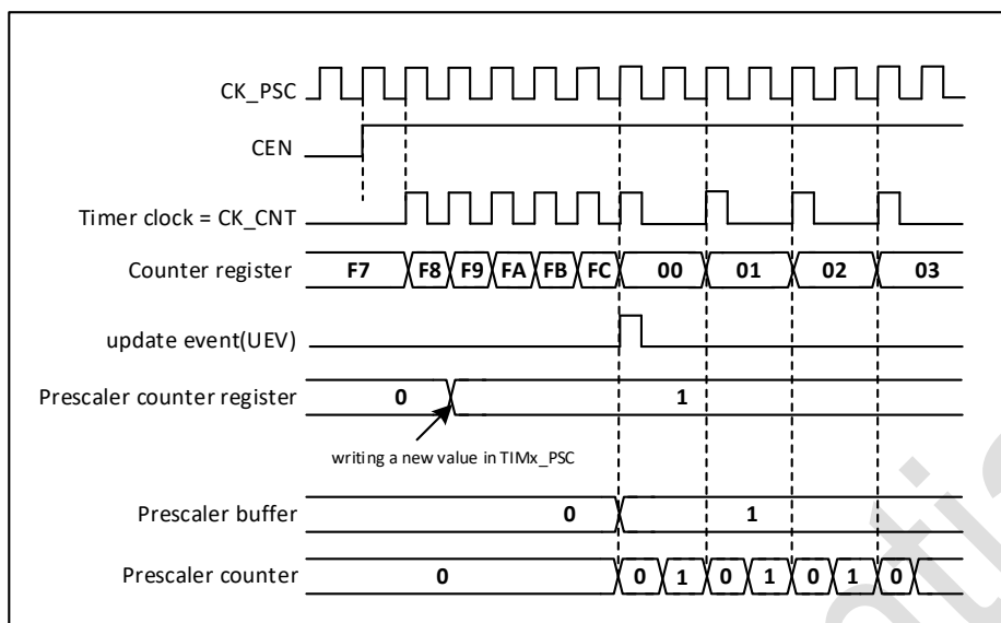
图 20-2 预分频器分频由 1 变为 2 时的计数器时序图
