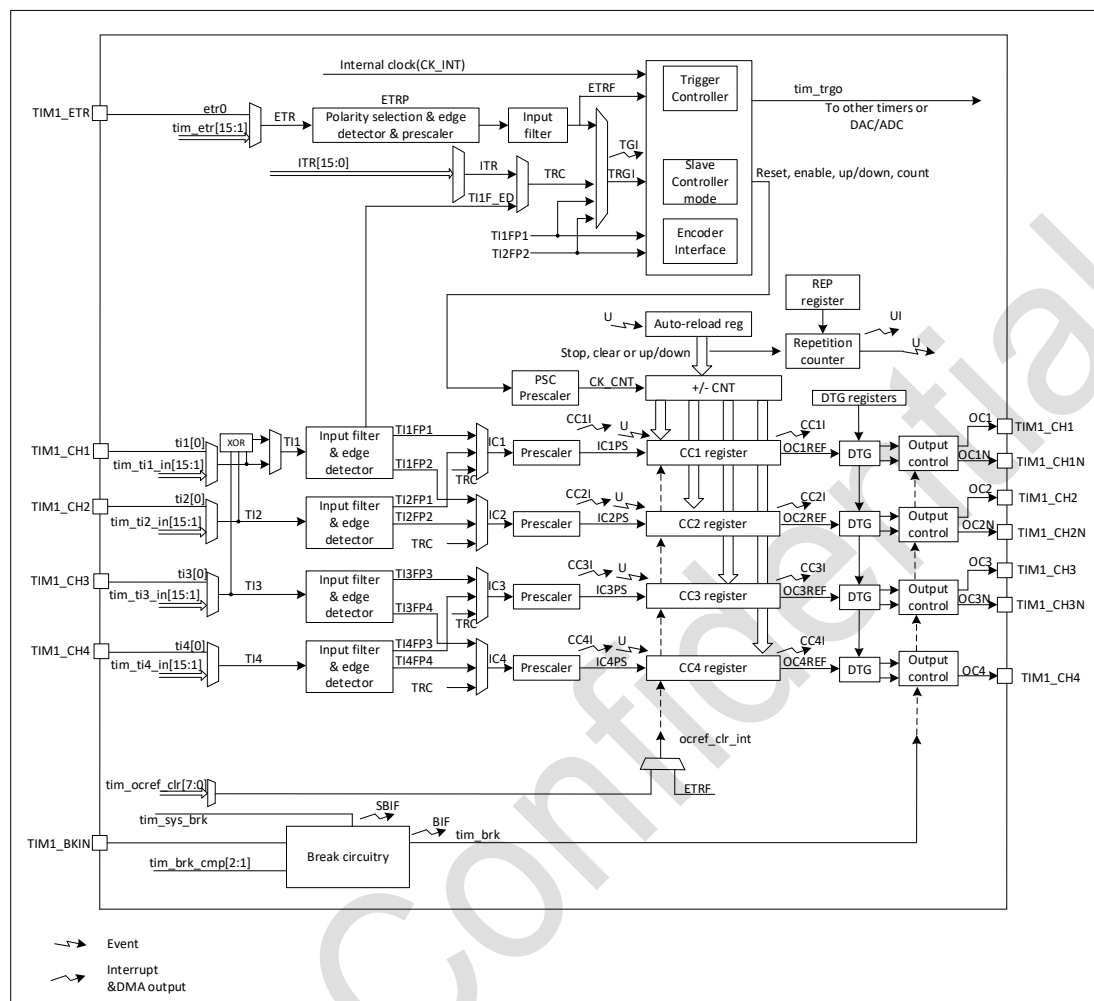
图 18-1 高级控制定时器框图
