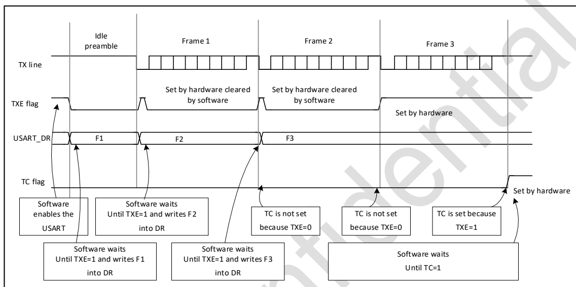
图 31-4 发送时的 TC/TXE 行为
