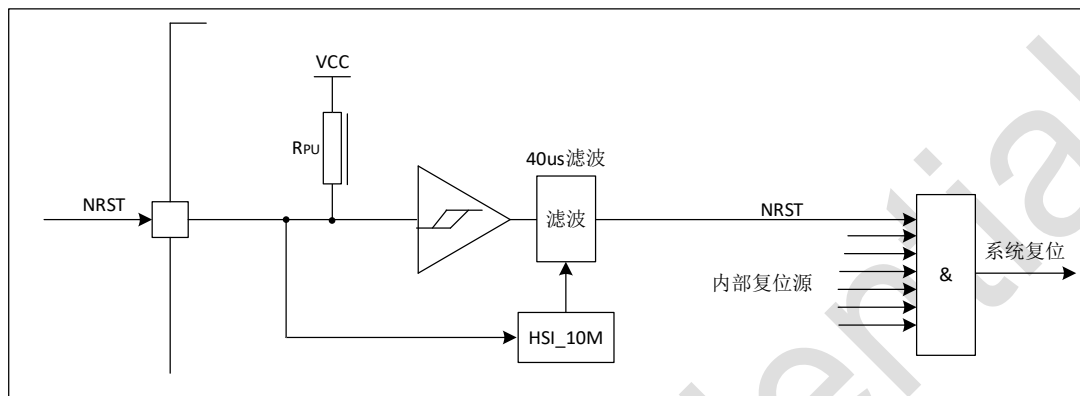
图 6-1 复位电路
