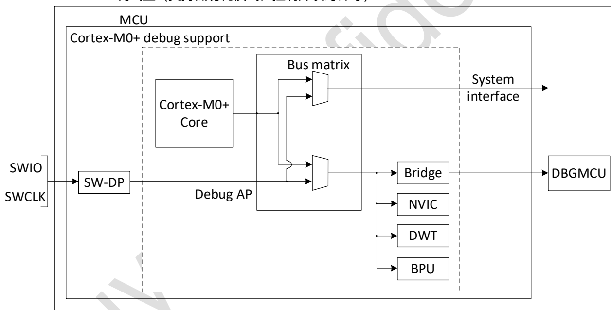
图 36-1 DBG 框图
