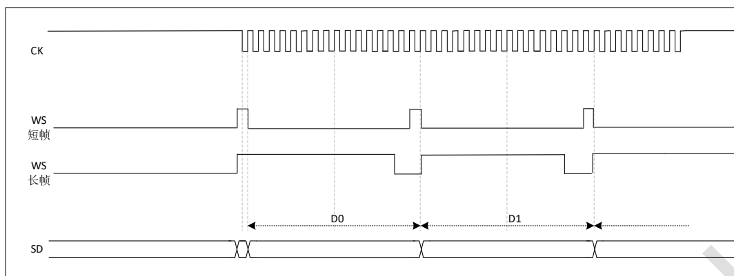
图 34-31 I²S PCM 标准 (16 位帧, CKPOL=1)
