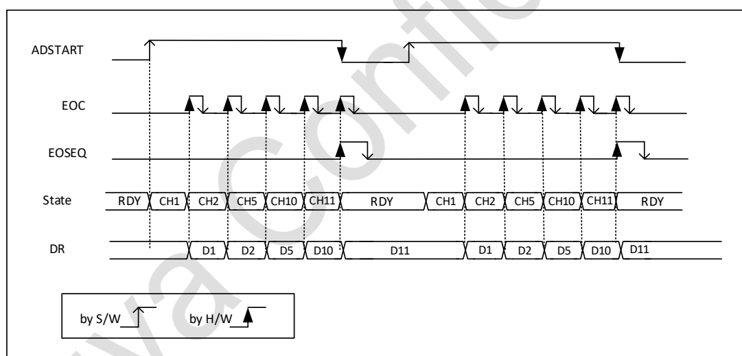
图 13-10 规则单次模式, 软件触发
