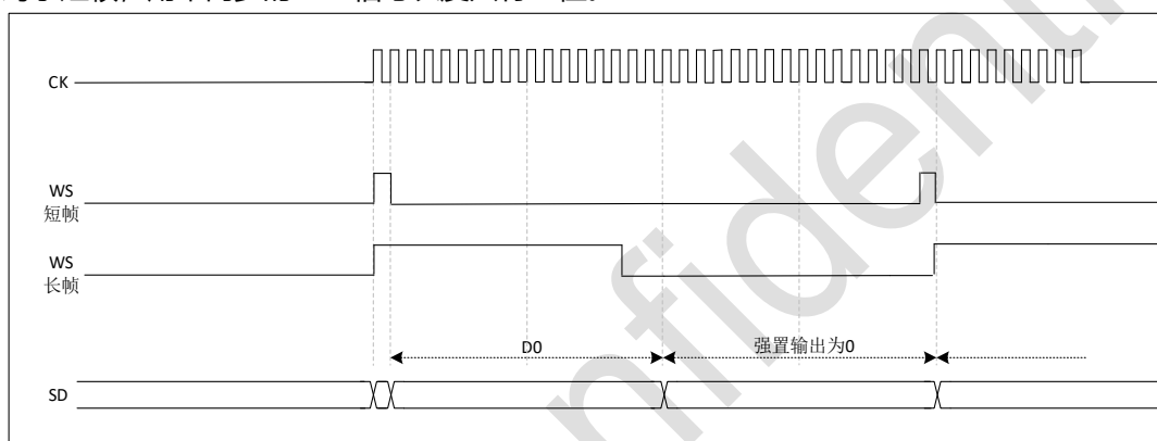
图 34-32 I²S PCM 标准(16 位扩展到 32 位, CKPOL=0)
