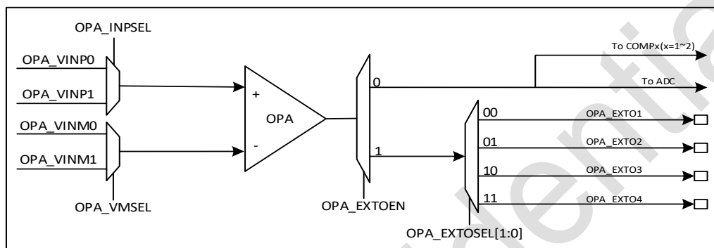
图 16-1 OPA 框图
