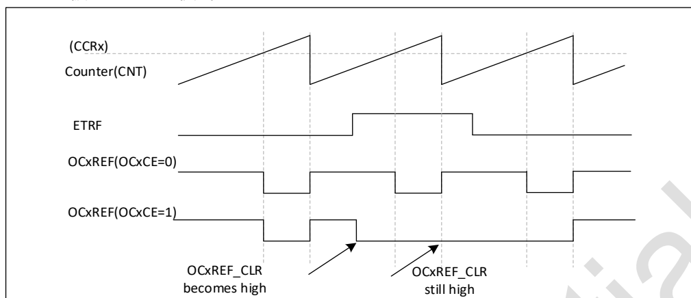
图 19-33 清除 TIMx 的 OCxREF
