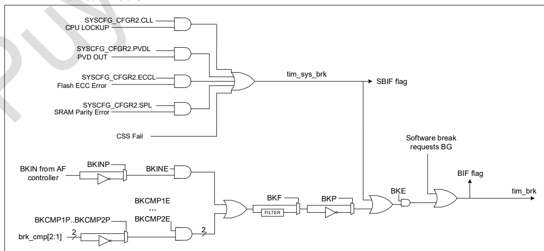
图 20-25 刹车电路图
