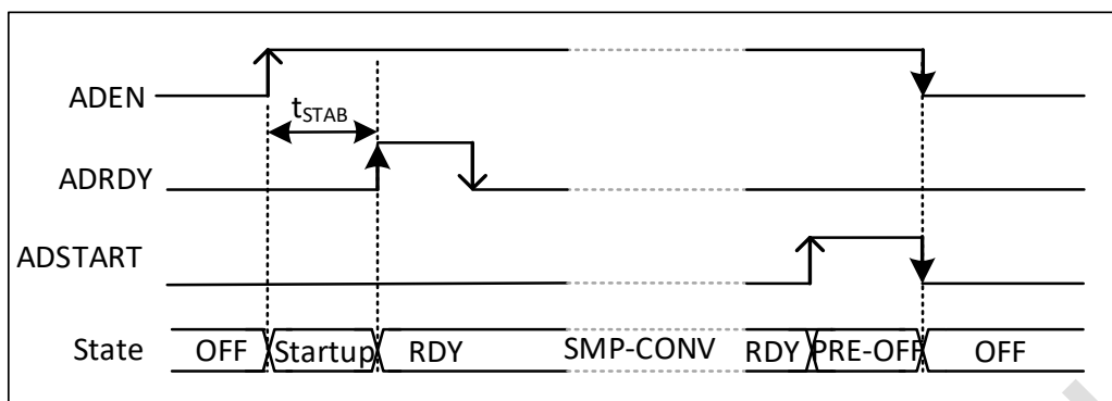
图 13-4 使能/禁止 ADC
