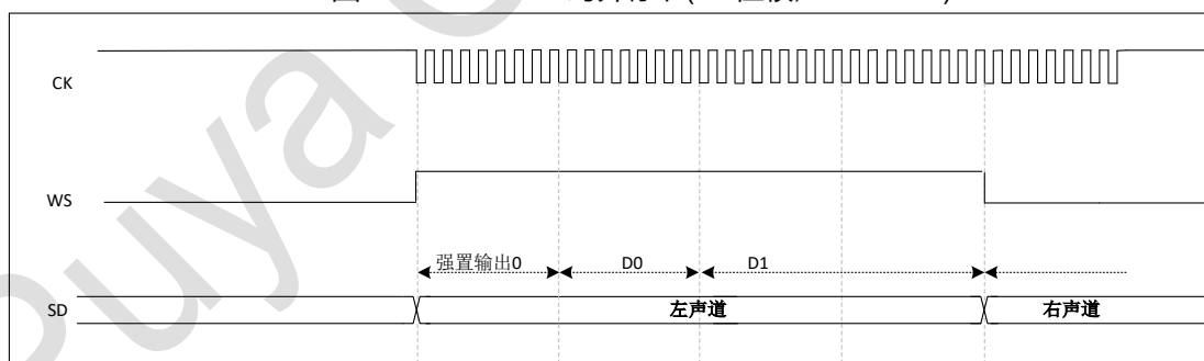
图 34-26 I²S LSB 对齐标准(24 位帧, CKPOL=0)
