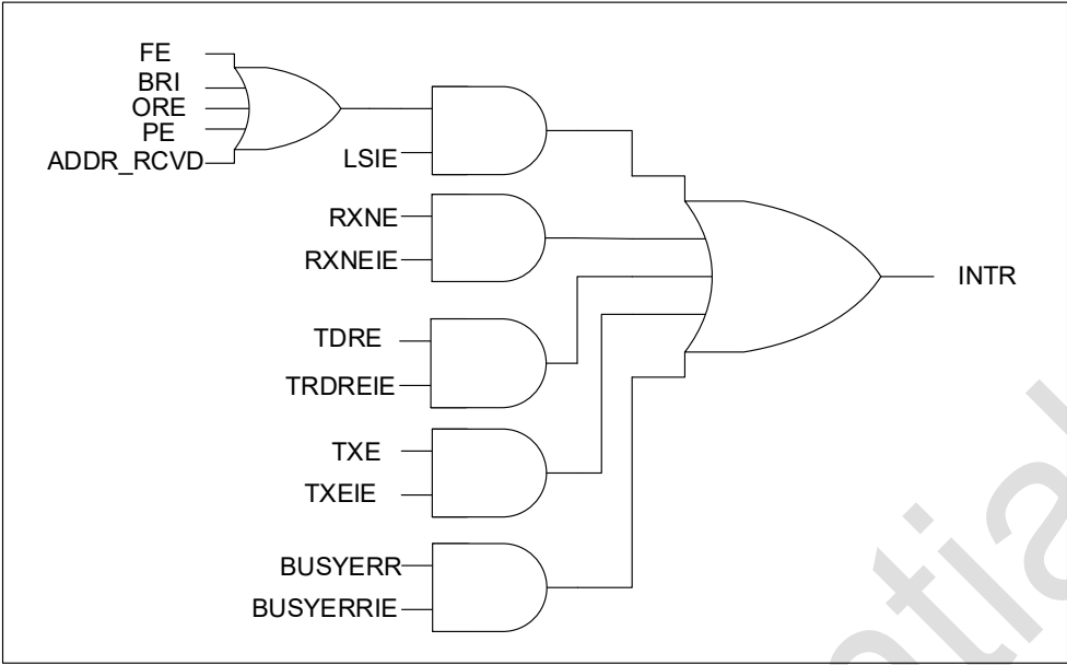
图 32-8 中断映射图
