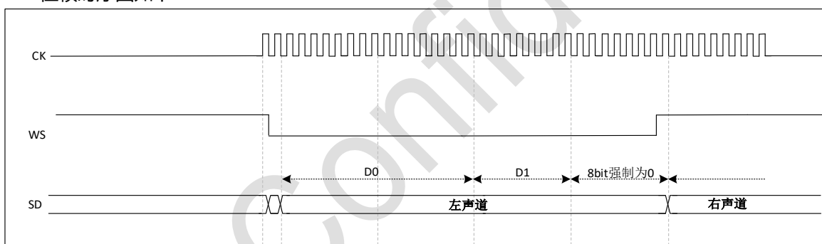
图 34-15 I 2 S 飞利浦协议波形(24 位帧, CKPOL=0)
