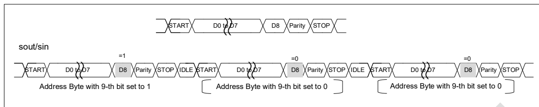
图 32-5 9位字符
