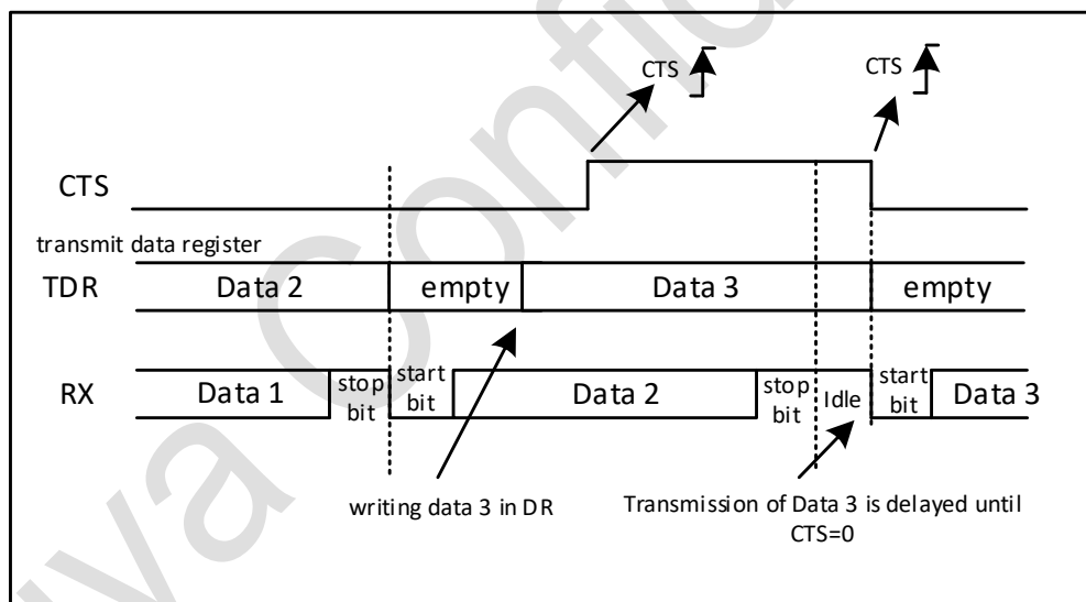
图 31-17 CTS 流控制
