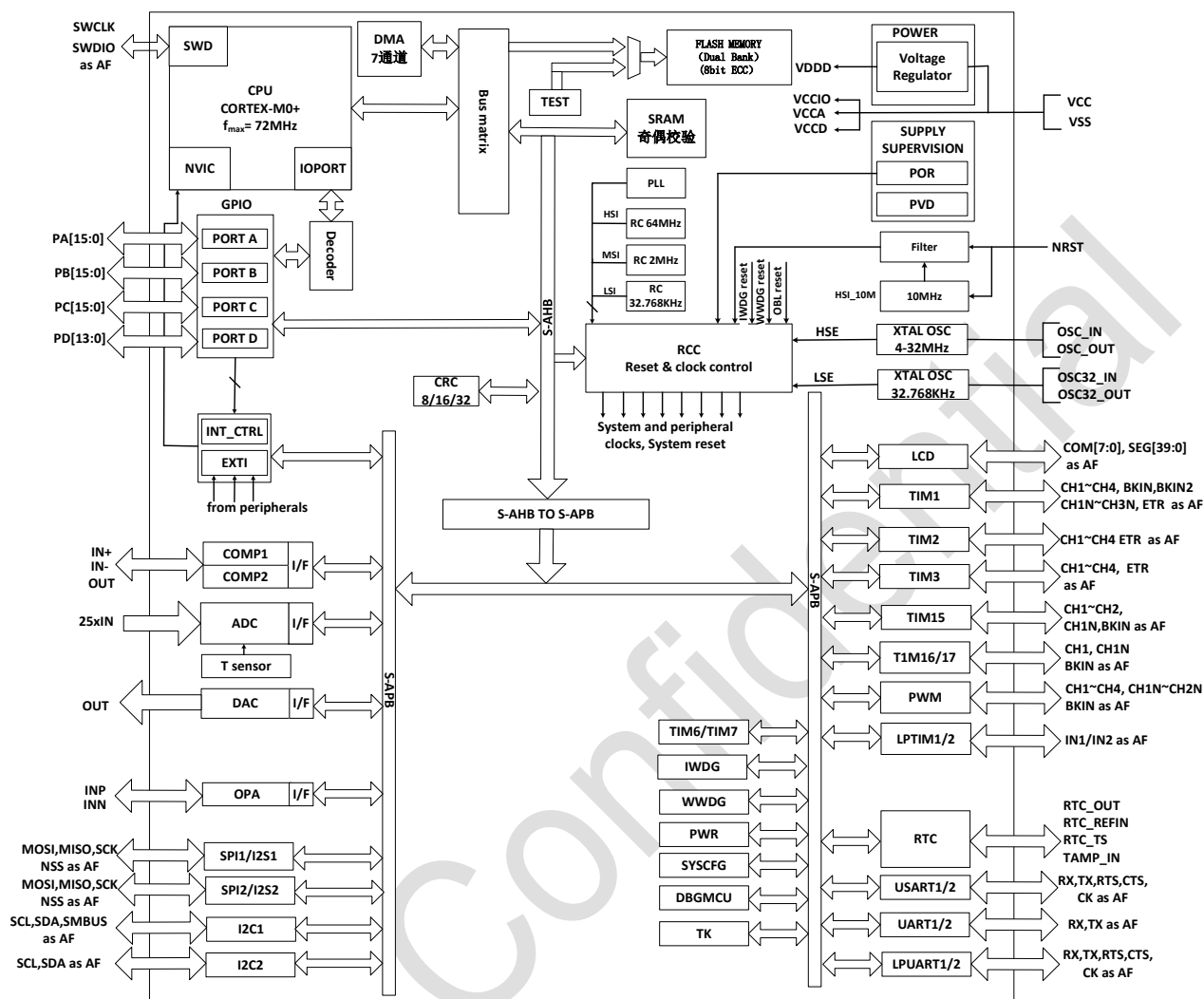
图 2-1 系统框图
