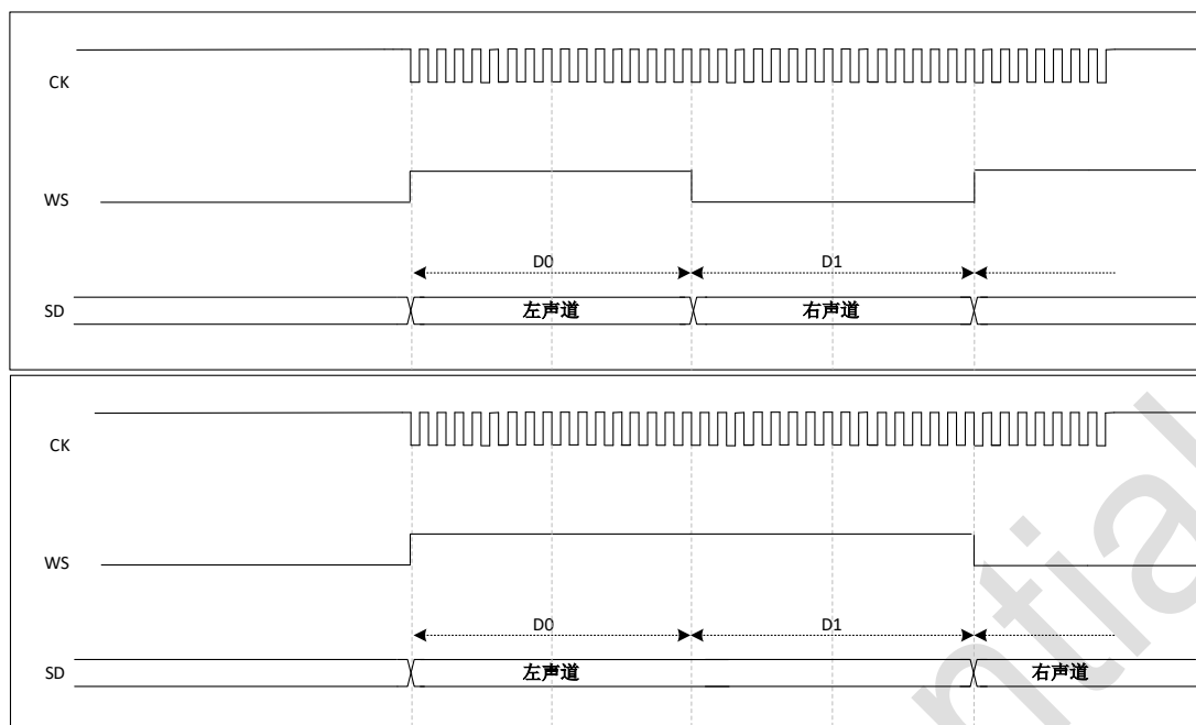
图 34-25 I²S LSB 对齐标准 (16/32 位全精度, CKPOL=1)
