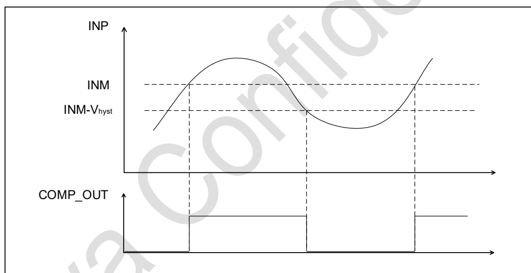
图 15-5 比较器迟滞
