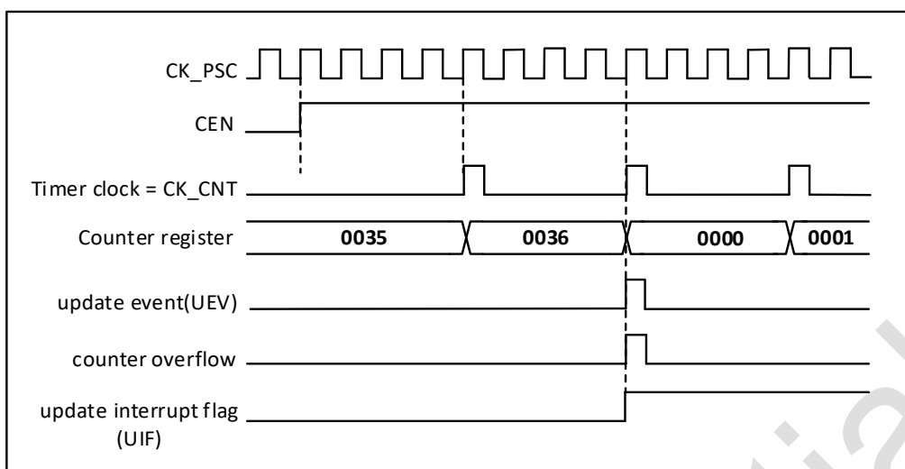
图 18-6 计数器时序图, 内部时钟 4 分频
