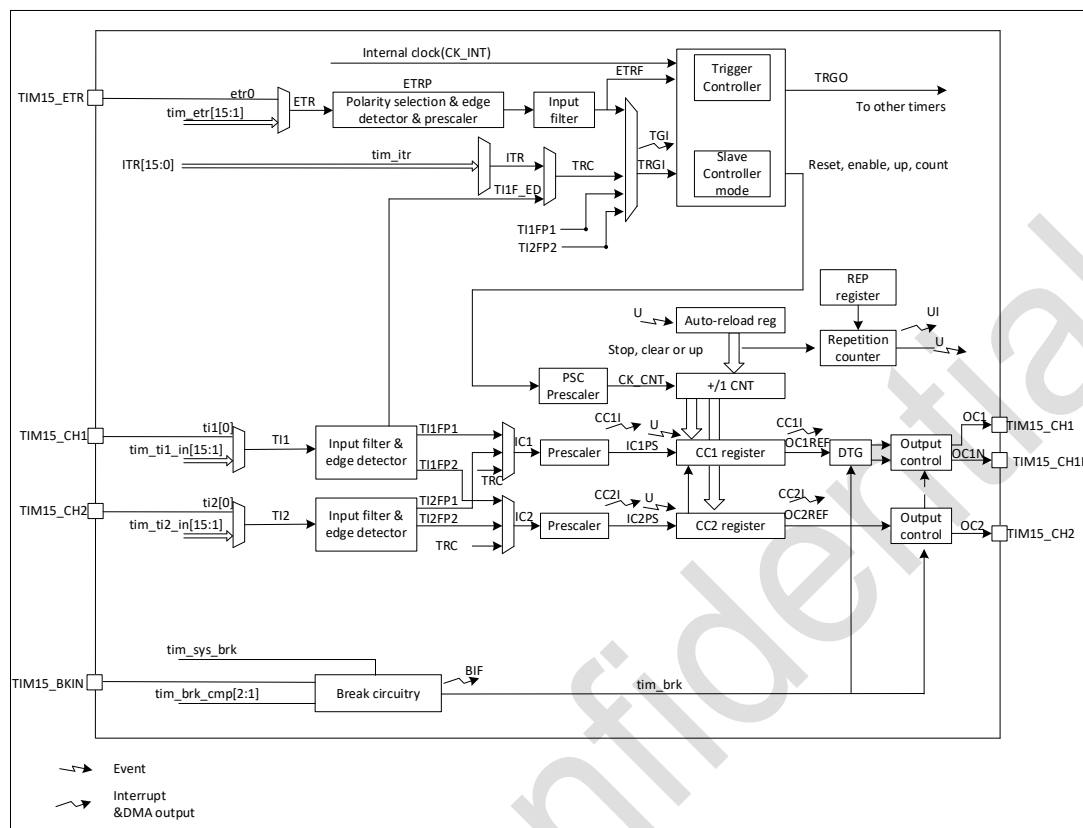
图 20-1 TIM15 框图
