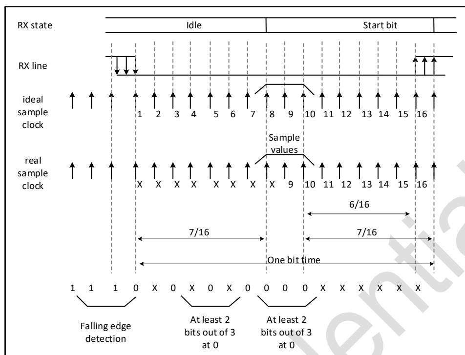
图 31-5 起始位检测
