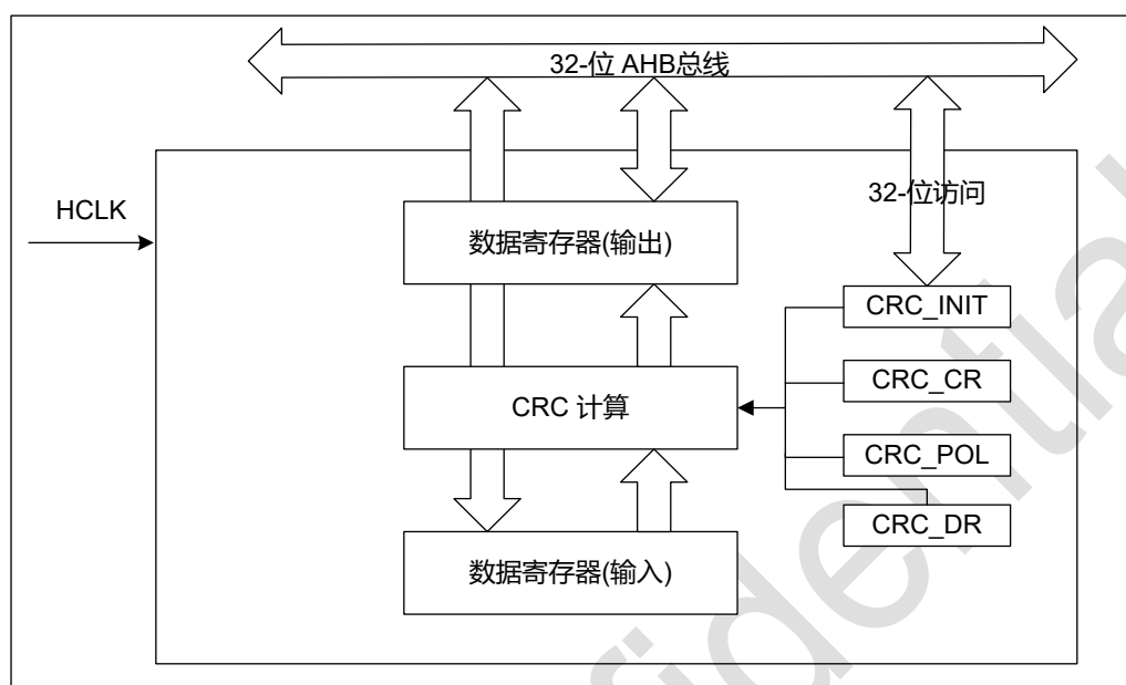
图 12-1 CRC 框图
