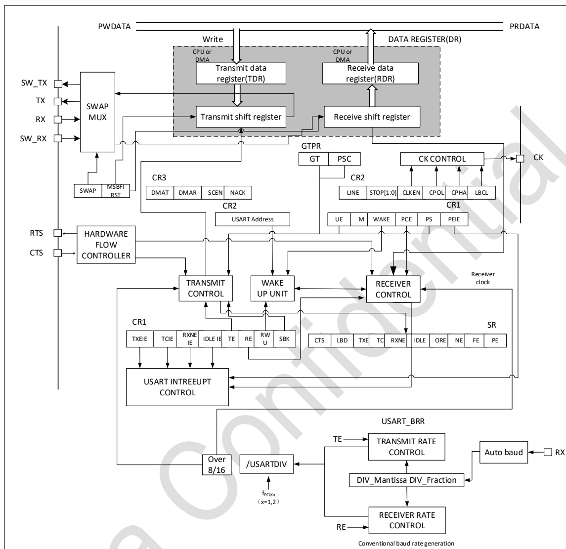
图 31-1 USART 框图
