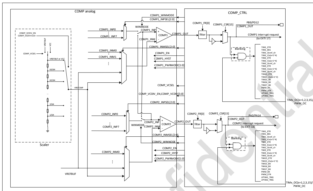
图 15-1 COMP 框图
