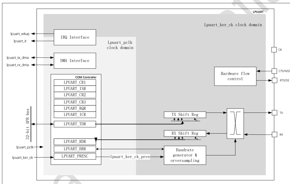
图 33-1 LPUART 框图
