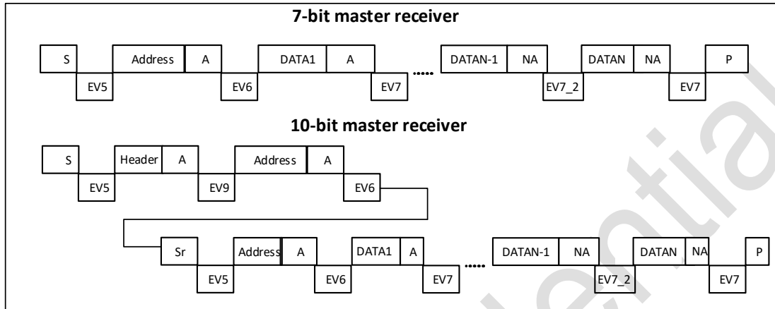
图 30-7 方法 2: 主机接收传输序列 N>2
