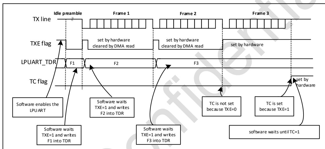
图 33-3 发送时的 TC/TXE 行为
