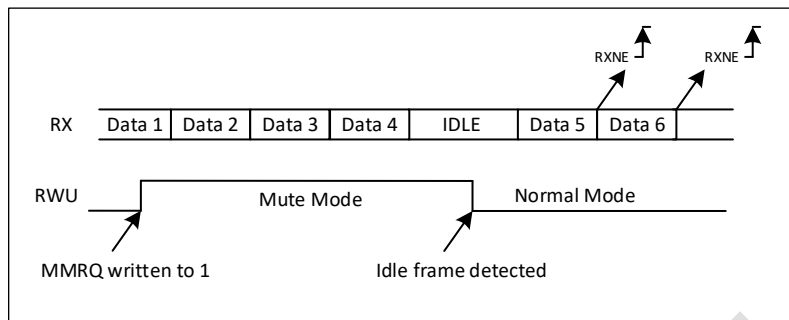
图 33-4 用总线帧检测的静默模式
