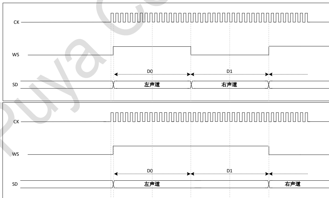
图 34-18 I²S MSB 对齐标准 (16/32 全精度, CKPOL=0)
