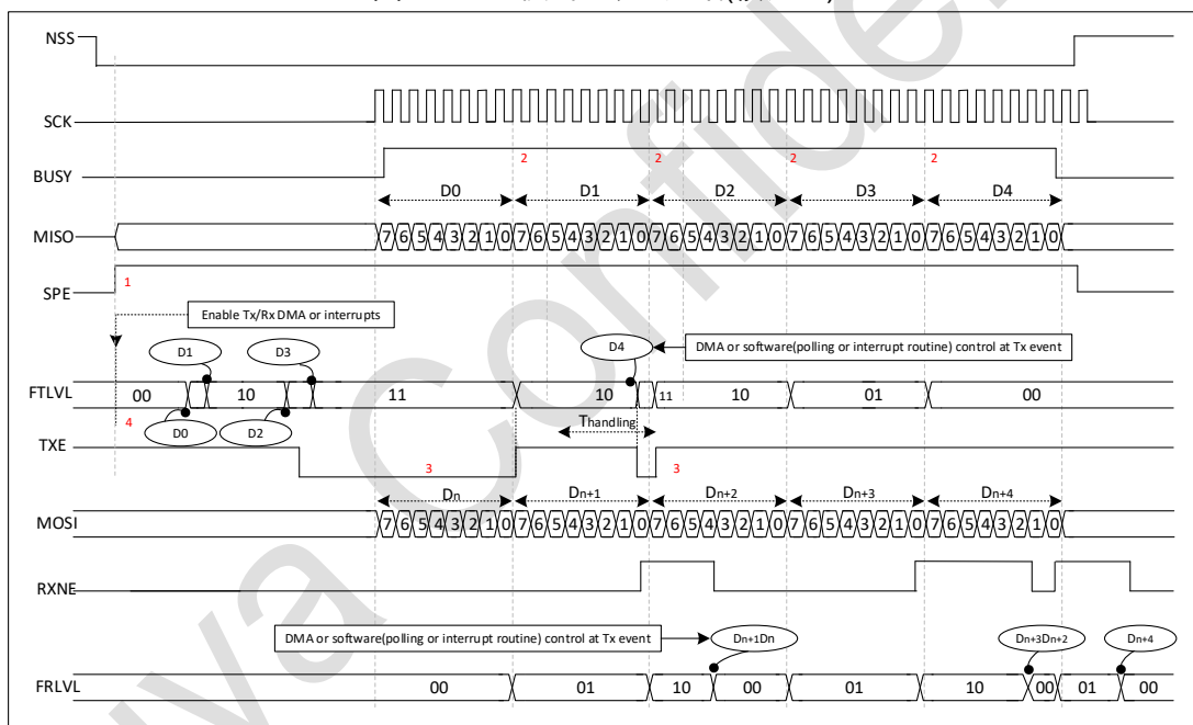
图 34-10 从模式全双工通讯(帧长=8)
