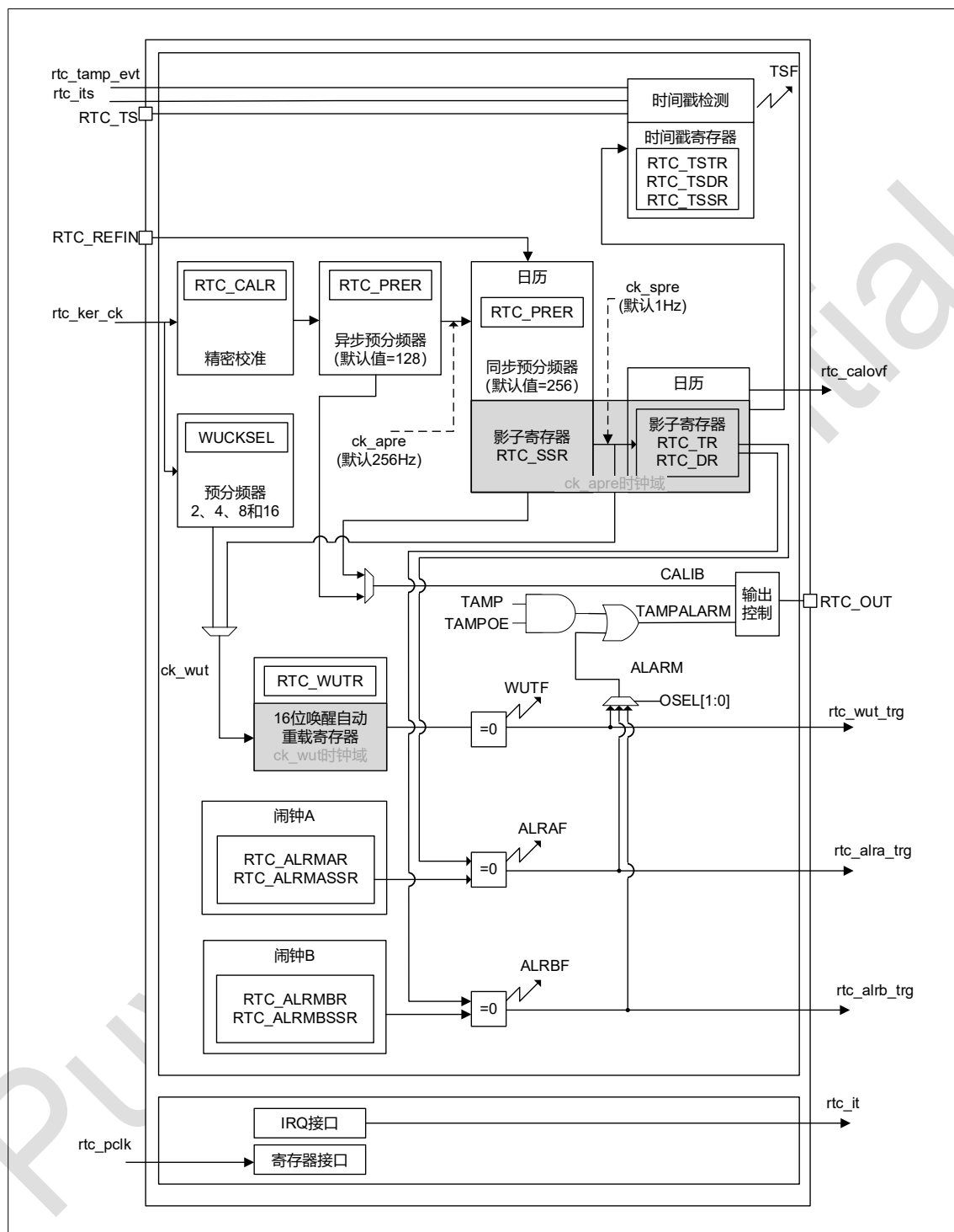
图 28-1 RTC 框图
