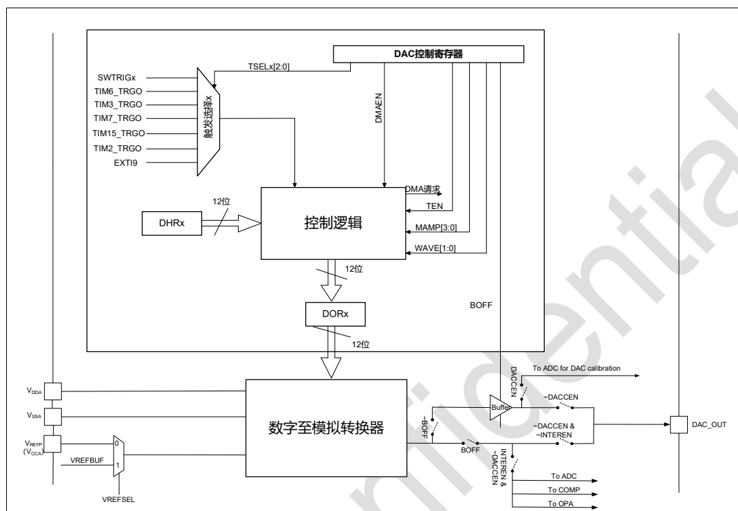
图 14-1 DAC 框图
