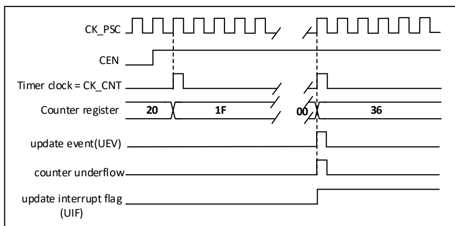
图 18-13 计数器时序图，内部时钟 N 分频
