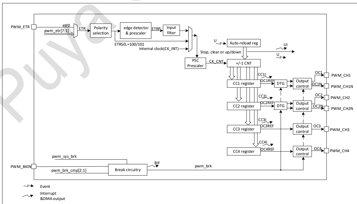
图 23-1 PWM 框图
