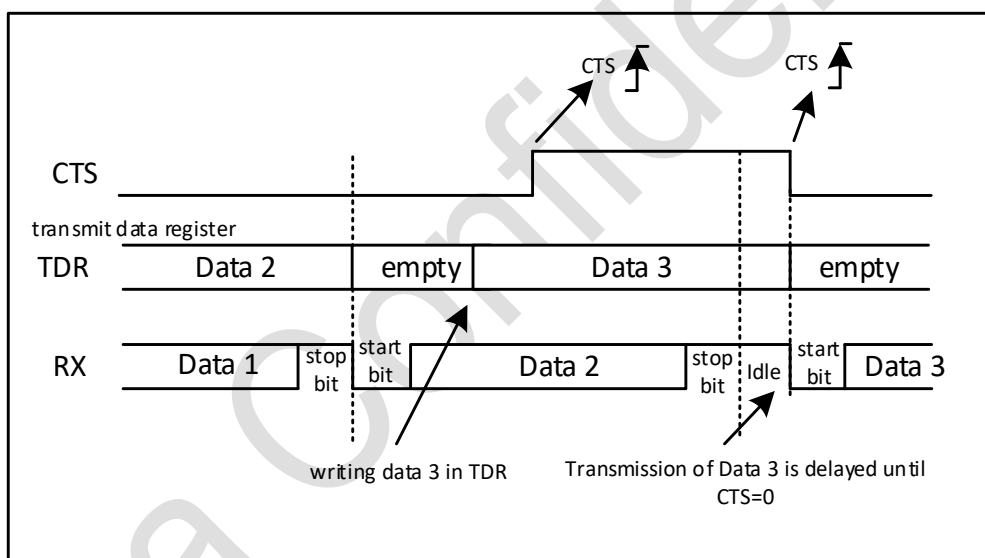
图 33-10 CTS 流控制
