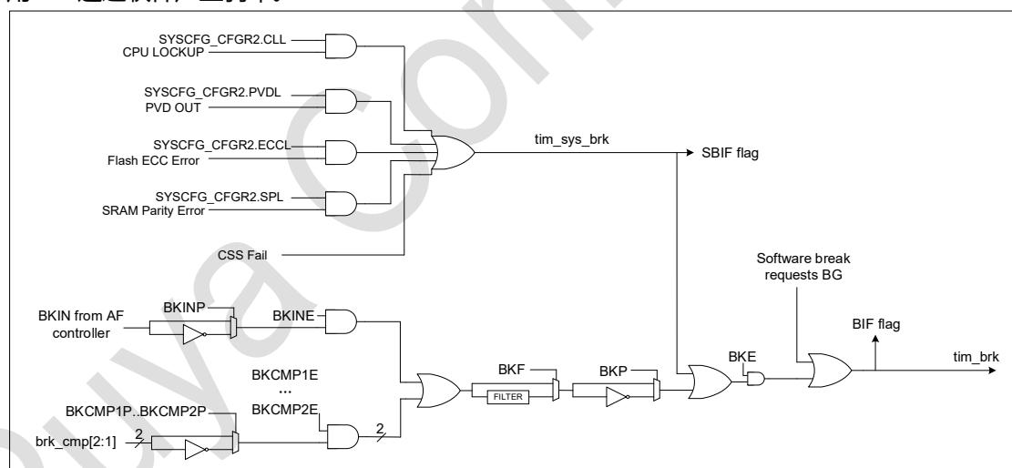
图 18-39 刹车电路图
