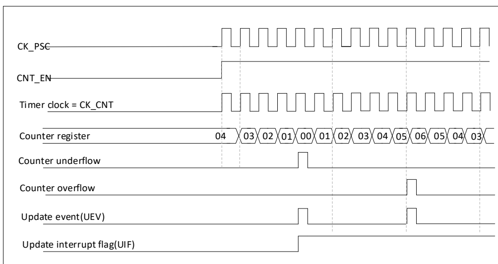
图 17-15 计数器时序图, 内部时钟 1 分频, TIM1_ARR = 0x6
