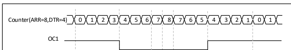
图 22-2 中心对齐模式 PWM 输出(ARR=8)
