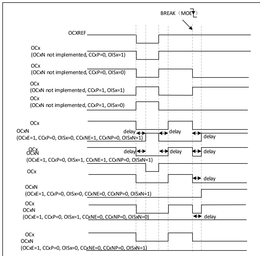
图 17-40 响应刹车事件的不同输出行为 (OSSI=1)
