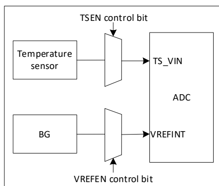
图 12-28 TS 和 VREFINT 通道
