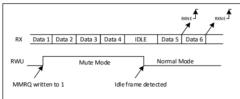
图 32-4 用总线帧检测的静默模式
