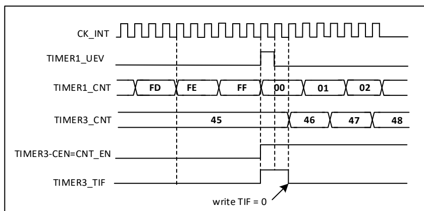
图 18-44 TIM1 的更新时间使能 TIM3
