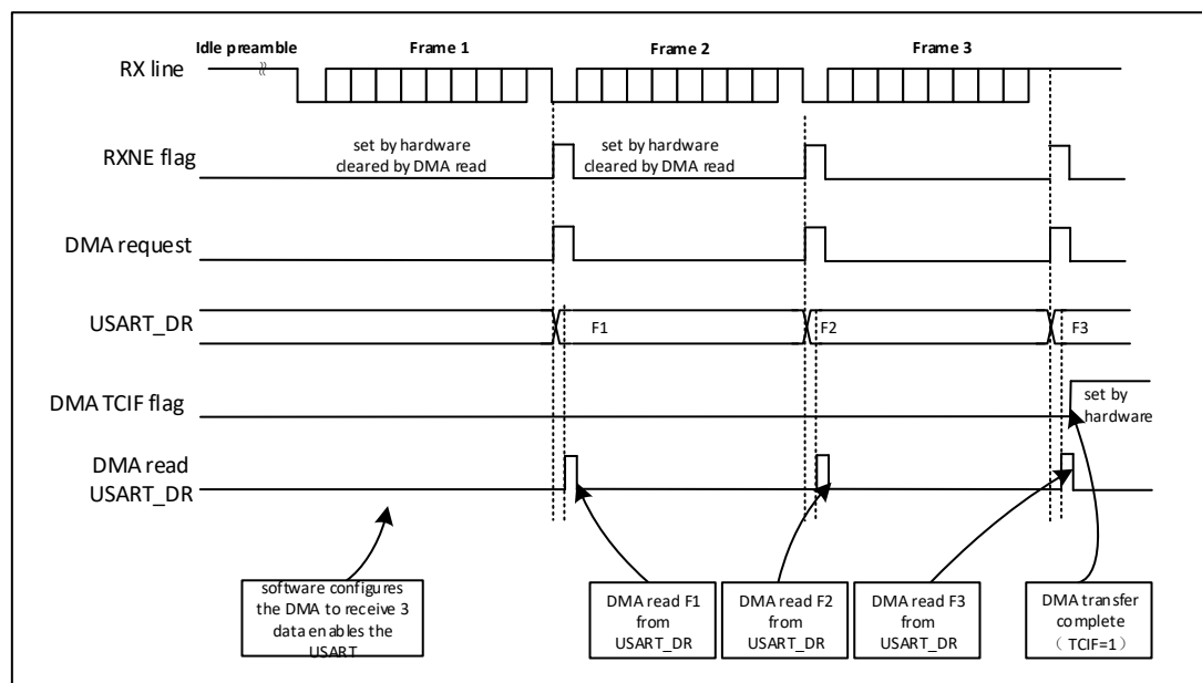
图 30-14 使用 DMA 接收
