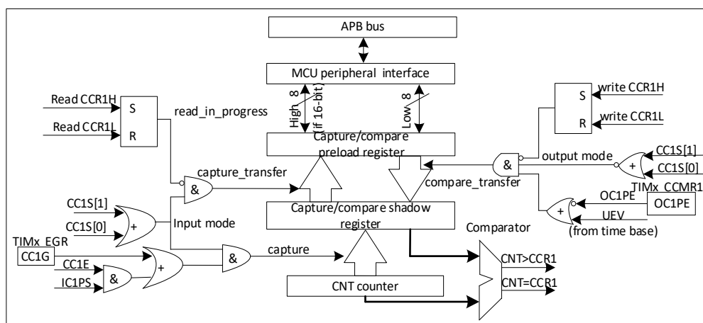
图 20-13 捕获/比较通道 1 主电路
