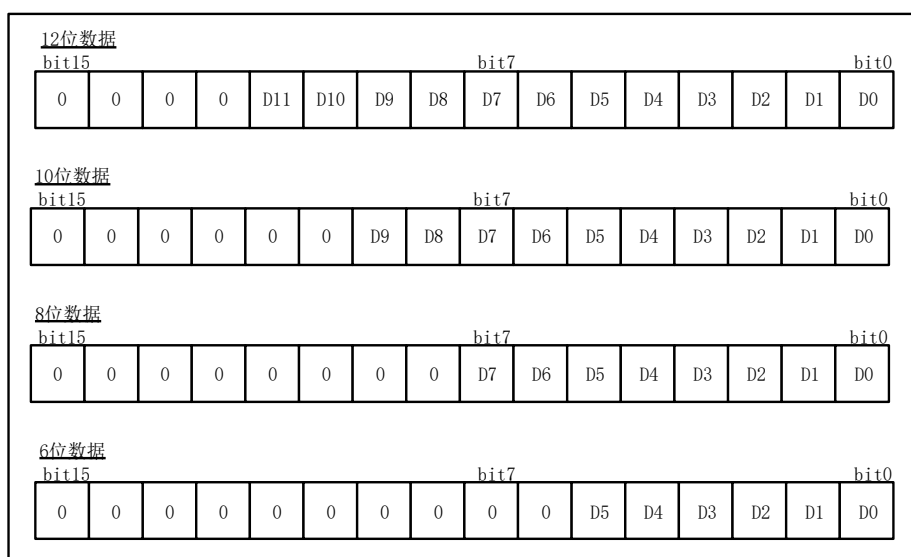
图 12-13 右对齐 (offset 未使能, 无符号数)
