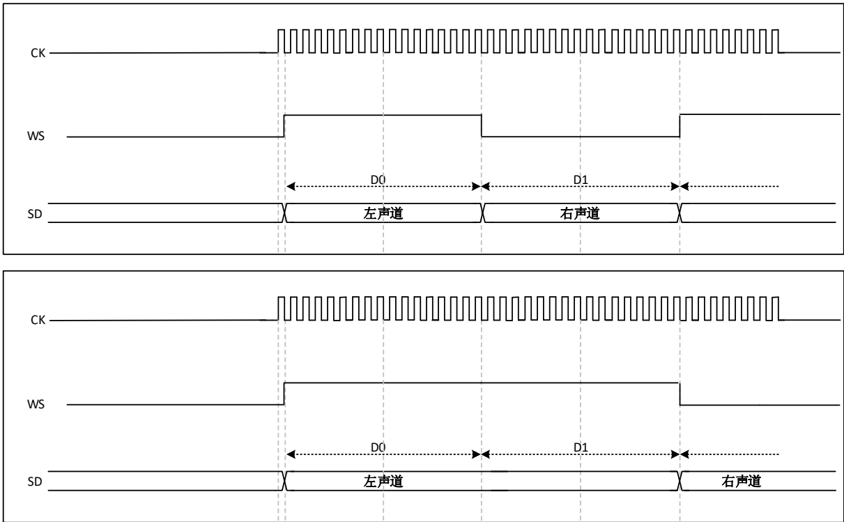
图 33-23 I2S LSB 对齐标准 (16/32 位全精度, CKPOL=0)
