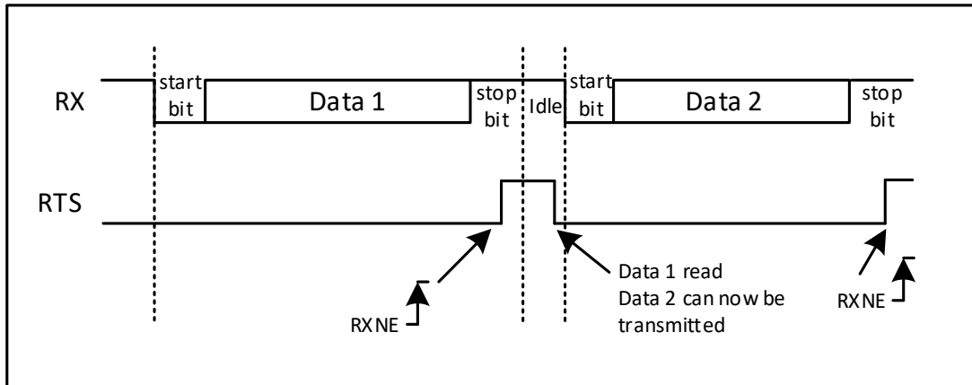
图 30-16 RTS 流控制
