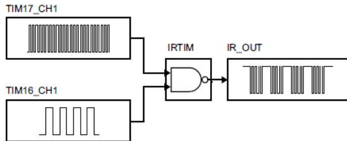
图 23-1 IRTIM implement
