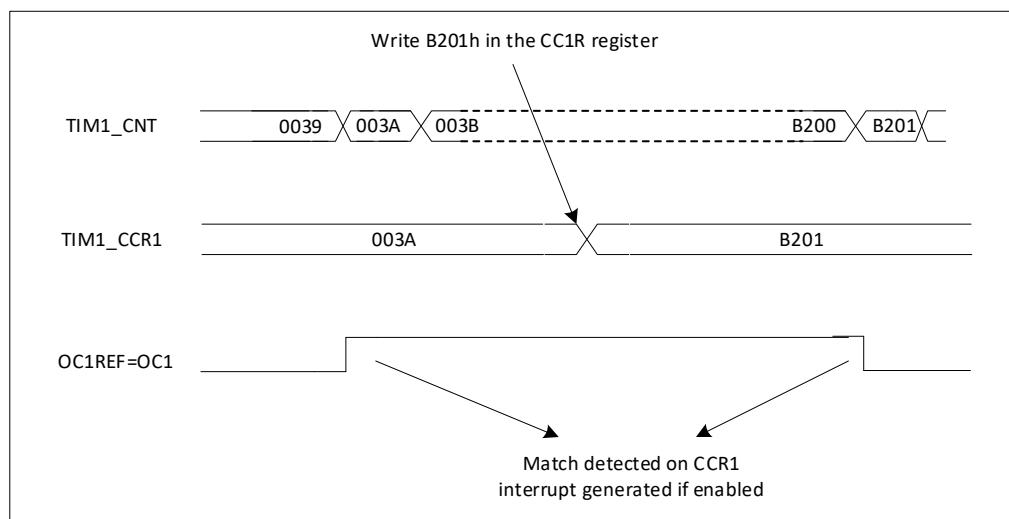
图 19-20 输出比较模式, 翻转 OC1
