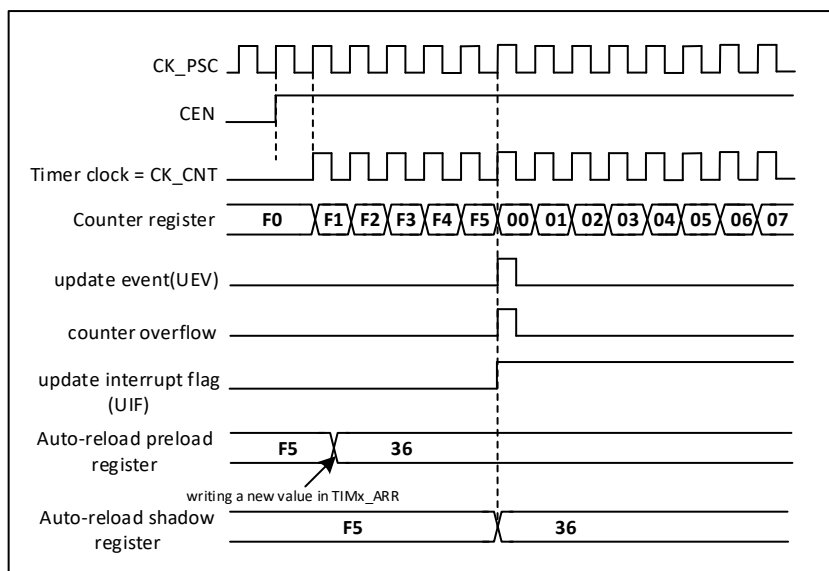
图 18-9 计数器时序图，ARPE=1 时更新事件（TIM1_ARR 预装载）
