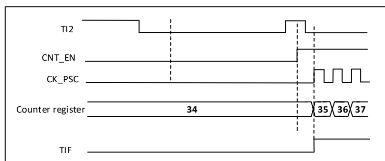
图 18-39 触发模式下的控制电路
