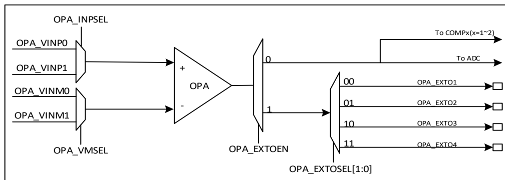
图 15-1 OPA 框图
