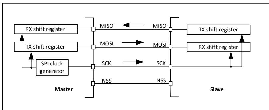
图 33-2 全双工单主/从机应用
