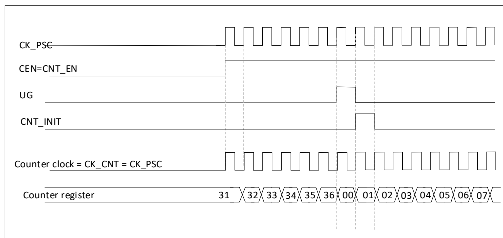
图 17-23 正常模式下的控制电路，内部时钟 1 分频
