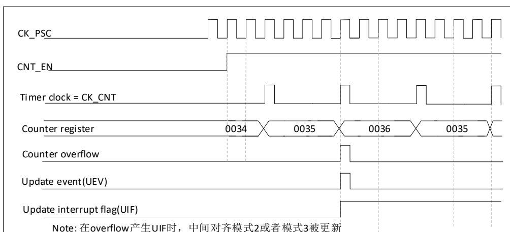
图 17-17 计数器时序图, 内部时钟 4 分频, TIM1_ARR=0x36
