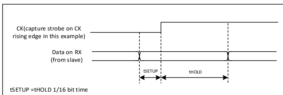
图 30-12RX 数据采样/保持时间
