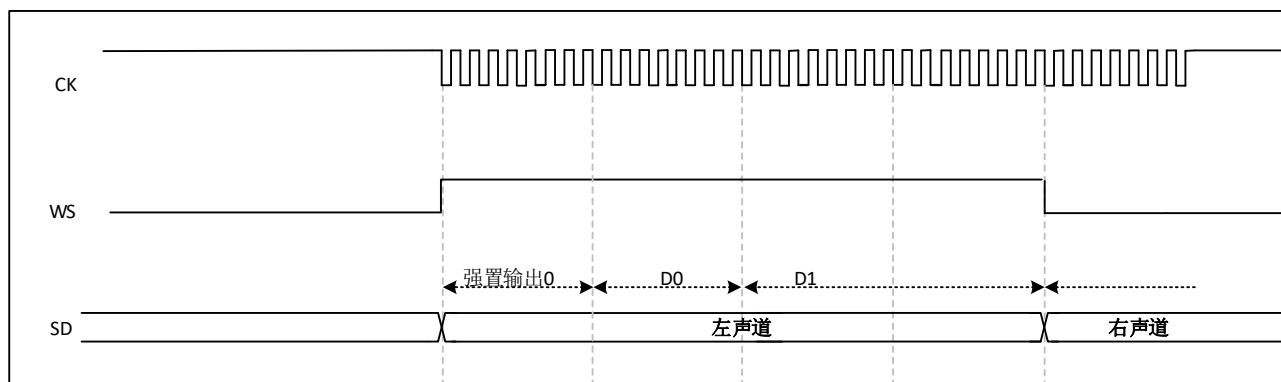
图 33-22 I2S MSB 对齐标准(16 位扩展到 32 位, CKPOL=1)
