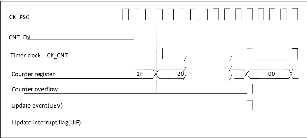
图 21-7 计数器时序图，内部时钟 N 分频
