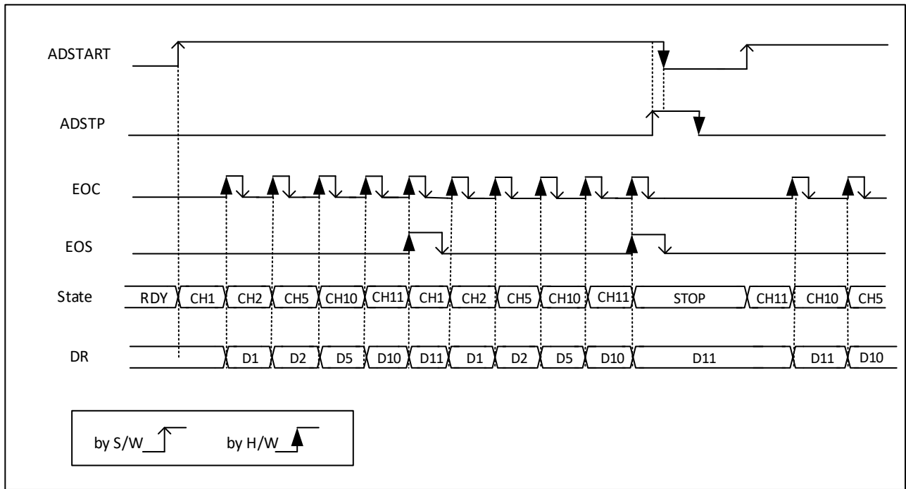
图 12-10 规则连续模式, 软件触发
