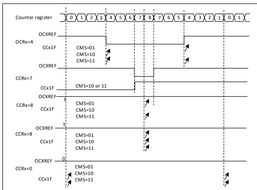
图 18-32 中心对齐模式波形(ARR=8)
