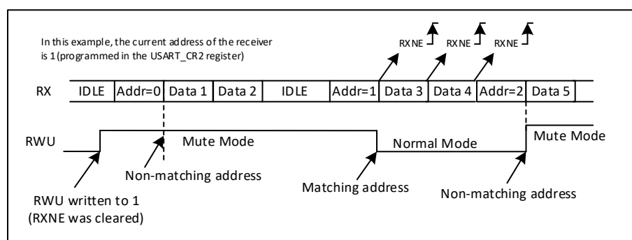
图 30-8 使用地址标志检测的静默模式
