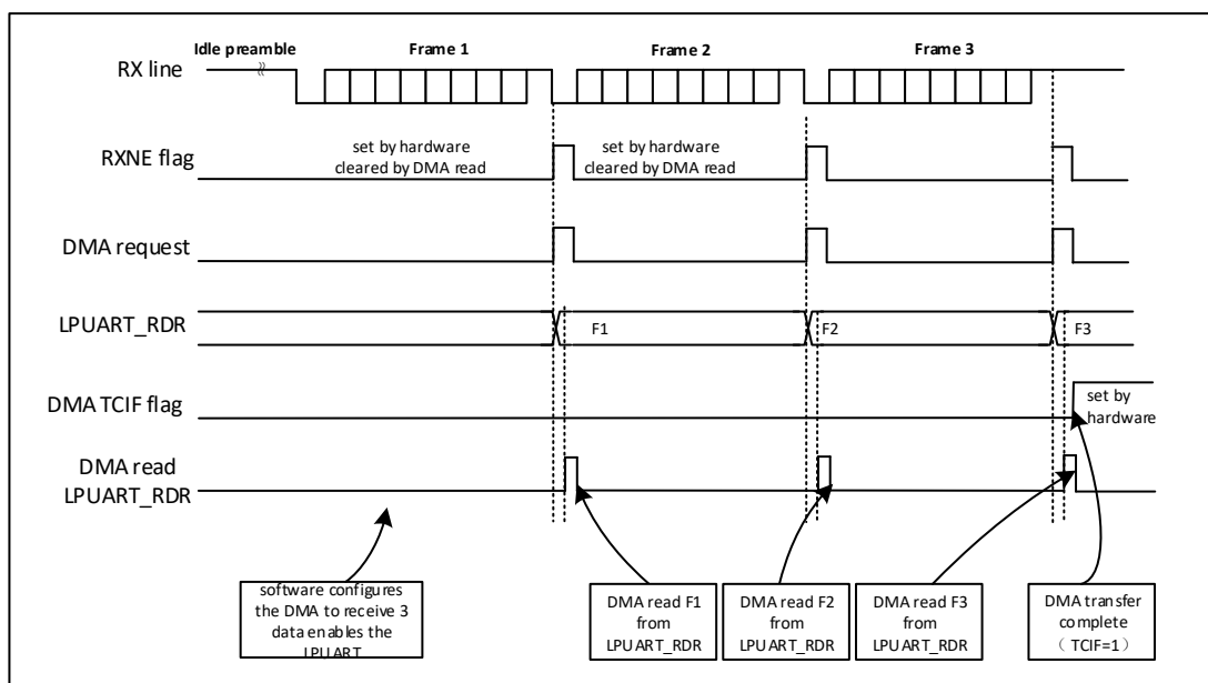
图 32-7 LPUART 用 DMA 接收
