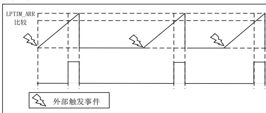
图 24-2 LPTIM 输出, 单次计数模式
