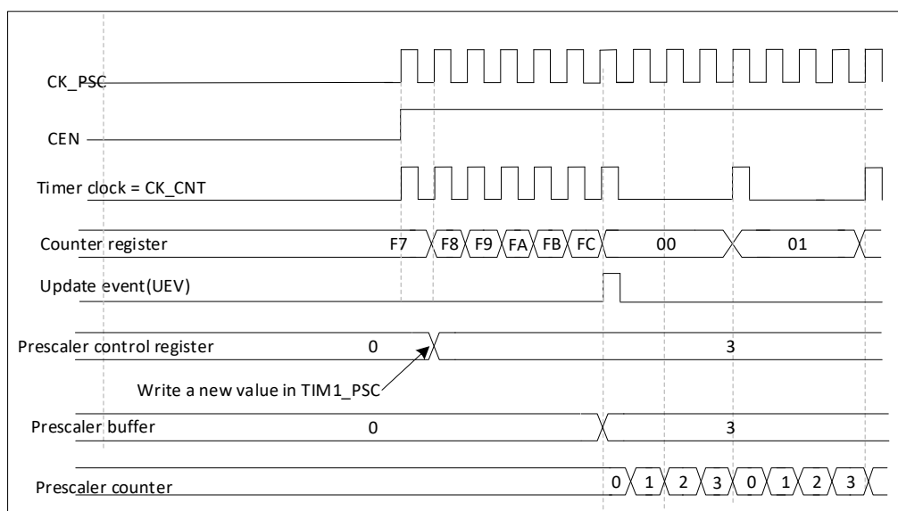
图 19-3 预分频器分频由 1 变为 4 时的计数器时序图
