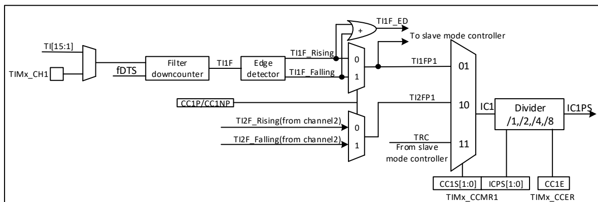
图 20-12 捕获/比较通道(示例:通道 1 输入阶段)
