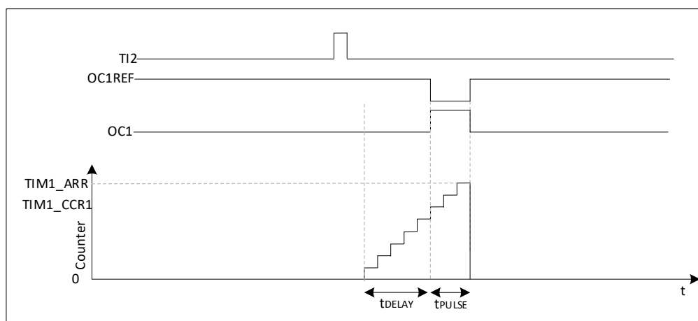
图 17-43 单脉冲模式示例
