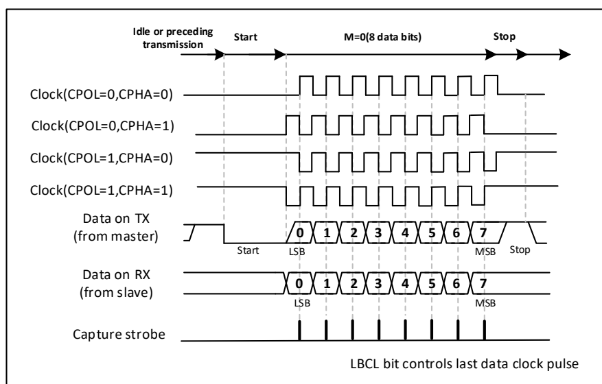
图 30-10 USART 数据时钟序时序图(M=0)
