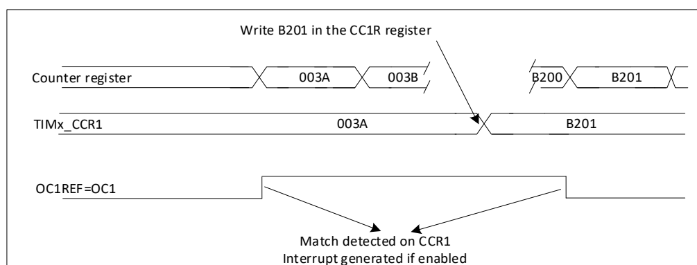
图 17-33 输出比较模式，翻转 OC1
