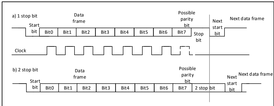
图 30-3 可配置的停止位
