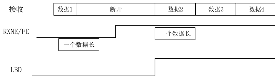
图 30-20 LIN 模式下的断开检测与帧错误的检测
