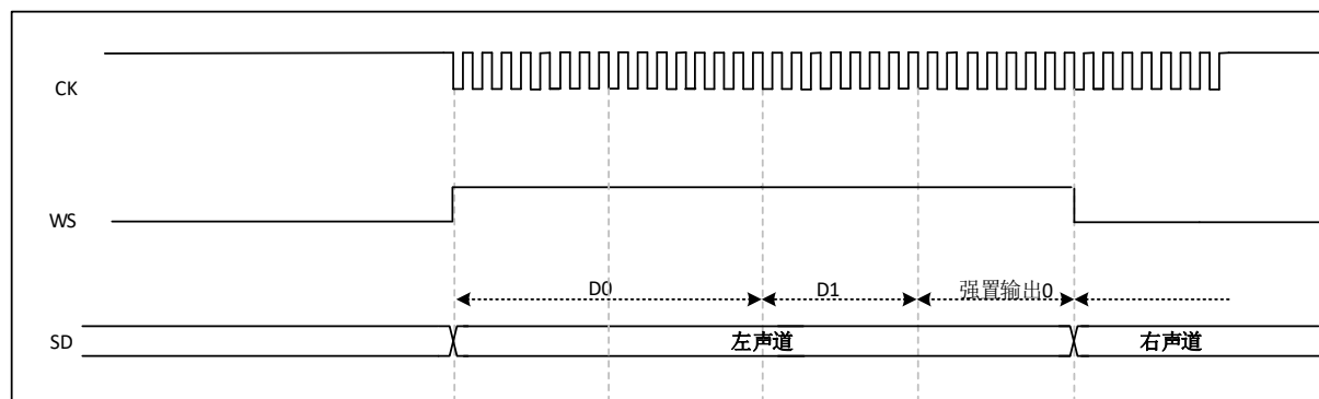
图 33-20 I2S MSB 对齐标准(24 位帧, CKPOL=1)
