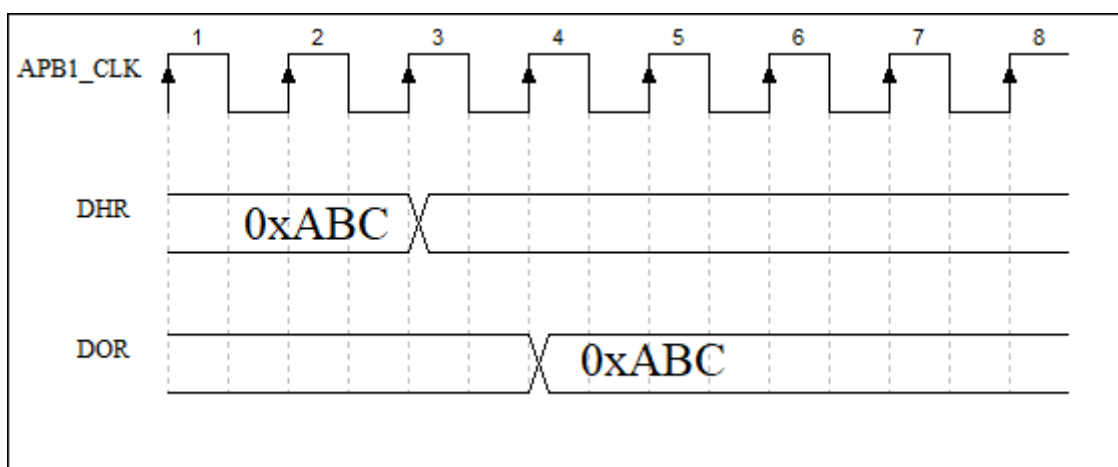
图 13-3 TEN=0 时转换的时间框图
