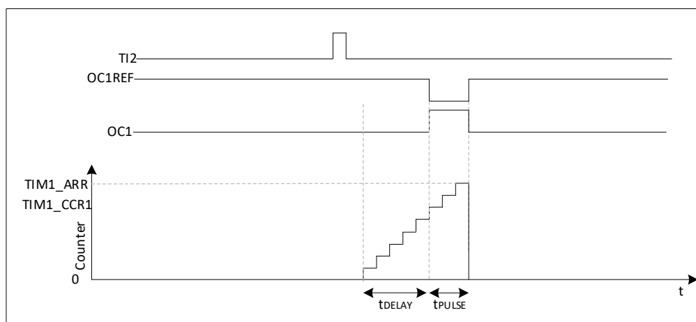
图 19-27 单脉冲模式示例
