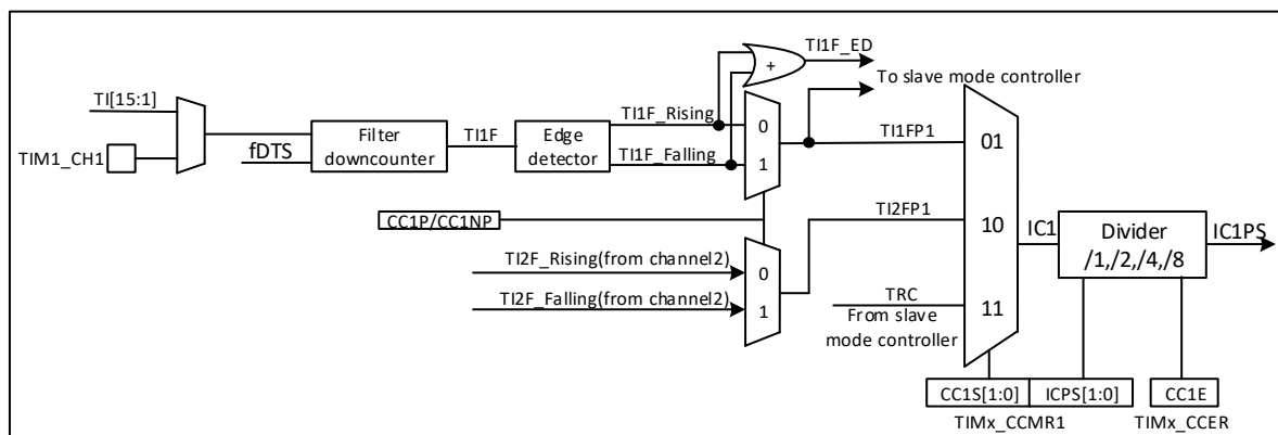
图 17-28 捕获/比较通道(示例：通道 1 输入阶段)
