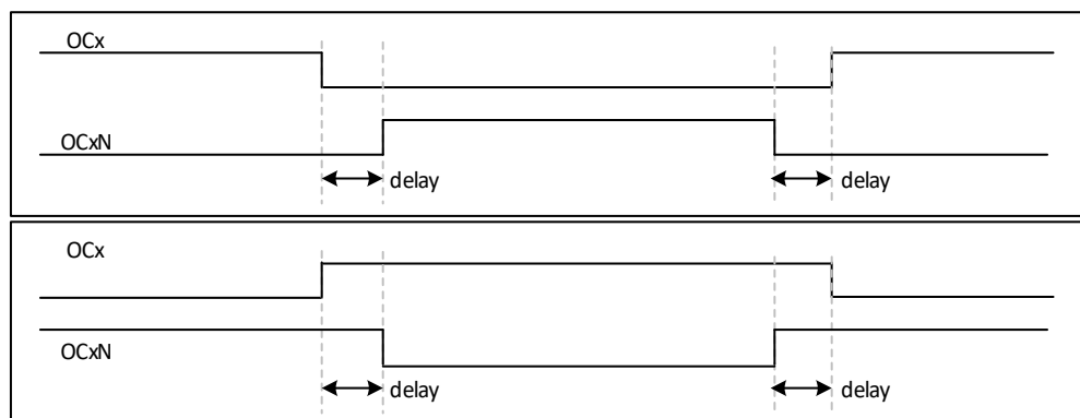
图 22-3 带死区插入的互补输出
