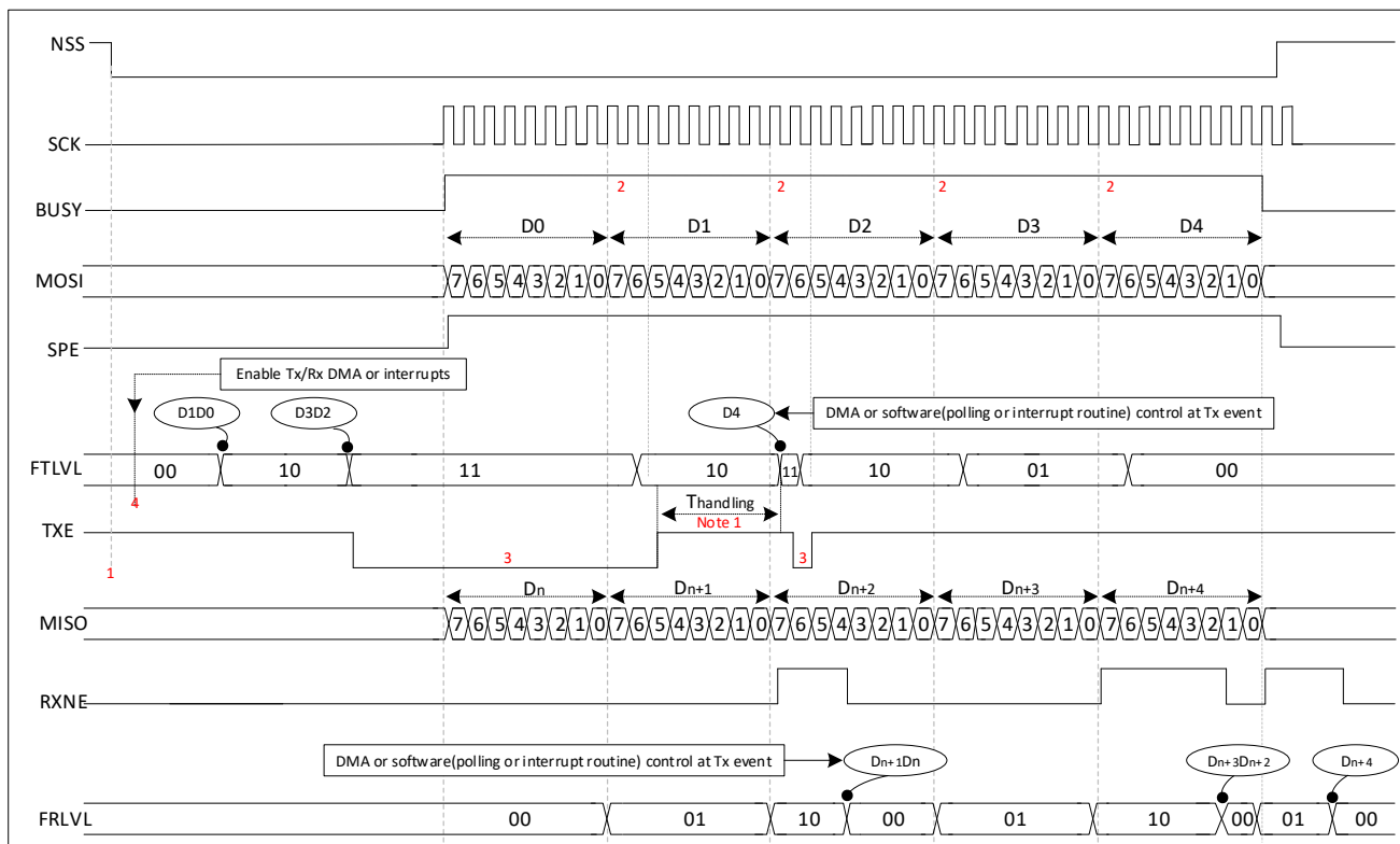
图 33-9 主模式全双工通讯(帧长=8)
