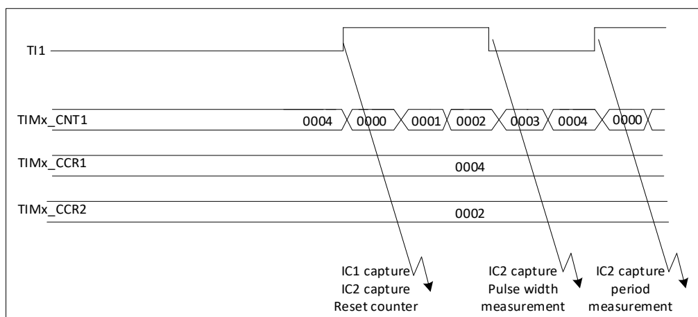
图 17-32 PWM 输入模式时序
