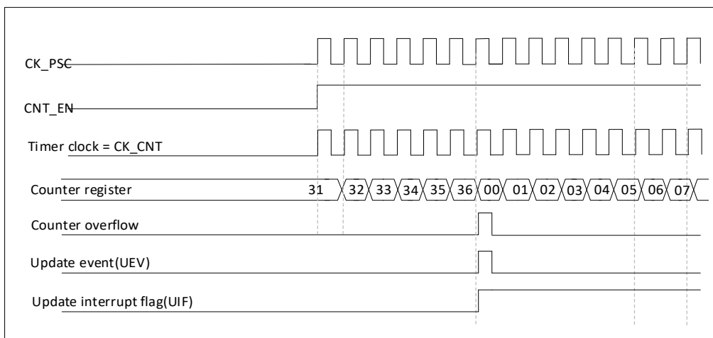
图 17-4 计数器时序图，内部时钟 1 分频
