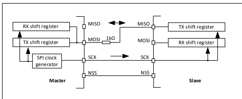
图 33-3 半双工单主/从机应用
