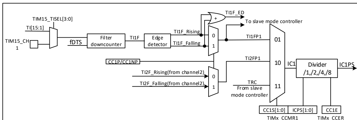
图 19-16 捕获/比较通道(示例:通道 1 输入阶段)
