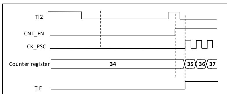
图 19-30 触发模式下的控制电路
