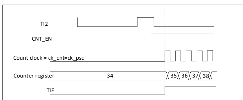
图 17-50 触发模式下的控制电路
