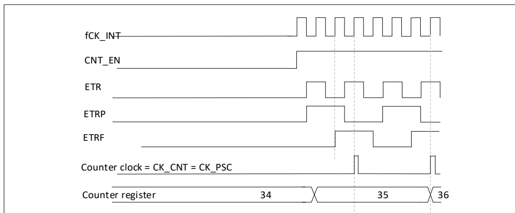
图 17-27 外部时钟模式 2 控制电路时序
