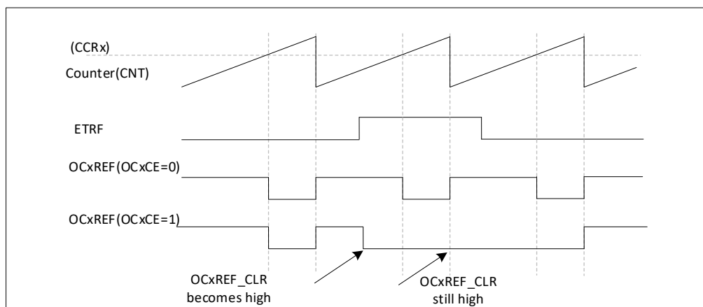
图 18-33 清除 TIMx 的 OCxREF
