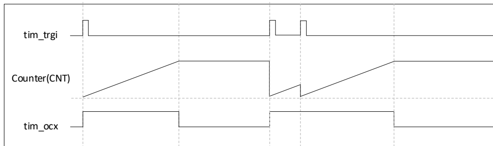
图 17-44 可再触发单脉冲模式
