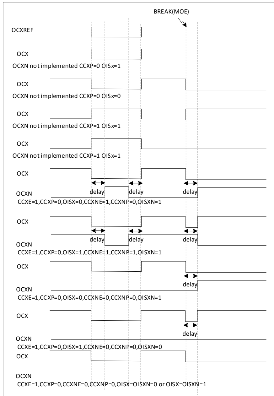
图 20-20 响应刹车事件的不同输出行为
