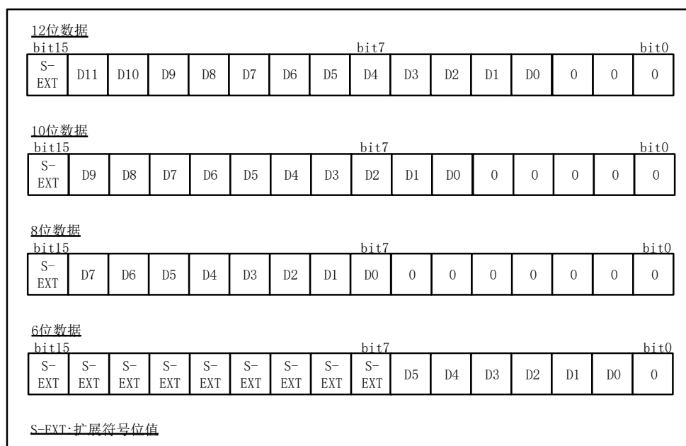
图 12-16 左对齐 (offset 使能, 有符号数)
