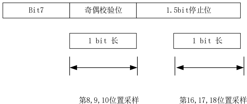
图 30-22 使用 1.5 停止位检测奇偶检验错
