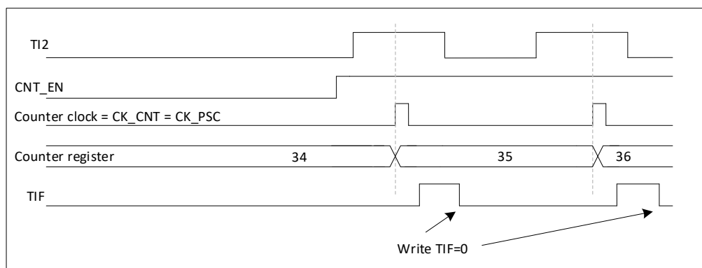
图 17-25 外部时钟模式 1 控制电路时序
