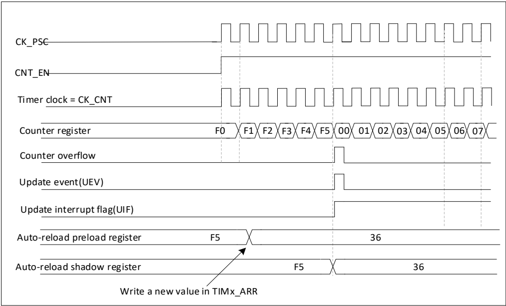
图 19-9 计数器时序图，ARPE=1 时更新事件 (TIM1_ARR 预装载)
