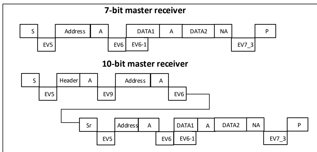
图 29-7 方法 2: 主机接收时的传输时序 N=2
