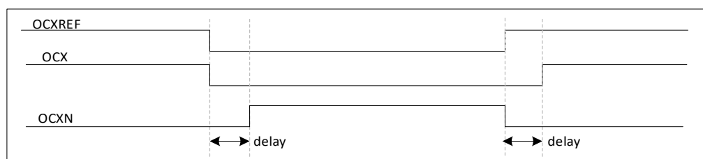
图 19-22 带死区插入的互补输出
