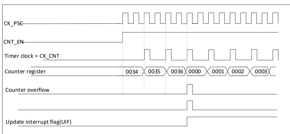
图 20-5 计数器时序图, 内部时钟 2 分频
