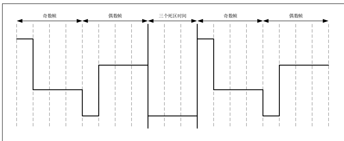
图 16-2 typeA 下的 CDRV[0]的波形
