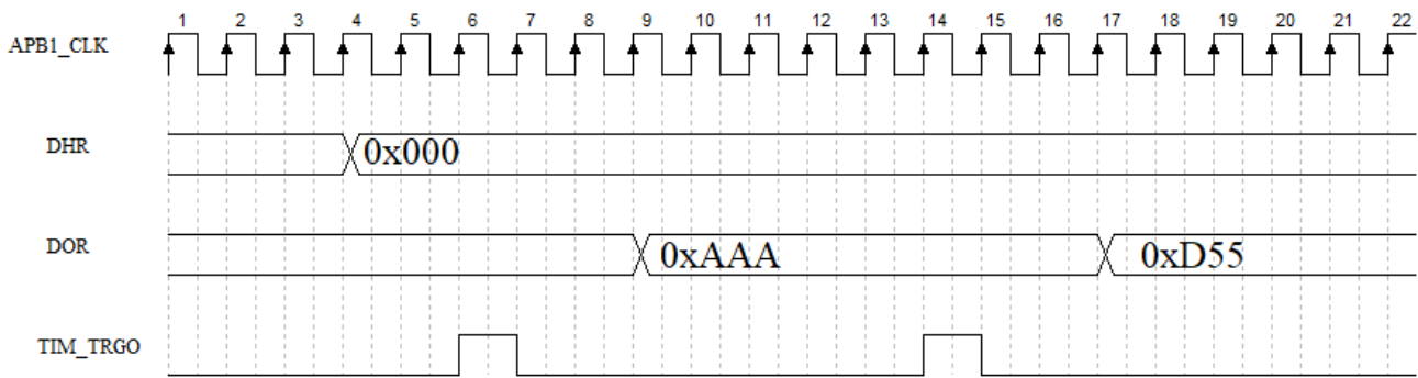
图 13-6 带 LFSR 波形生成的 DAC 转换(使能硬件触发)
