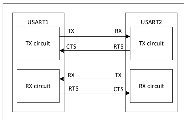
图 30-15 USART 间的硬件流控制
