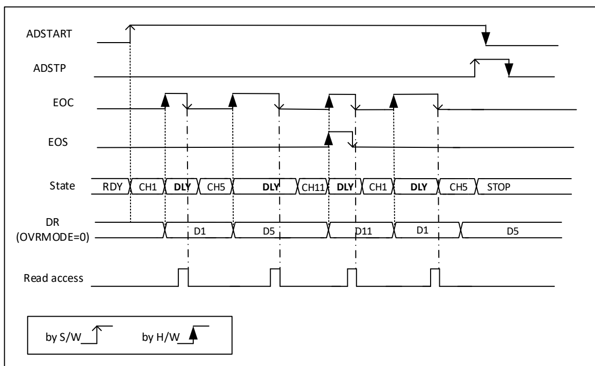
图 12-19 AUTODLY 模式
