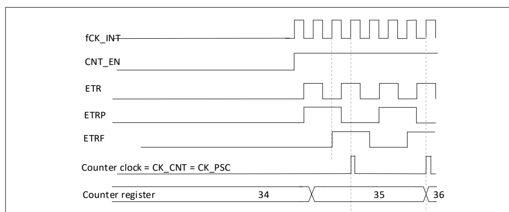
图 19-15 外部时钟模式 2 时序
