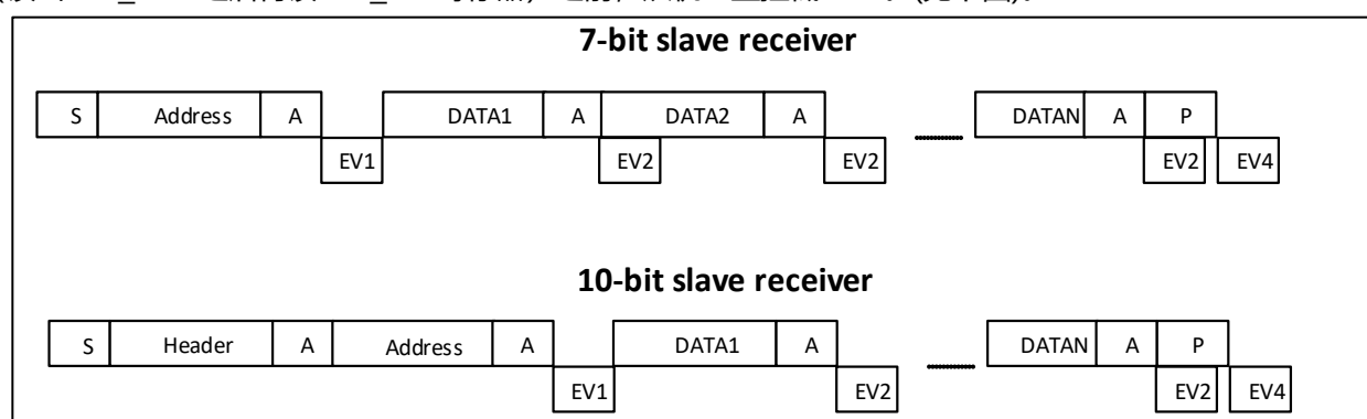
图 29-3 从机接收序列图
