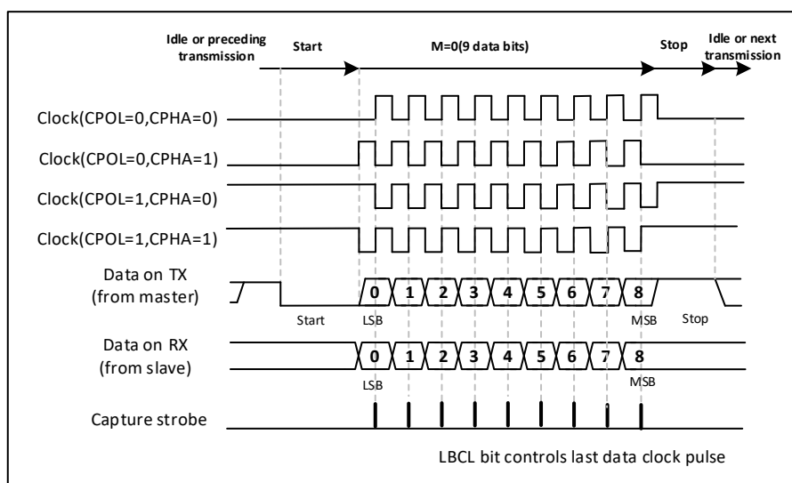
图 30-11 USART 数据时钟序时序图(M=1)
