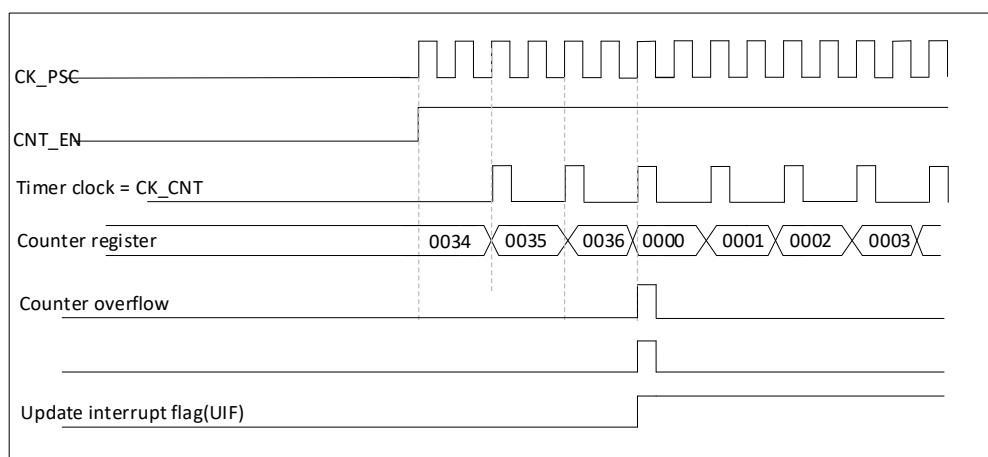
图 19-5 计数器时序图, 内部时钟 2 分频
