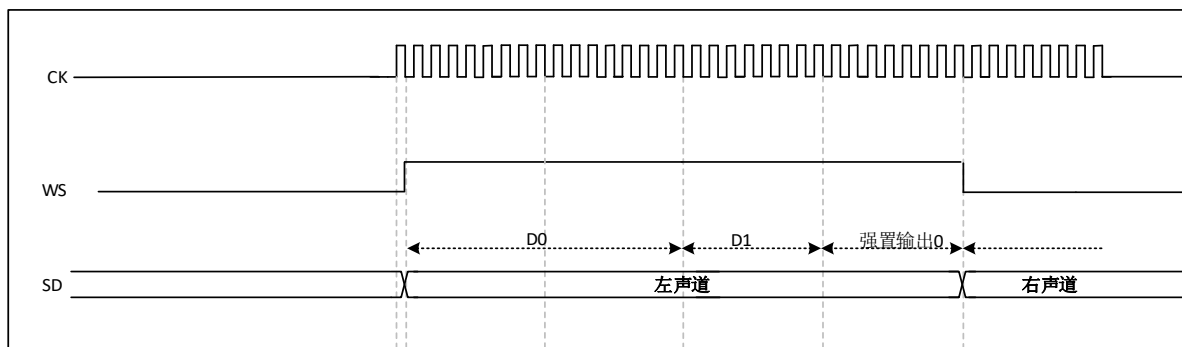
图 33-19 I2S MSB MSB 对齐标准(24 位帧, CKPOL=0)
