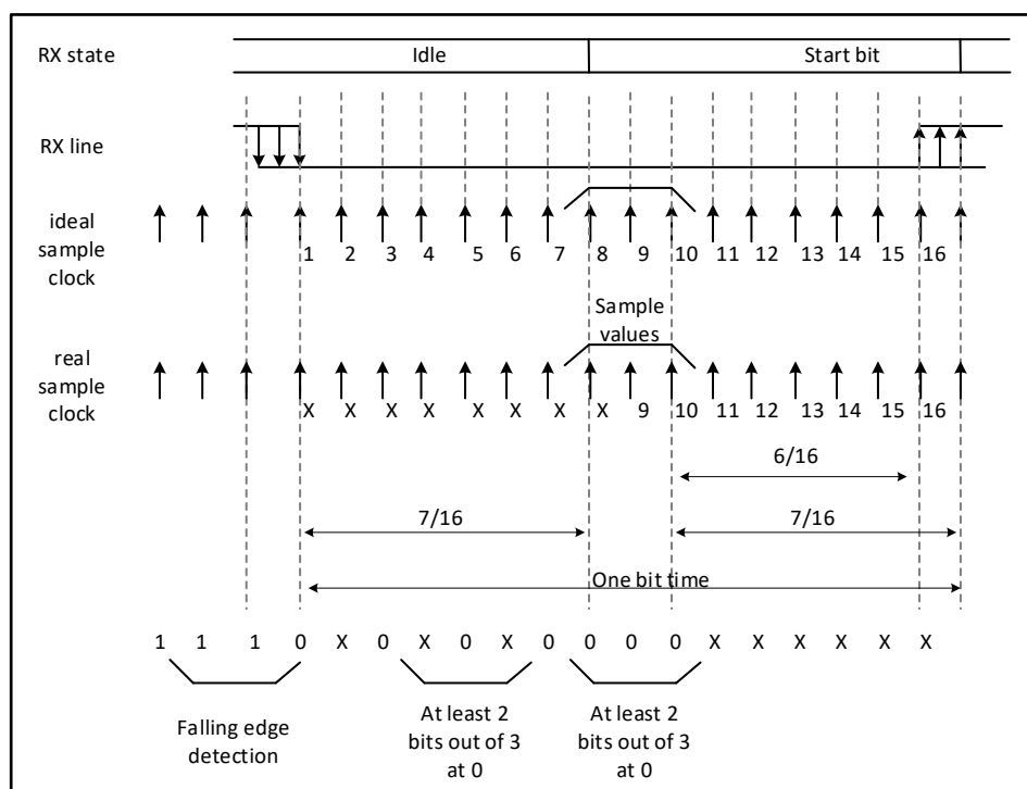
图 30-5 起始位检测
