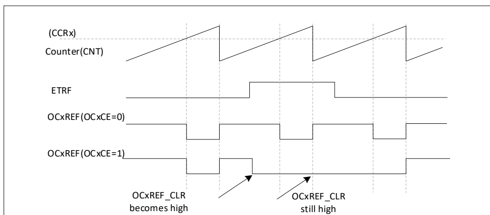
图 17-41 清除 TIM1 的 OCxREF
