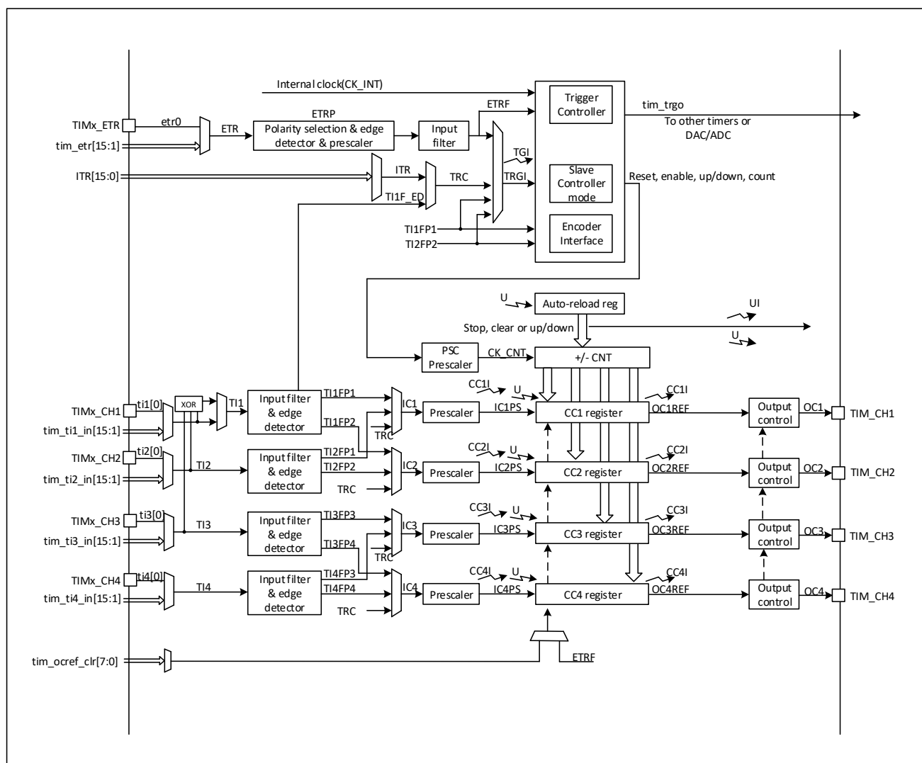
图 18-1 通用框图 (TIM2)
