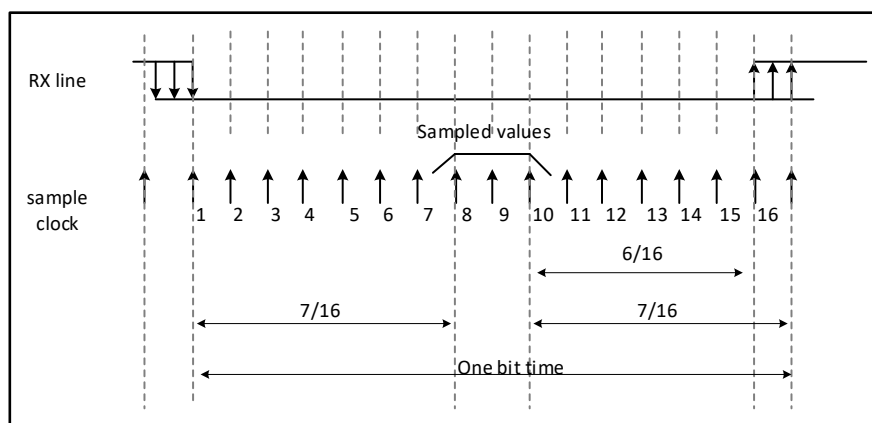
图 30-6 噪声检测时数据采样
