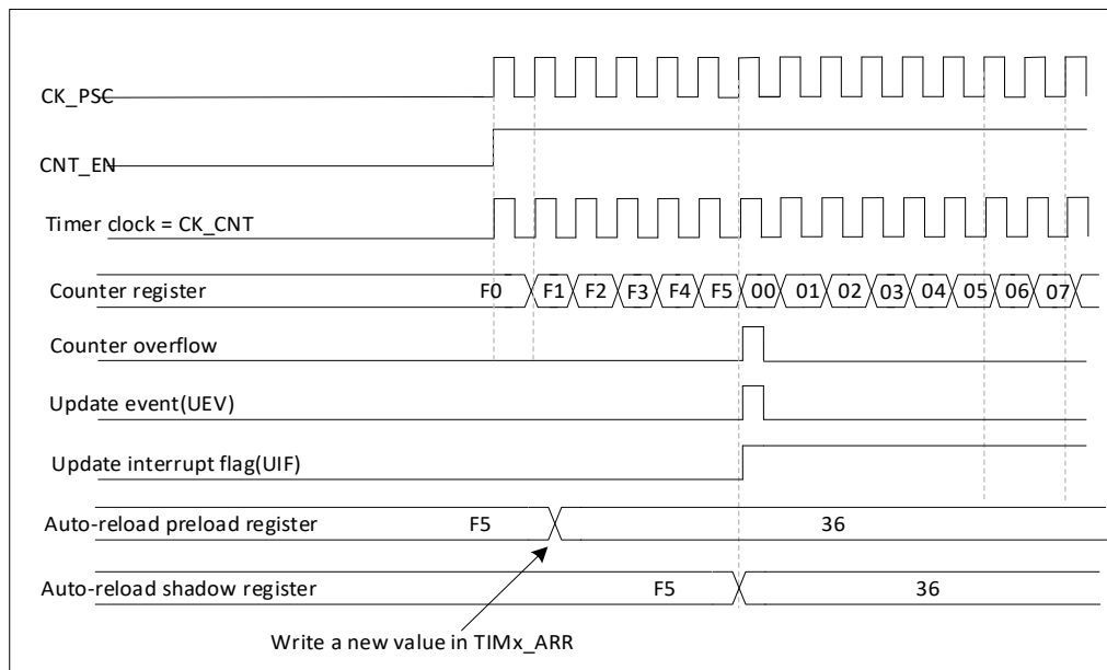
图 21-9 计数器时序图, ARPE=1 时的更新事件(TIMx_ARR 预装载)
