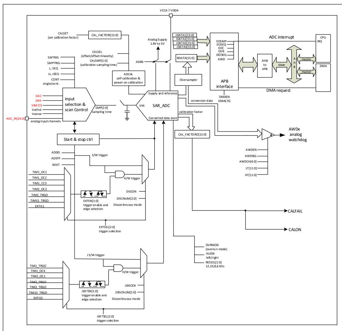
图 12-1 ADC 框图
