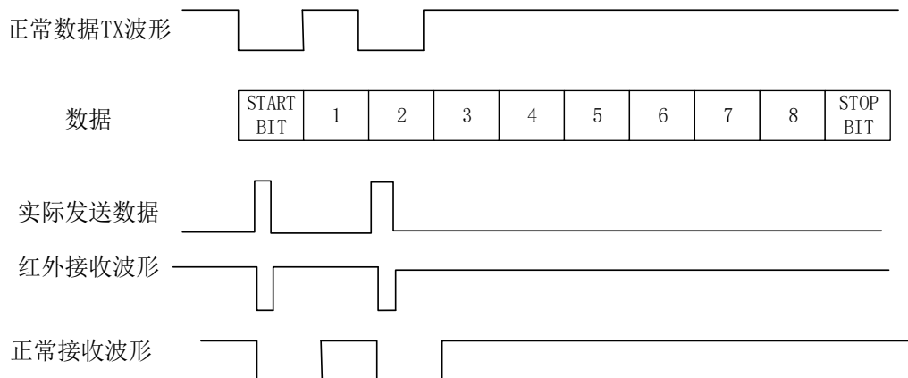
图 30-24 IrDA 数据调制 (3/16) — 普通模式
