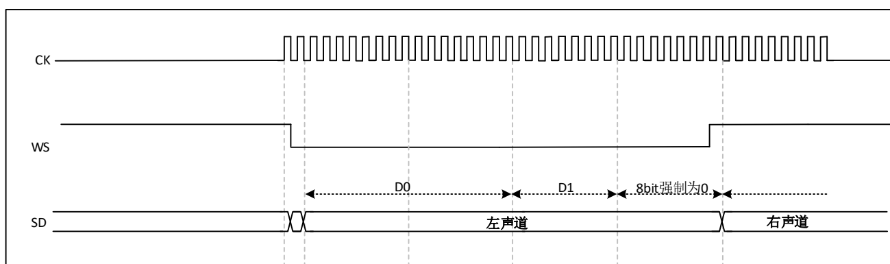
图 33-14 I2S 飞利浦协议波形(24 位帧, CKPOL=0)
