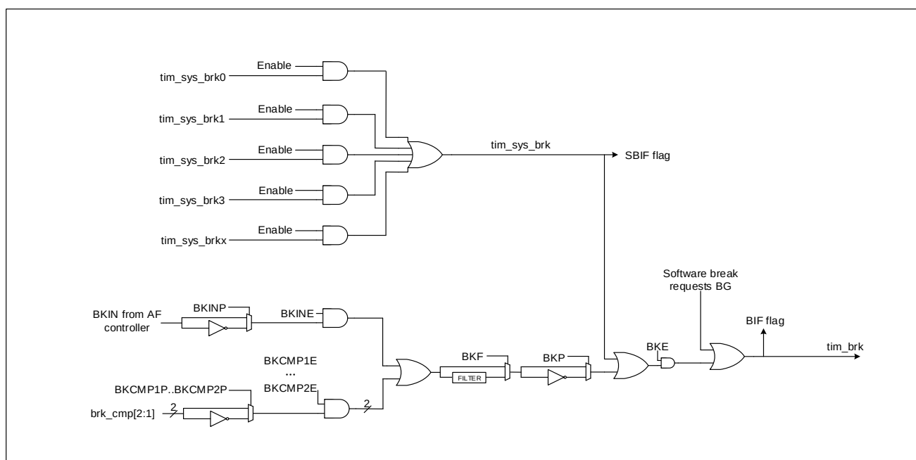
图 17-39 刹车电路图
