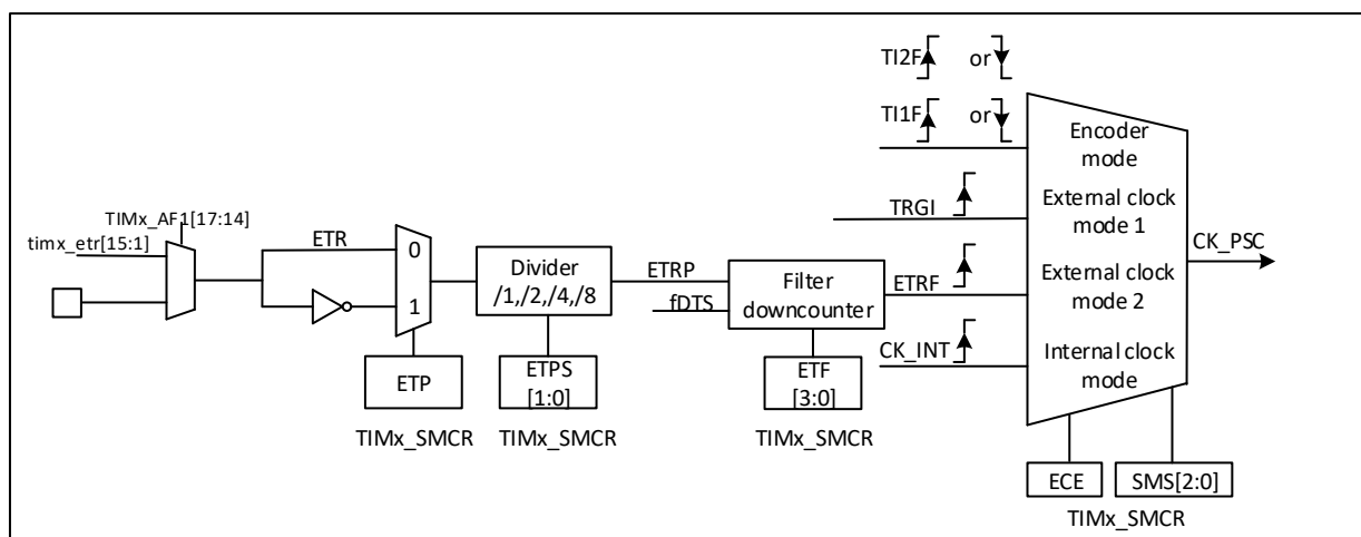
图 18-24 外部触发输入模块
