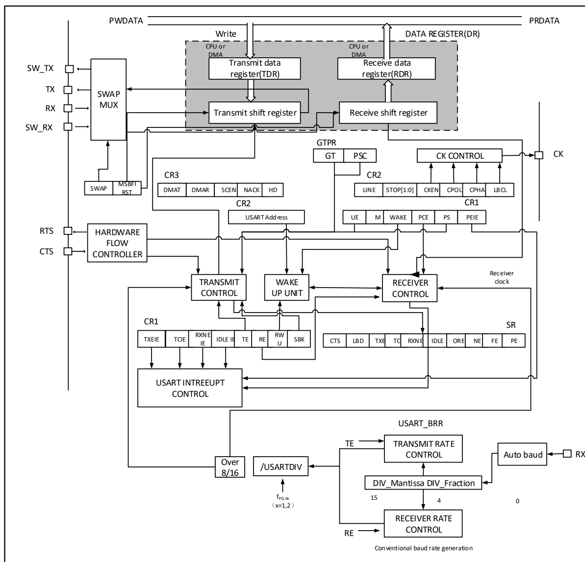
图 30-1 USART 框图
