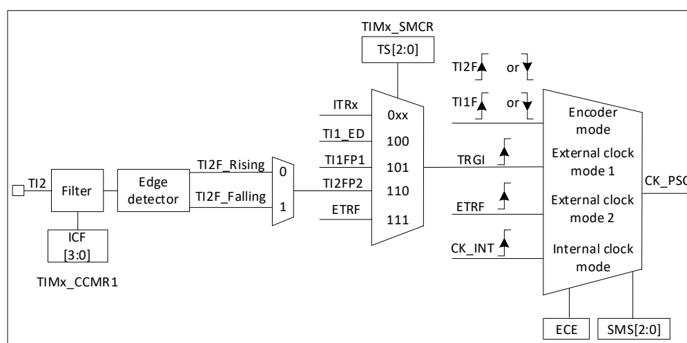
图 17-24 TI2 外部时钟连接示例
