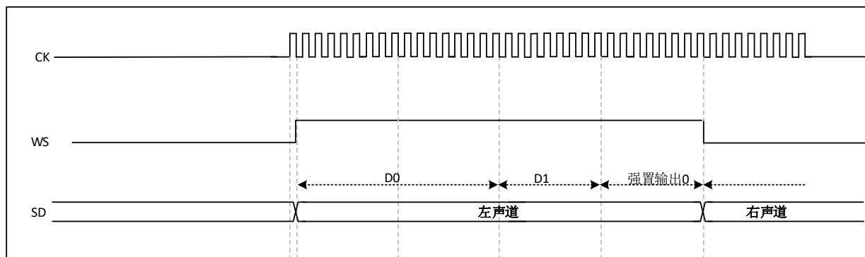
图 33-21 I2S MSB 对齐标准(16 位扩展到 32 位, CKPOL=0)
