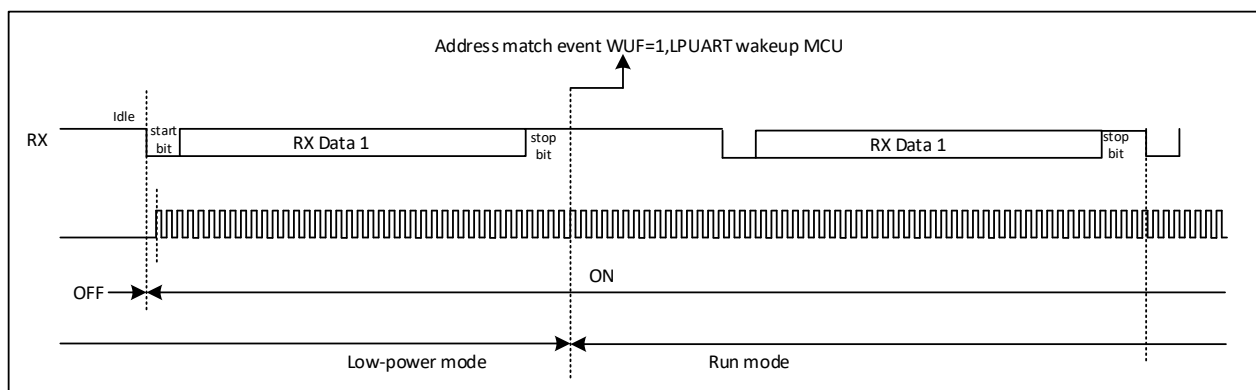
图 32-11 LPUART 地址匹配唤醒
