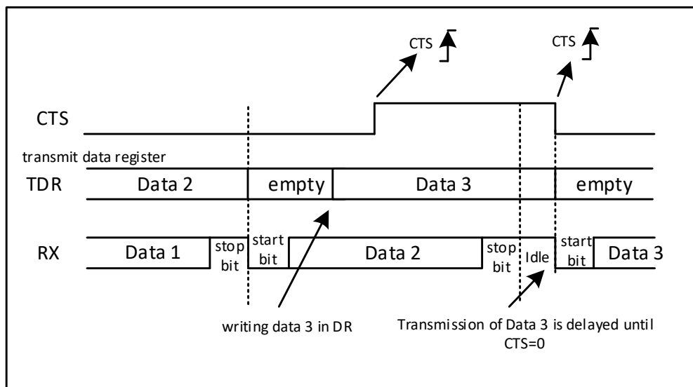
图 30-17 CTS 流控制
