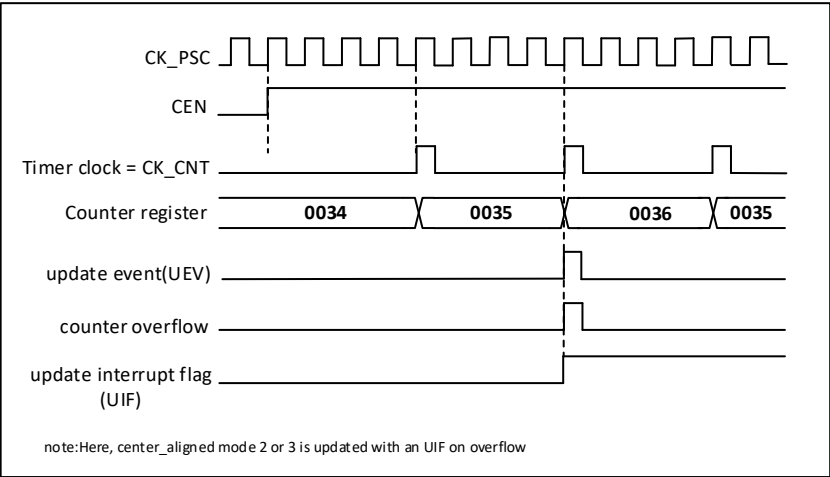
图 18-17 计数器时序图，内部时钟 4 分频, TIM1_ARR=0x36
