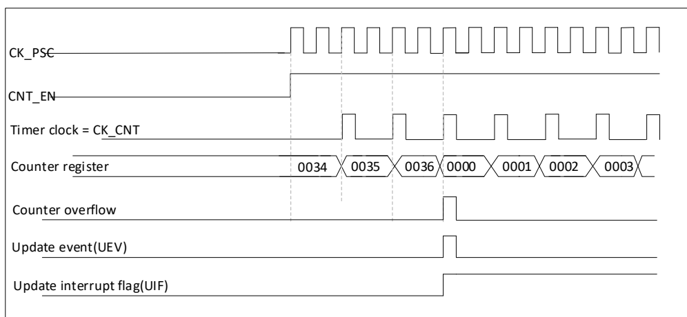
图 17-5 计数器时序图，内部时钟 2 分频
