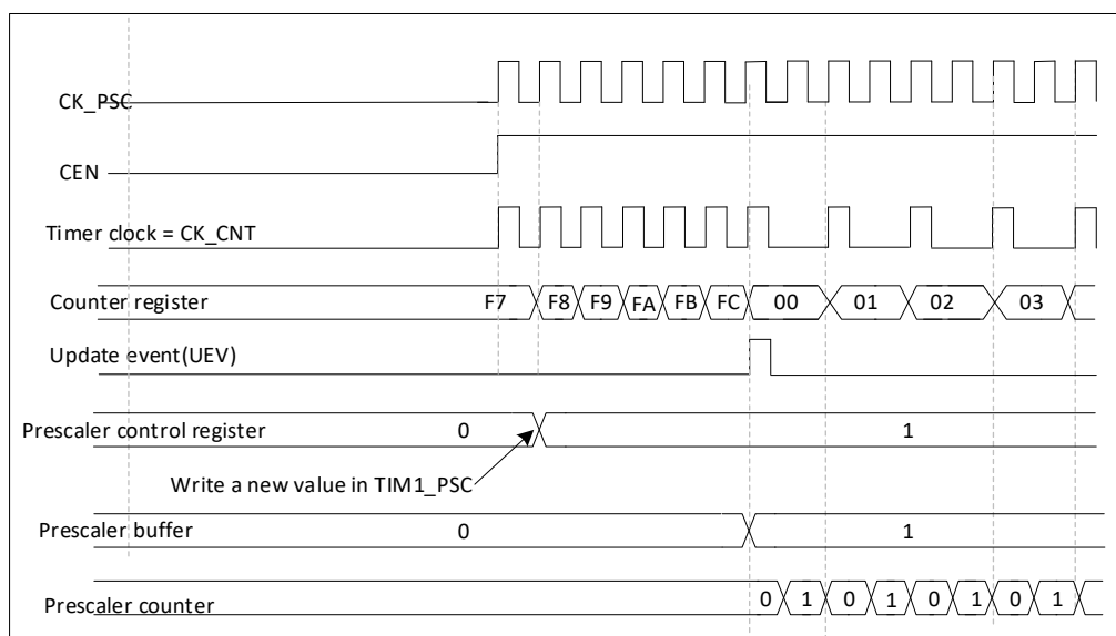
图 19-2 预分频器分频由 1 变为 2 时的计数器时序图
