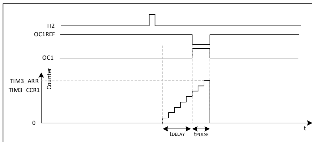
图 18-34 单脉冲模式示例
