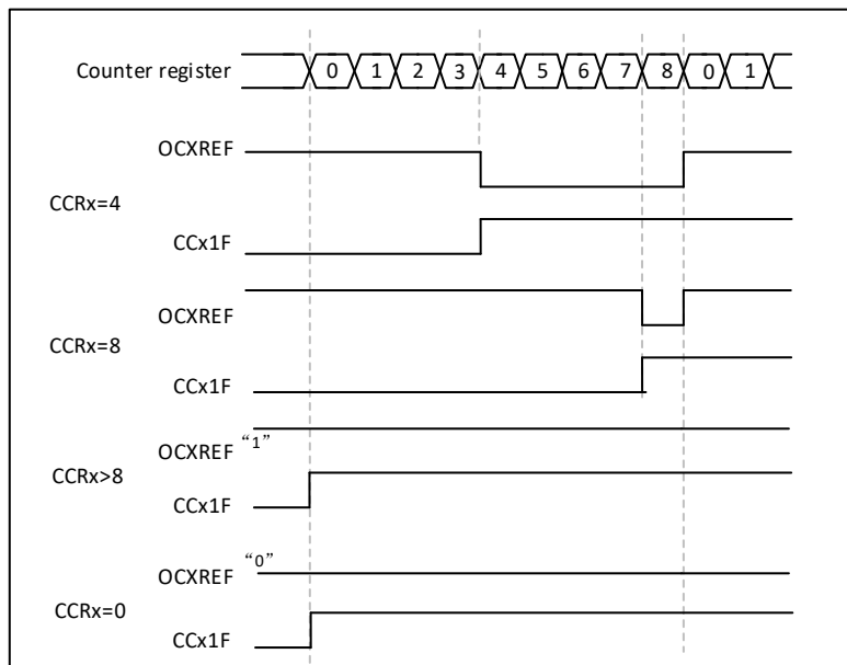
图 18-31 边沿对齐方式 PWM 输出波形 (ARR=8)
