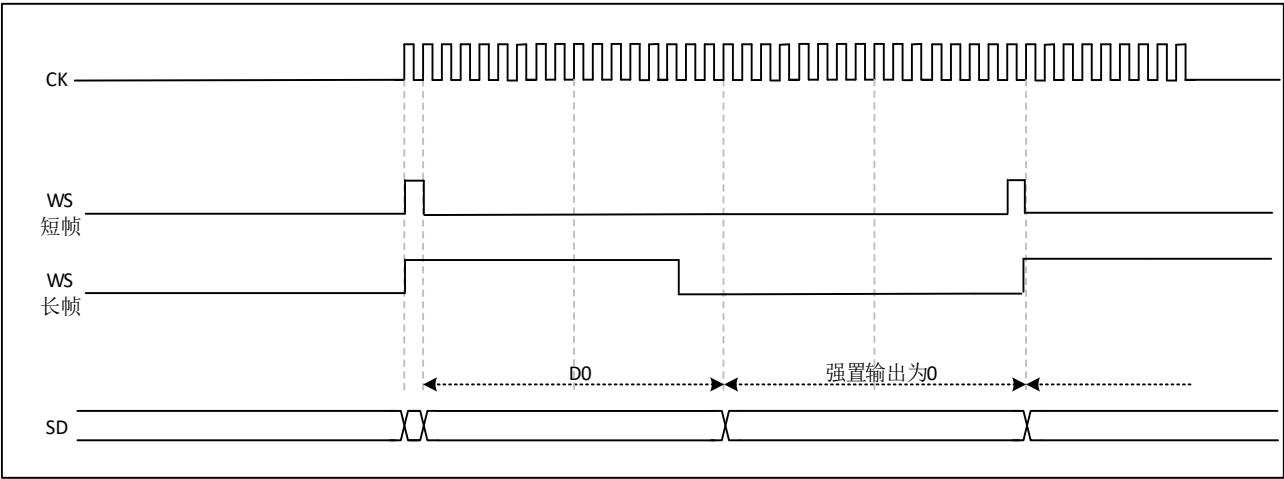
图 33-31I2S PCM 标准(16 位扩展到 32 位, CKPOL=0)
