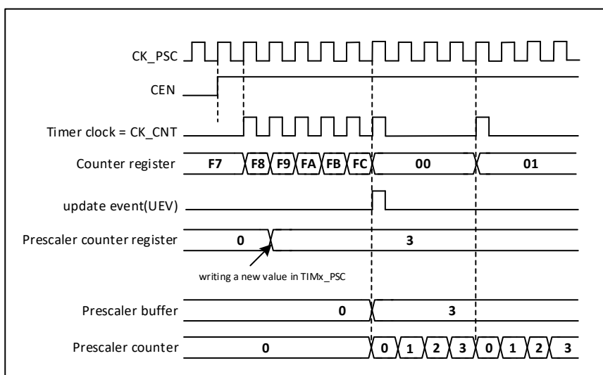
图 18-3 预分频器分频由 1 变为 4 时的计数器时序图
