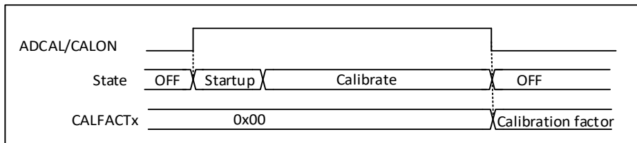
图 12-2 ADC 校准
