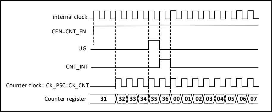
图 18-21 正常模式下的控制电路，内部时钟 1 分频
