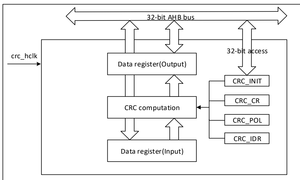
图 11-1 CRC calculation unit 框图
