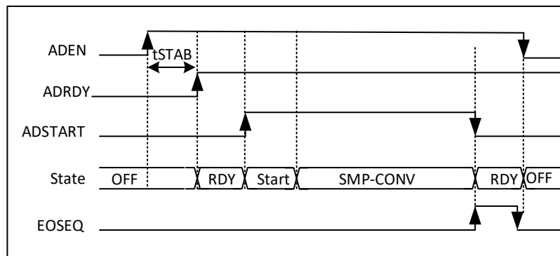
图 12-3 使能/禁止 ADC
