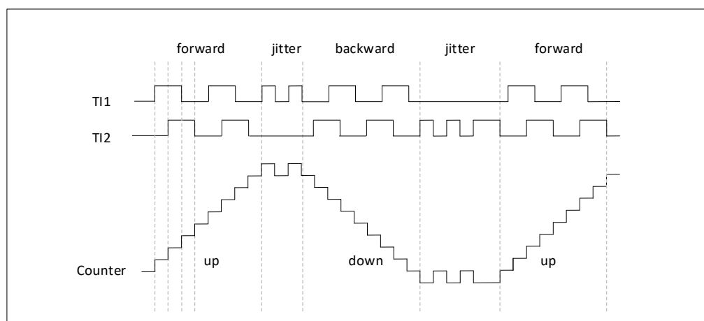
图 17-45 编码器接口模式下的计数器工作示例
