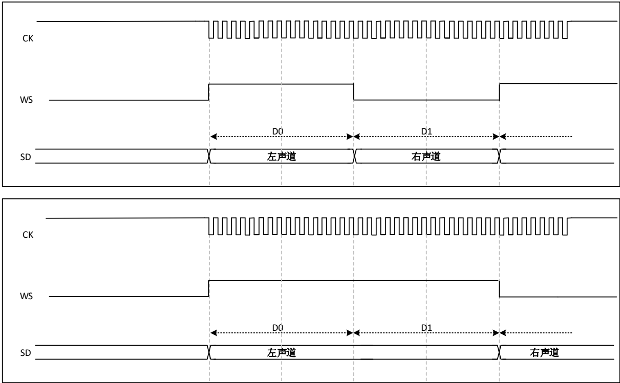
图 33-24 I2S LSB 对齐标准 (16/32 位全精度, CKPOL=1)
