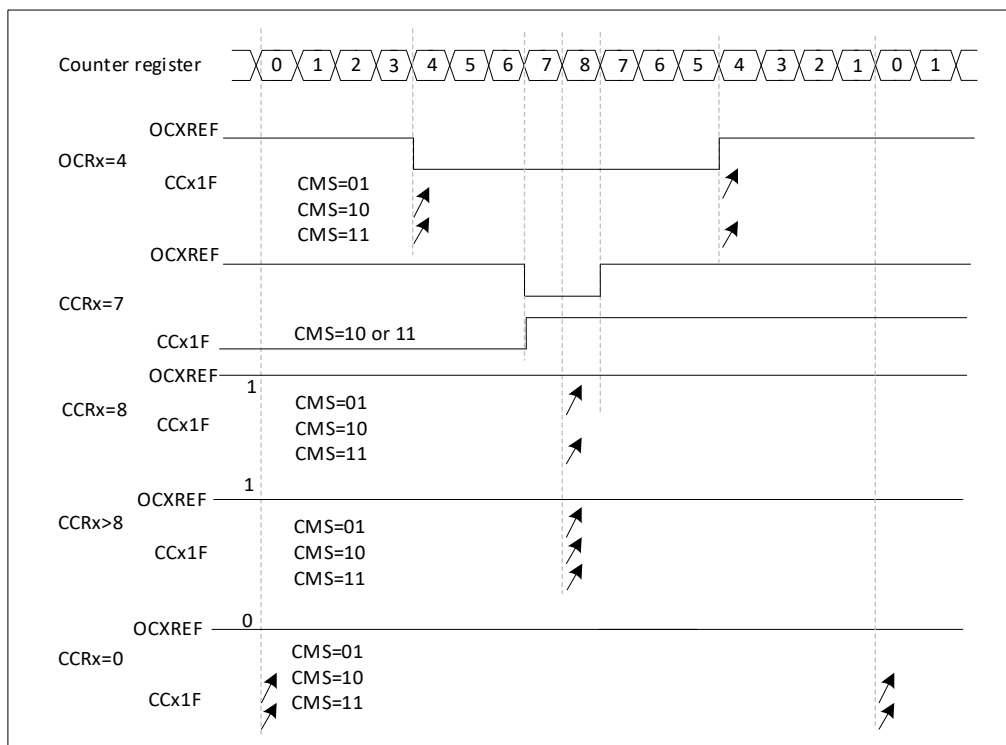
图 17-35 中心对齐模式波形(ARR=8)
