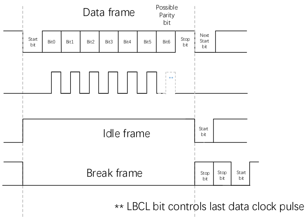
图 32-2 LPUART 字长编程
