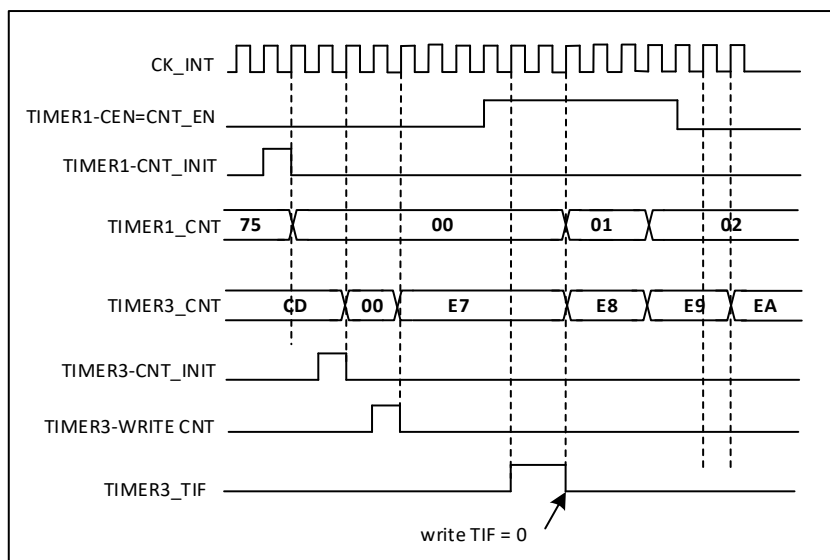
图 18-45 使能 TIM1 启动 TIM3
