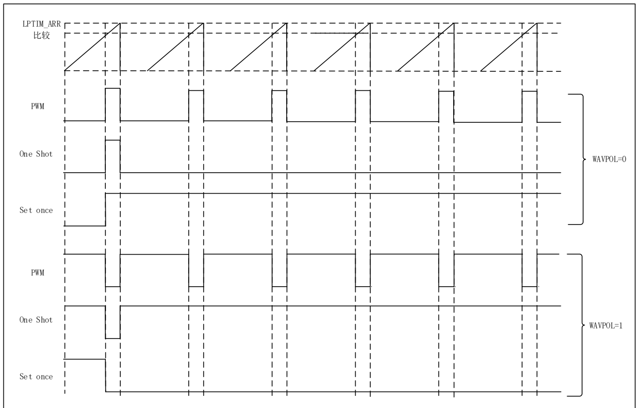
图 24-5 LPTIM 波形产生
