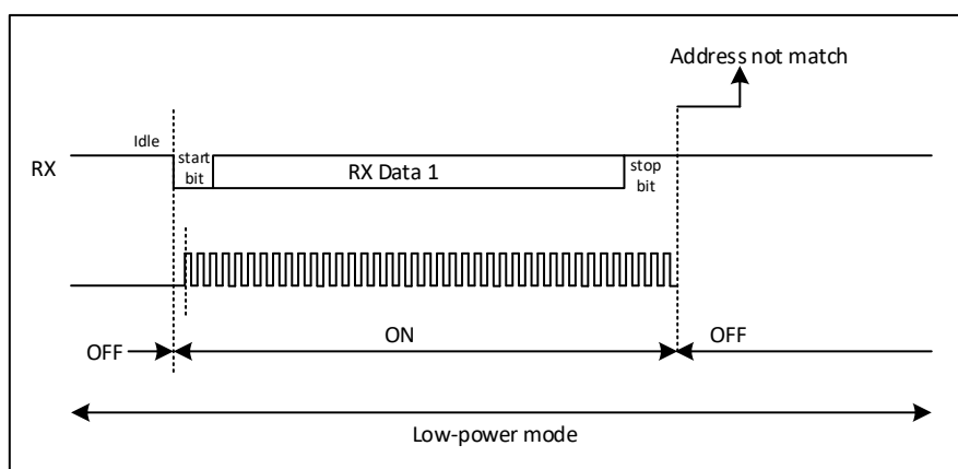
图 32-12 LPUART 地址不匹配无法唤醒
