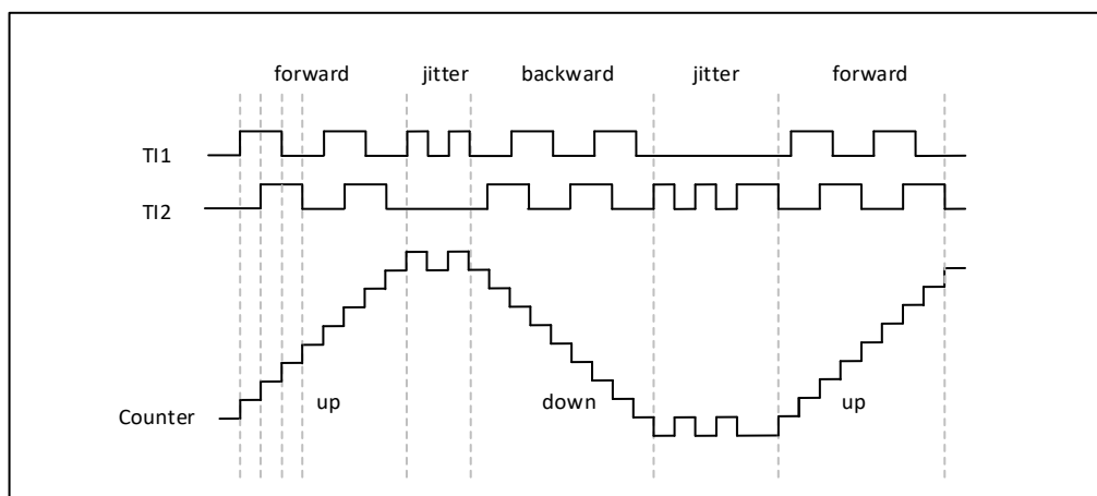
图 18-35 编码器接口模式下的计数器工作示例
