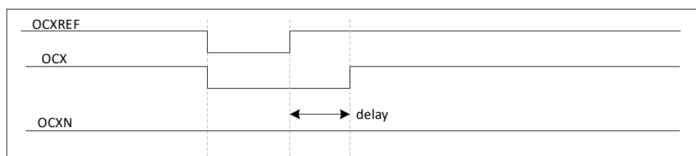
图 17-37 延迟时间大于负脉冲宽度的死区波形
