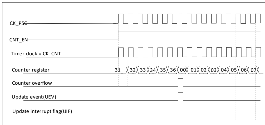
图 19-4 计数器时序图, 内部时钟 1 分频
