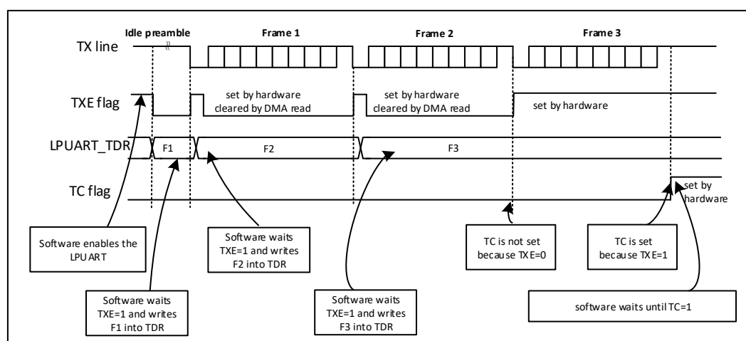
图 32-3 发送时的 TC/TXE 行为
