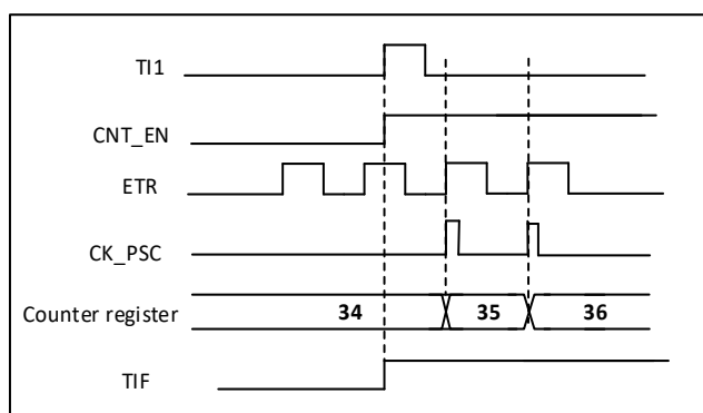
图 18-40 外部时钟模式 2 + 触发模式下的控制电路
