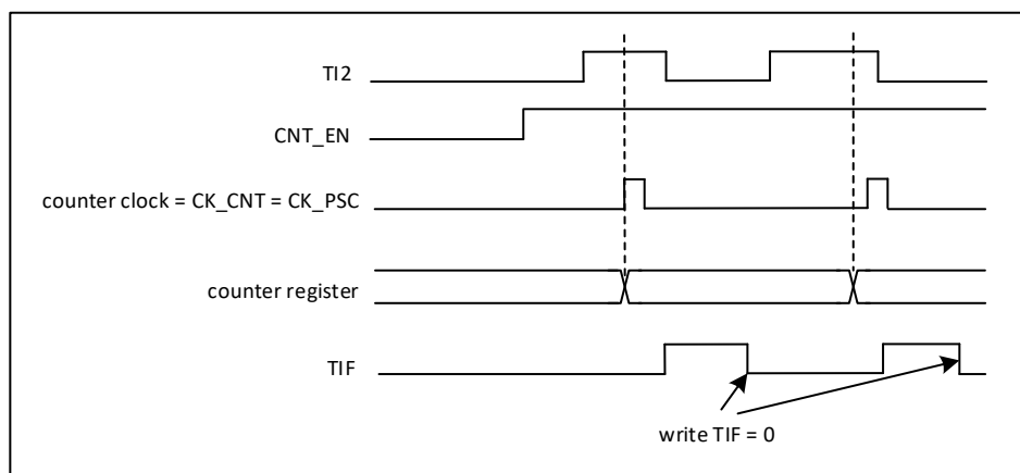
图 18-23 外部时钟模式 1 控制电路时序
