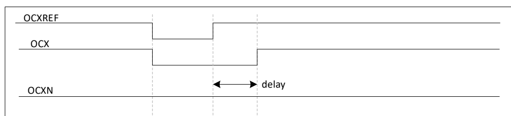
图 20-18 延迟时间大于负脉冲宽度的死区波形
