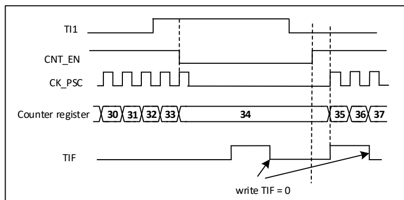
图 18-38 门控模式下的控制电路
