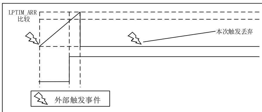
图 24-3 LPTIM 输出,单次计数模式 (WAVE=1)
