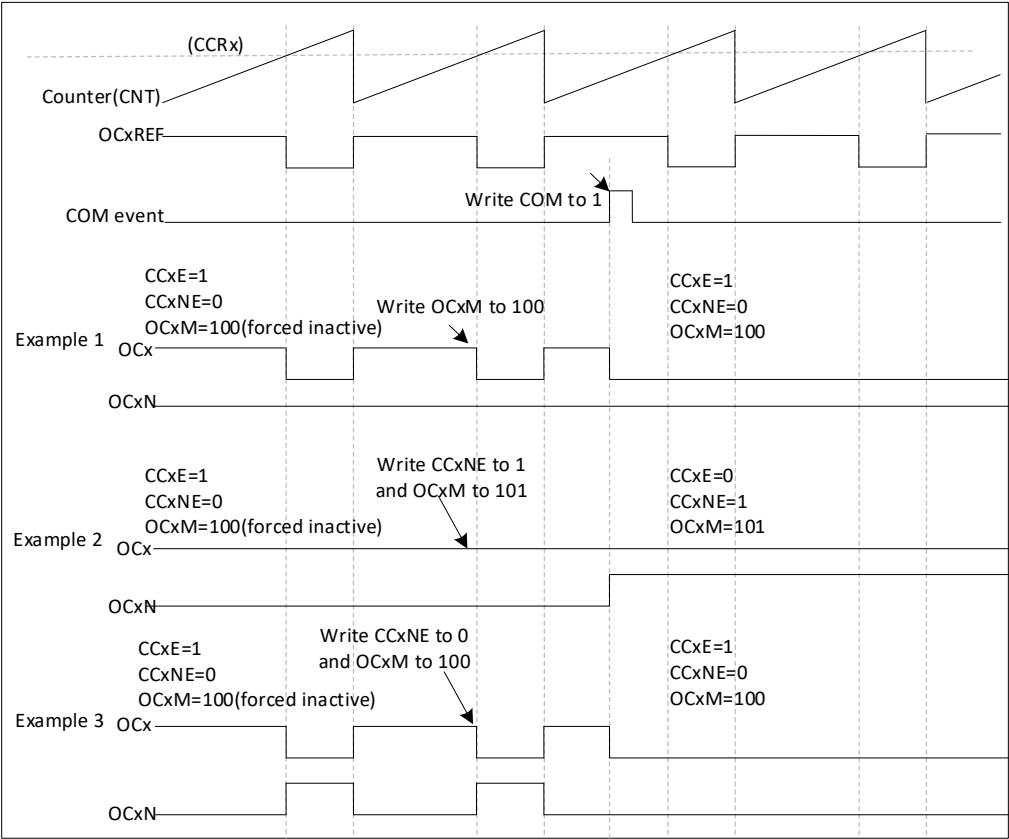
图 17-42 COM 事件生成 6 步 PWM 的示例 (OSSR=1)
