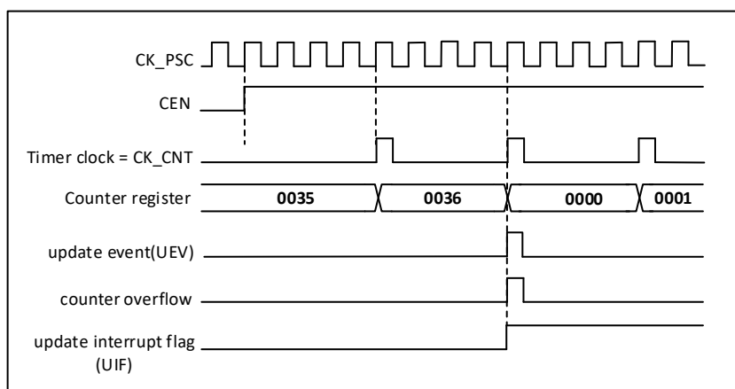
图 18-6 计数器时序图, 内部时钟 4 分频
