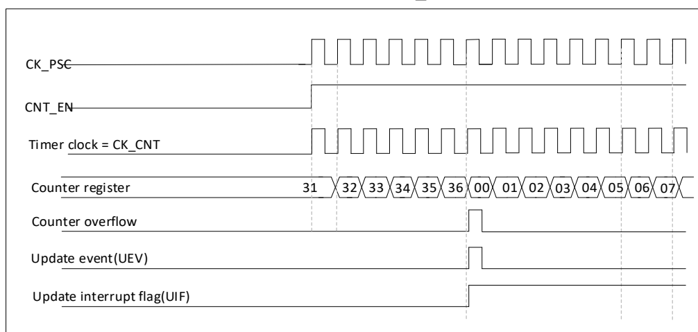
图 20-4 计数器时序图, 内部时钟 1 分频
