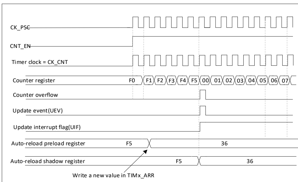
图 17-9 计数器时序图，ARPE=1 时更新事件 (TIM1_ARR 预装载)
