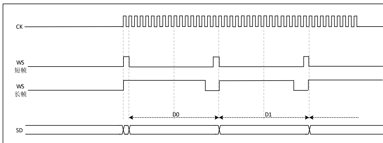
图 33-29 I2S PCM 标准(16 位帧, CKPOL=0)
