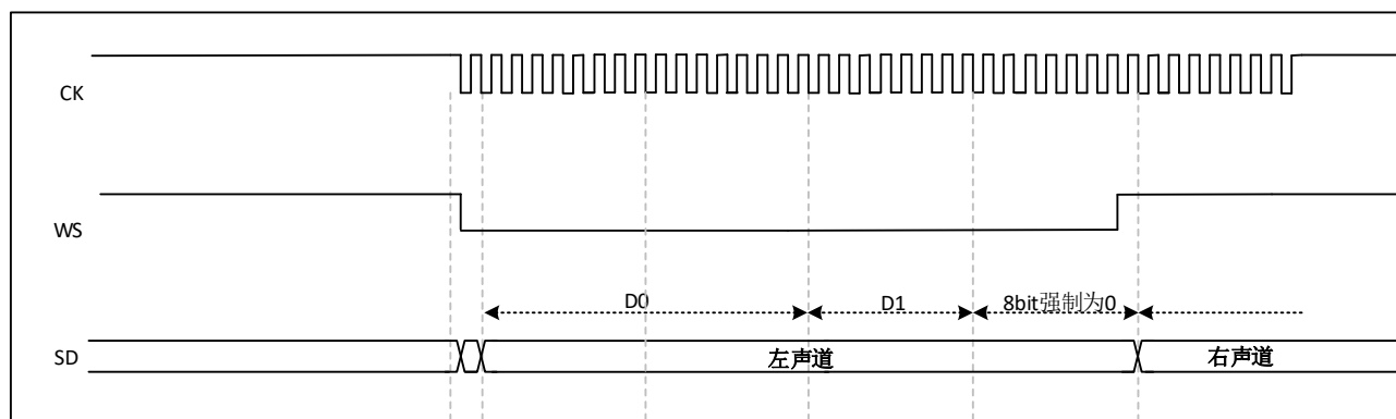
图 33-15 I2S 飞利浦协议波形(24 位帧, CKPOL=1)
