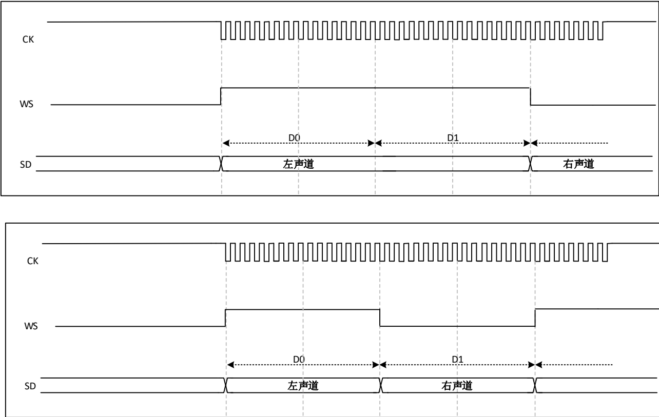
图 33-17 I2S MSB 对齐标准 (16/32 全精度, CKPOL=0)
