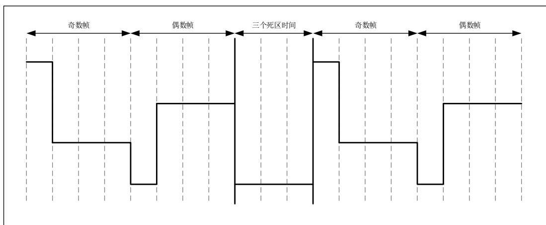
图 16-3 typeB 下的 CDRV[0]的波形
