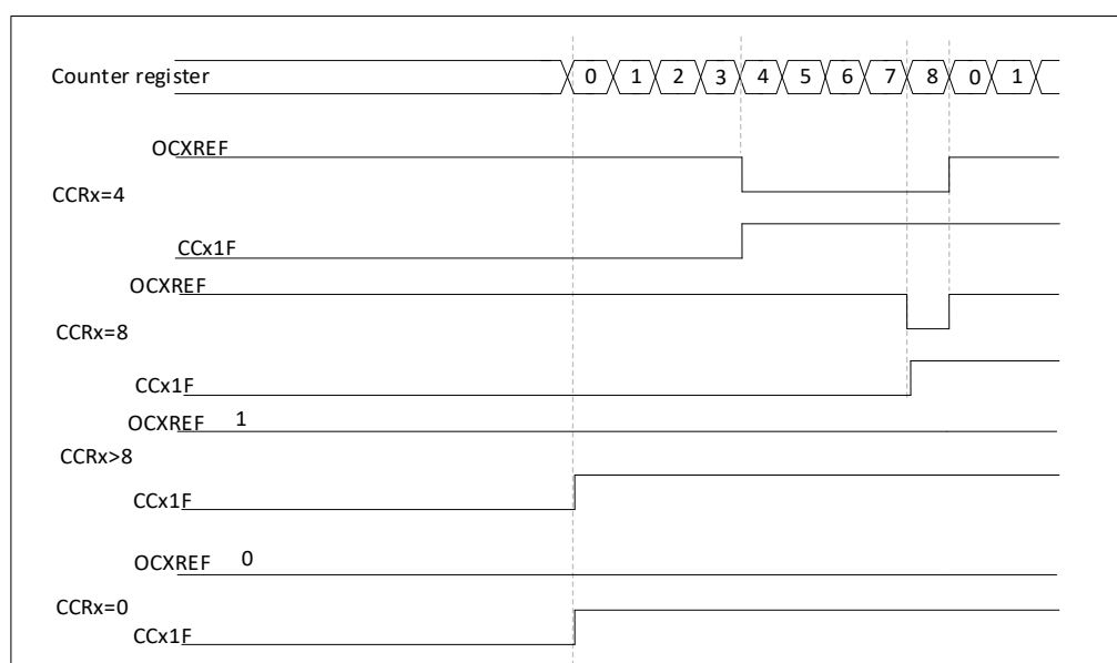
图 17-34 边沿对齐方式 PWM 输出波形 (ARR=8)
