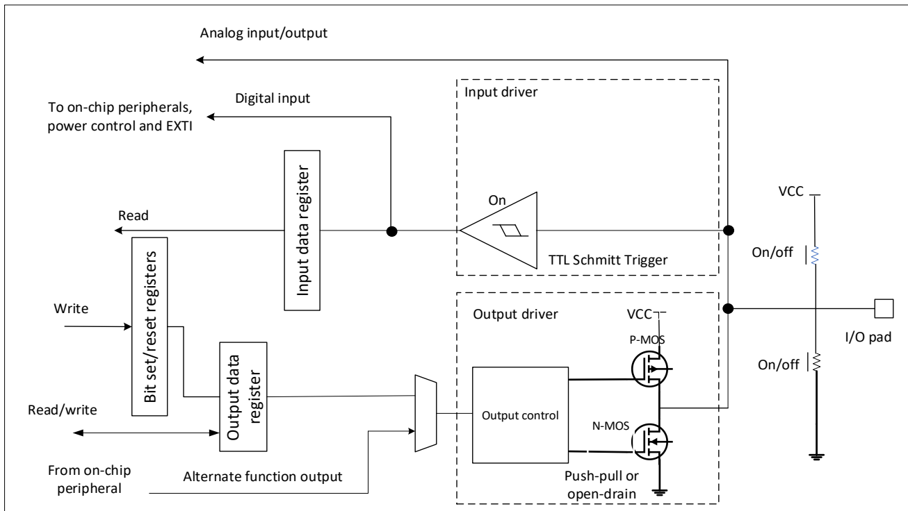
图 7-2 output configuration
