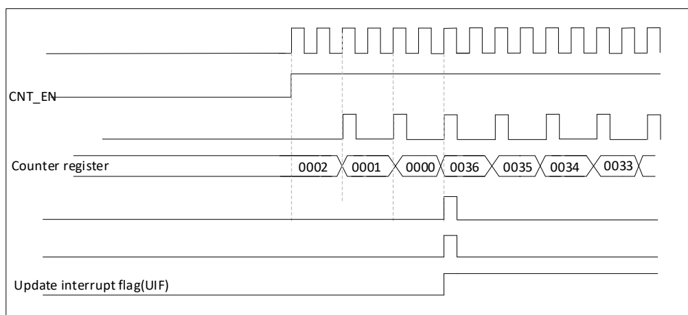
图 17-11 计数器时序图，内部时钟 2 分频
