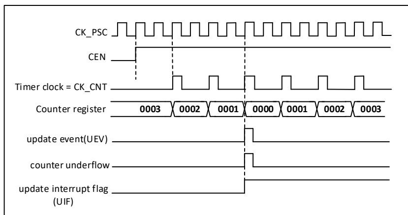
图 18-16 计数器时序图，内部时钟 2 分频
