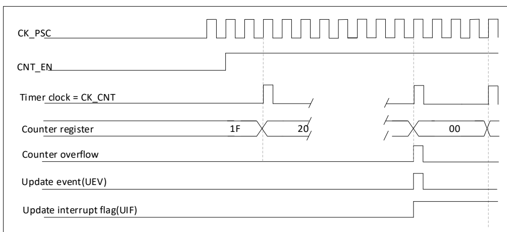
图 17-7 计数器时序图，内部时钟 N 分频
