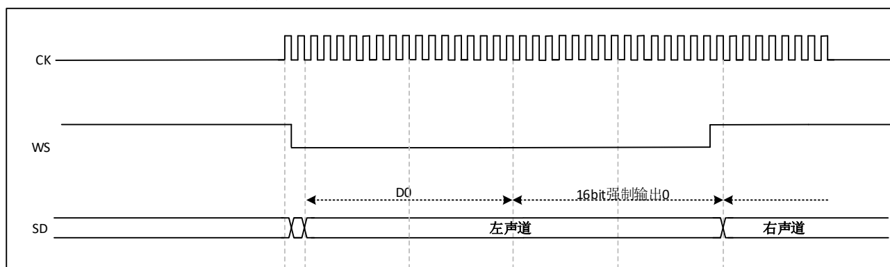
图 33-16 I2S 飞利浦协议波形(16 位扩展到 32 位)
