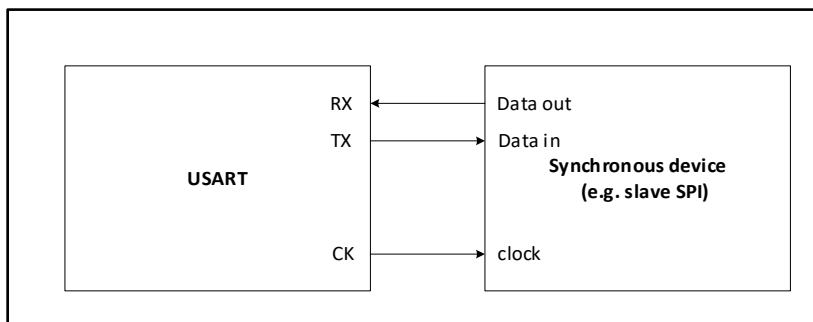
图 30-9 USART 同步传输例子
