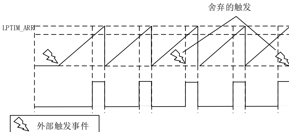
图 24-4 LPTIM 输出,连续计数模式
