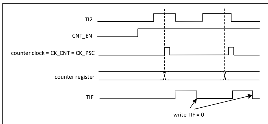
图 19-13 外部时钟模式 1 控制电路时序
