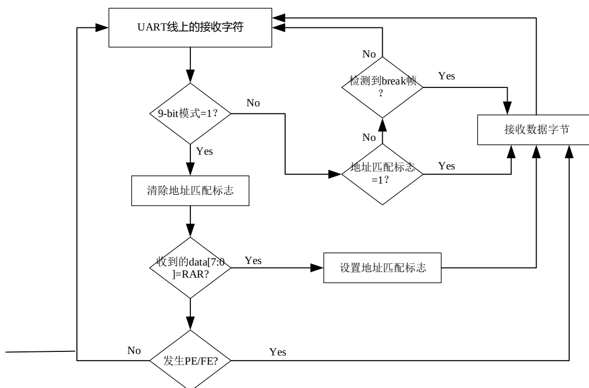
图 31-7 硬件地址匹配接收模式
