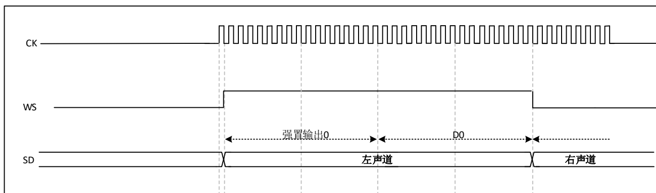
图 33-27 I2S LSB 对齐标准(16 位扩展到 32 位, CKPOL=0)
