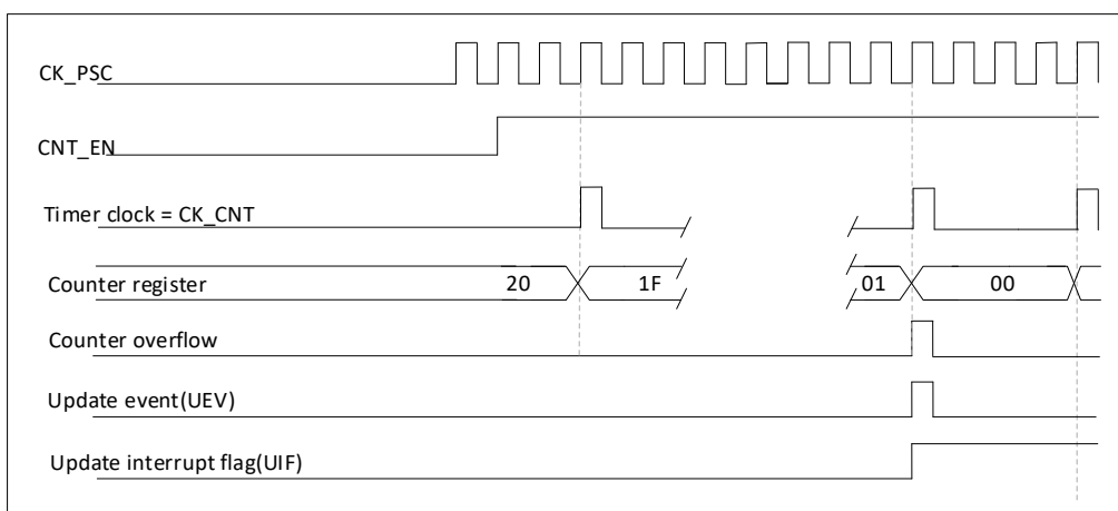
图 17-18 计数器时序图，内部时钟 N 分频
