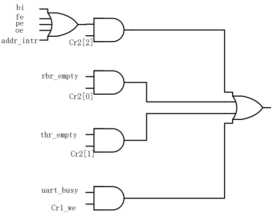
图 31-8 中断映射图
