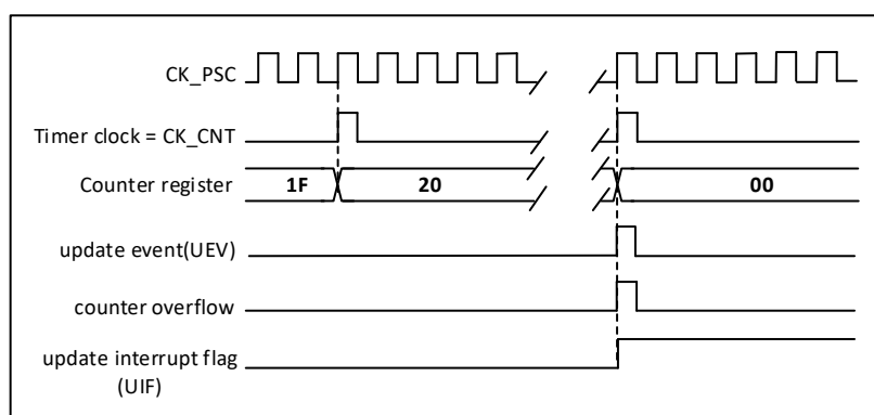
图 18-7 计数器时序图, 内部时钟 N 分频
