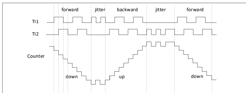
图 17-46 TI1FP1 极性反相时的编码器接口模式
