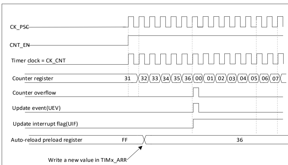
图 17-8 计数器时序图，ARPE=0 时更新事件 (TIM1_ARR 未预装载)
