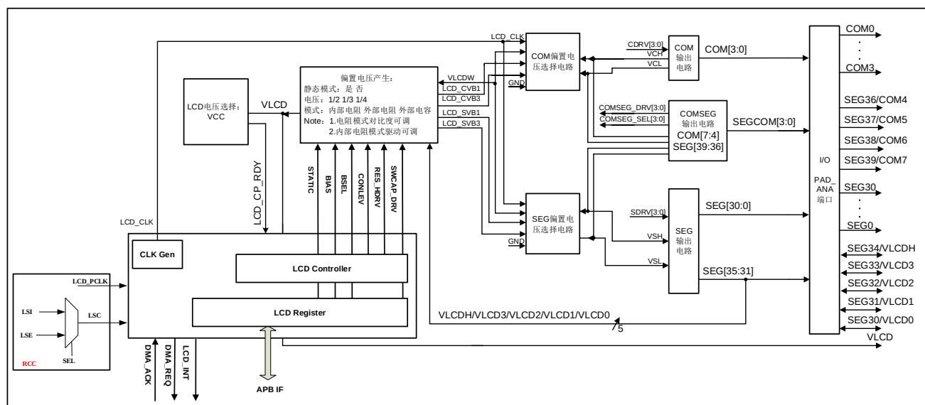
图 16-1 LCD 控制器框图
