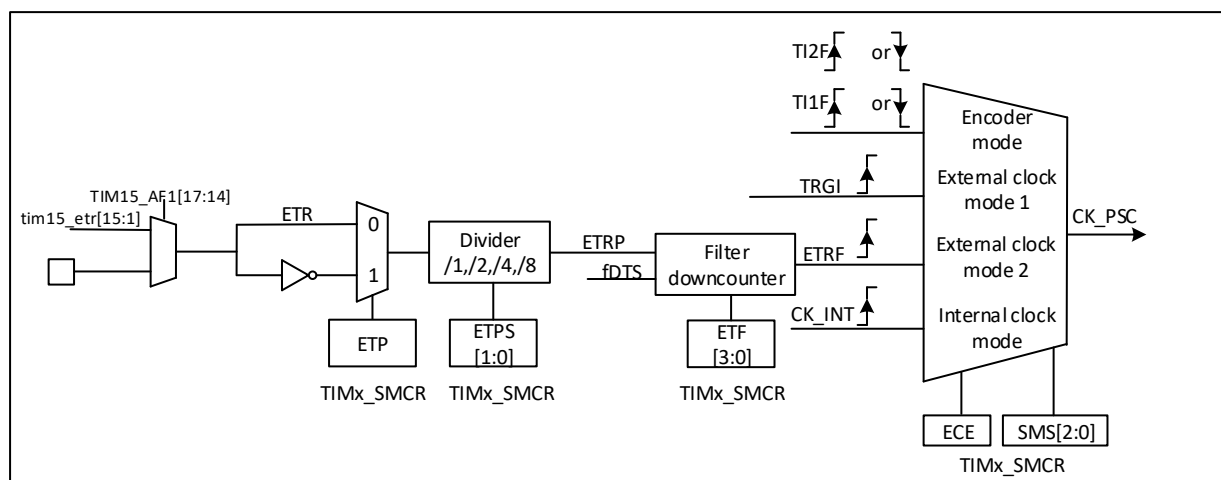
图 19-14 外部触发输入 ETR 连接
