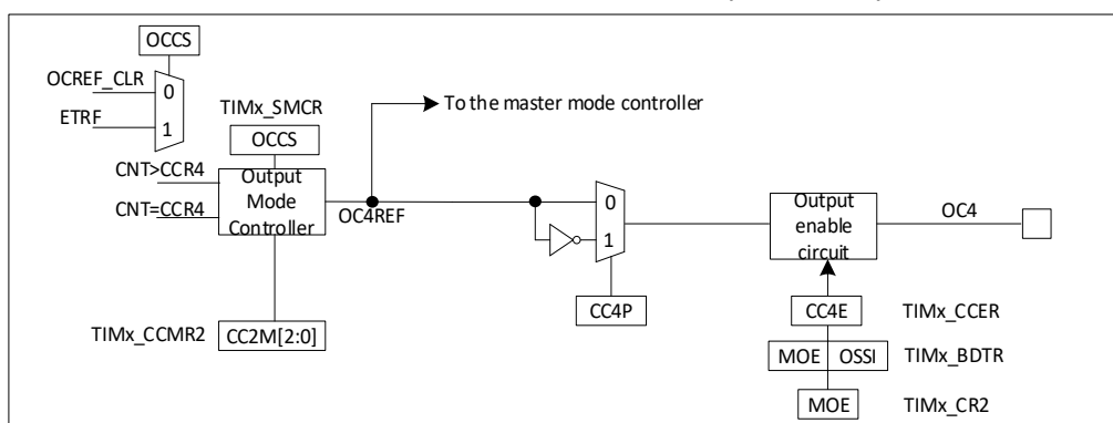
图 17-31 捕获/比较通道的输出阶段（通道 4）
