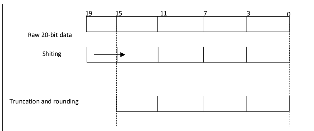
图 12-20 20bit to 16bit result truncation
