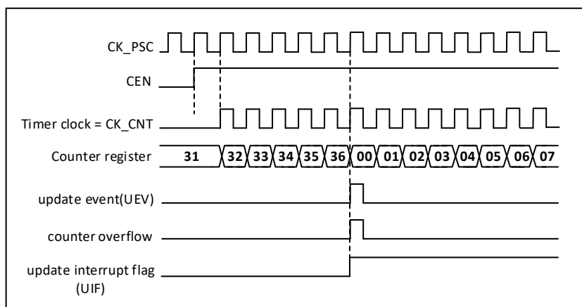
图 18-4 计数器时序图，内部时钟 1 分频
