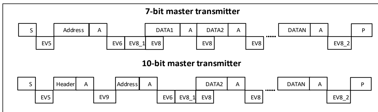
图 29-4 主机发送序列图
