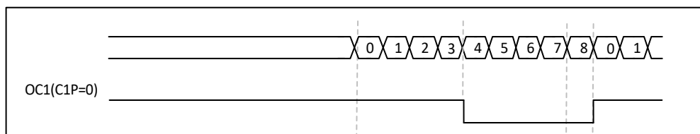
图 22-1 边沿对齐方式 PWM 输出，向上 (ARR=8)
