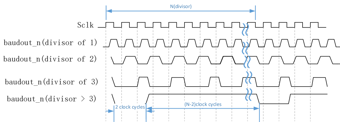
图 31-4 不同除数值的baudout_n输出的时序图
