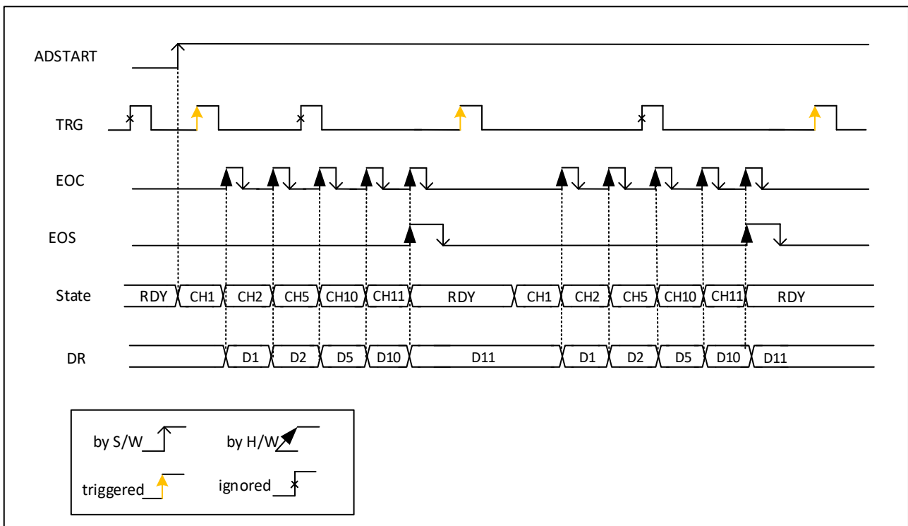
图 12-11 规则单次模式, 硬件触发
