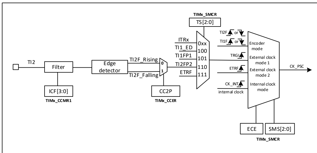
图 19-12 TI2 外部时钟连接示例
