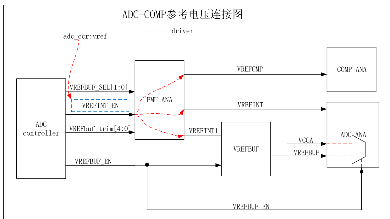
图 12-27 ADC VREF connection
