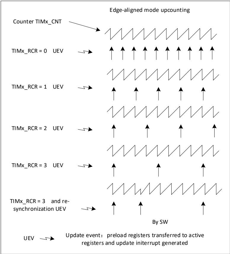
图 19-10 不同模式和 TIM15_RCR 寄存器设置下的更新频率示例
