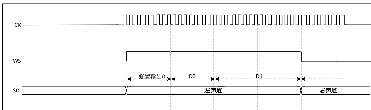
图 33-25 I2S LSB 对齐标准(24 位帧, CKPOL=0)
