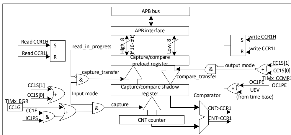
图 17-29 捕获/比较通道 1 主电路
