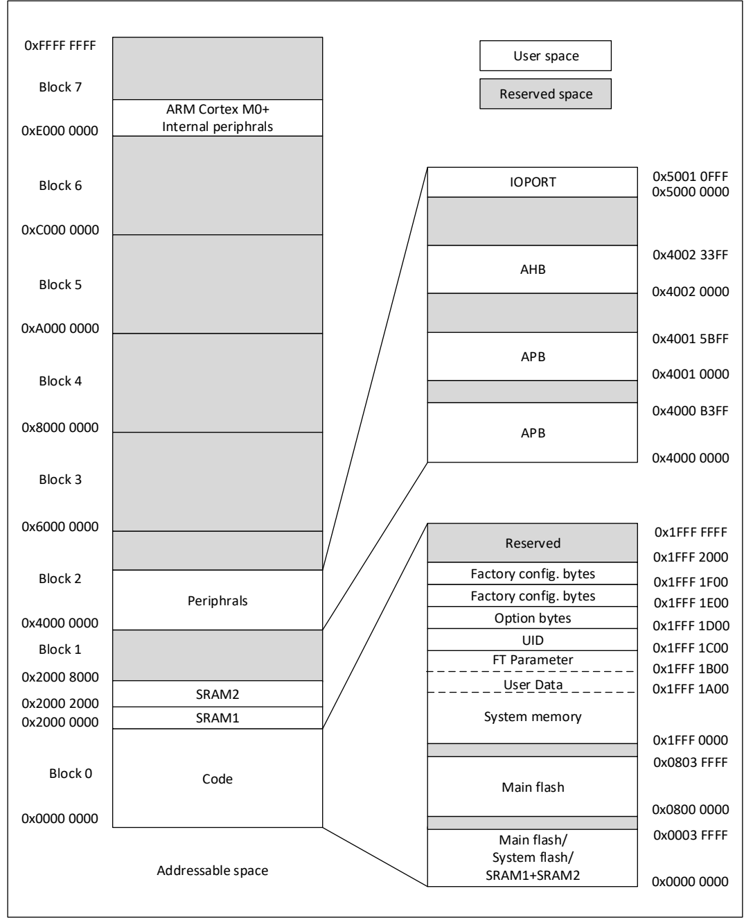
图 3-2 存储器映射
