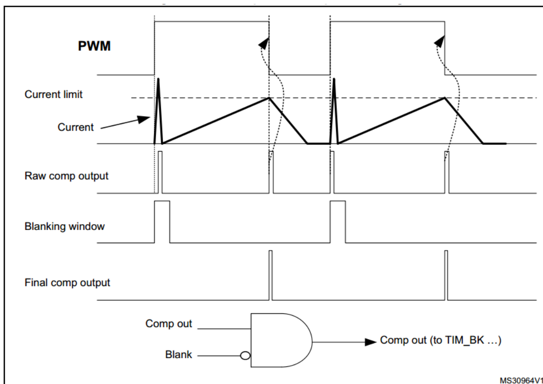
图 14-2 COMP 消隐
