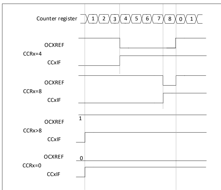
图 19-21 边沿对齐方式 PWM 输出波形 (ARR=8)
