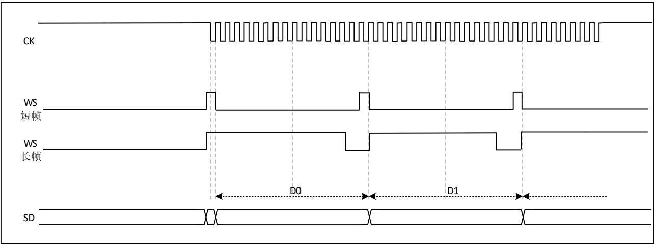
图 33-30 I2S PCM 标准 (16 位帧, CKPOL=1)
