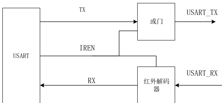
图 30-23 IrDA SIR ENDEC 框图
