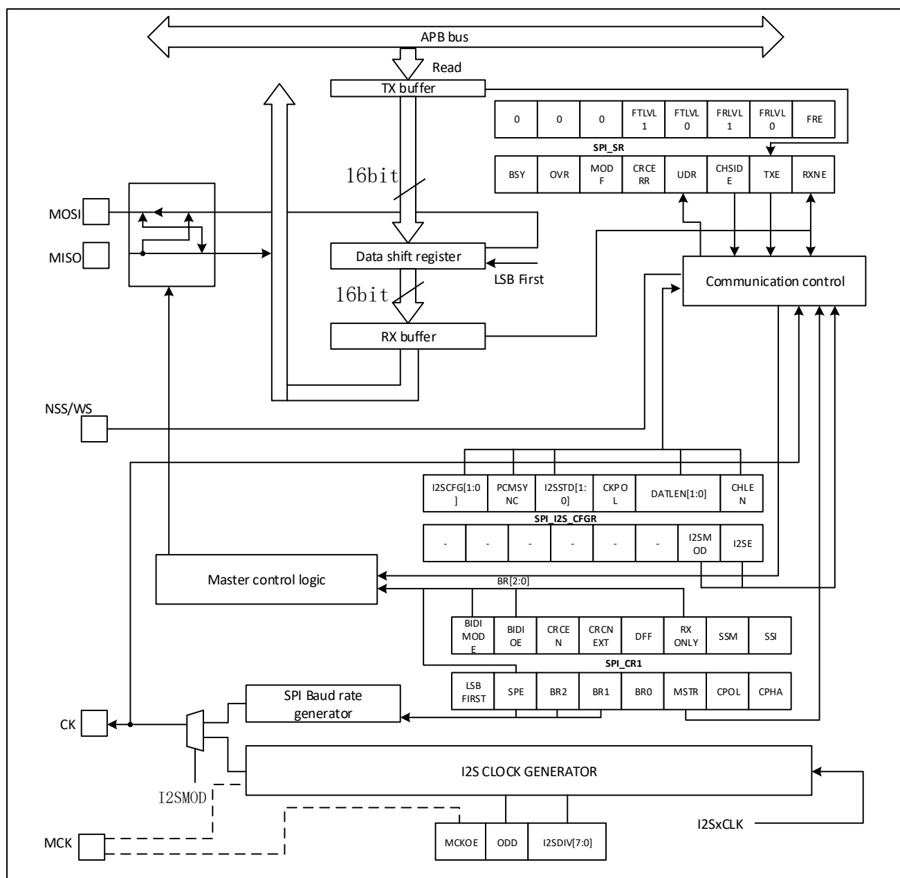
图 33-11 I2S 框图
