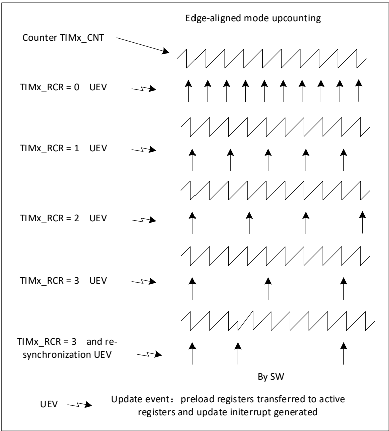
图 20-10 不同模式和 TIMx_RCR 寄存器设置下的更新频率示例
