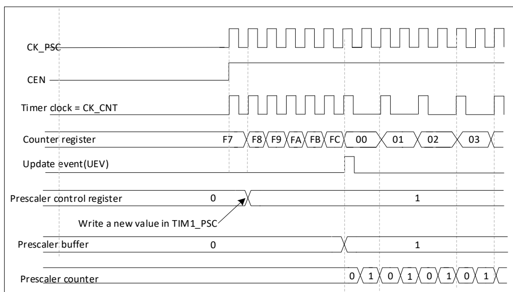
图 17-2 预分频器分频由 1 变为 2 时的计数器时序图
