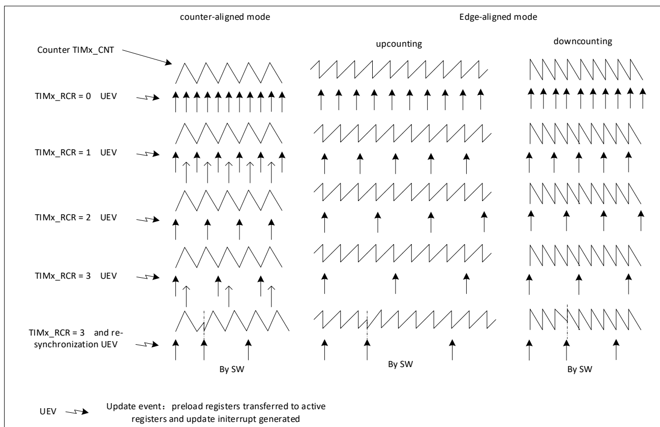
图 17-21 不同模式和 TIM1_RCR 寄存器设置下的更新频率示例
