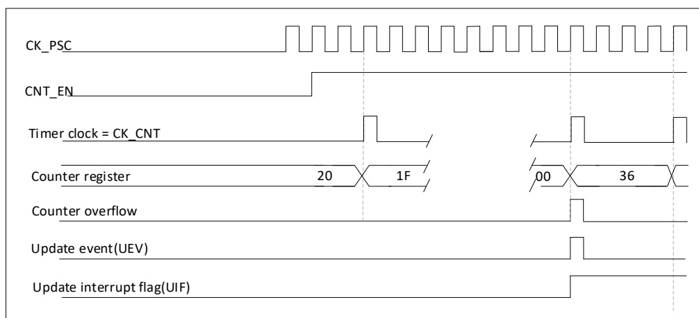
图 17-13 计数器时序图，内部时钟 N 分频
