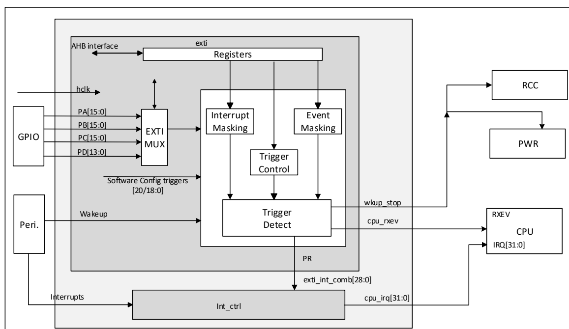
图 10-1 EXTI 框图
