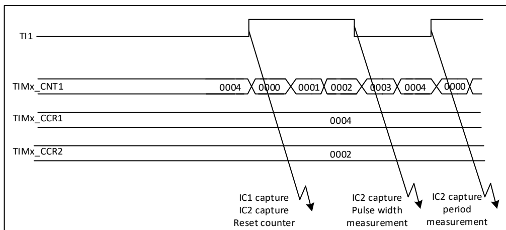
图 19-19 PWM 输入模式时序
