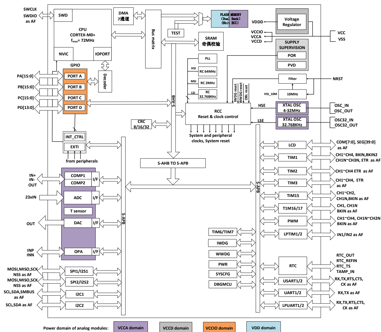
图 2-1 系统框图
