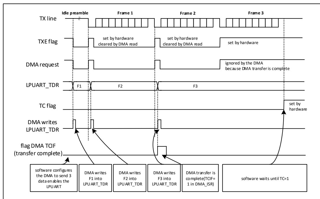
图 32-6 LPUART 用 DMA 发送
