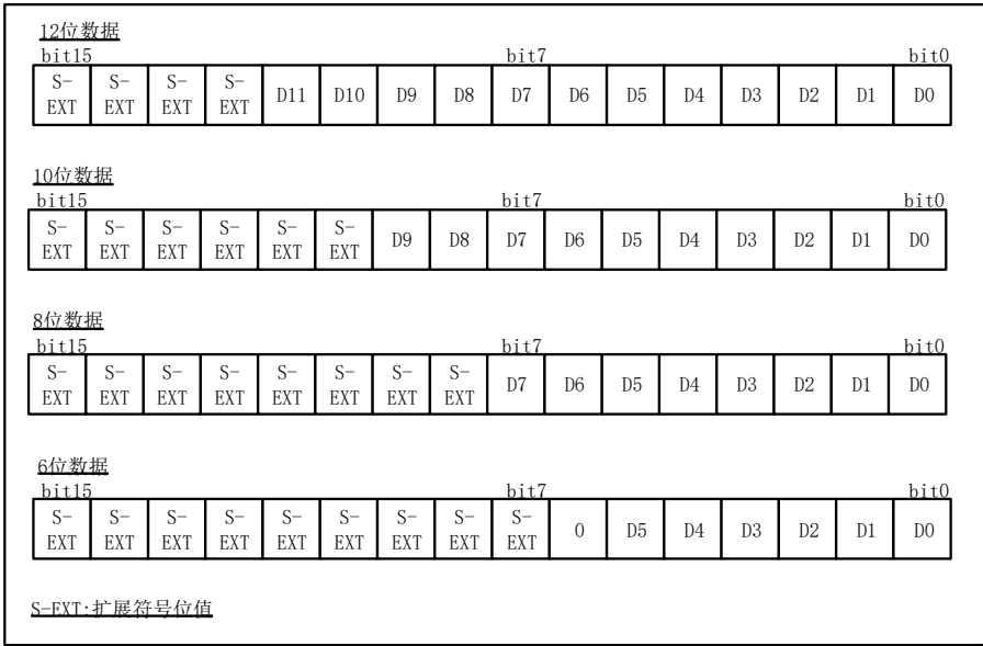
图 12-14 右对齐 (offset 使能, 有符号数)
