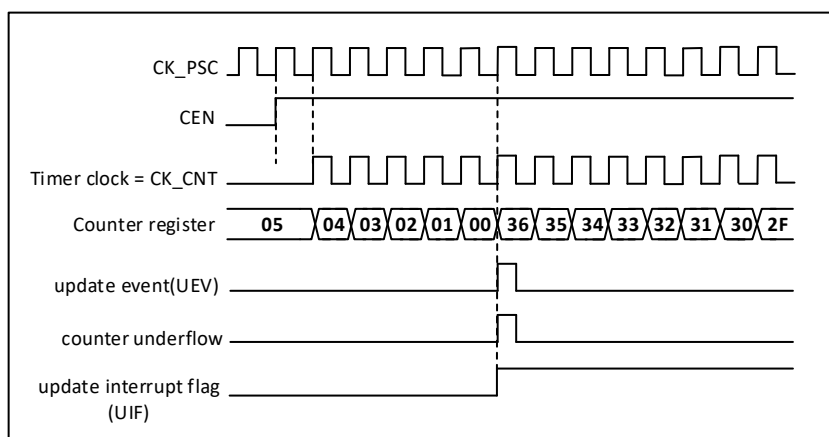
图 18-10 计数器时序图，内部时钟 1 分频
