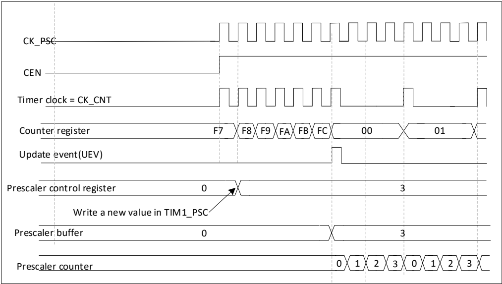
图 17-3 预分频器分频由 1 变为 4 时的计数器时序图
