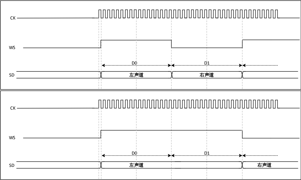
图 33-17 I2S MSB 对齐标准 (16/32 全精度, CKPOL=0)
