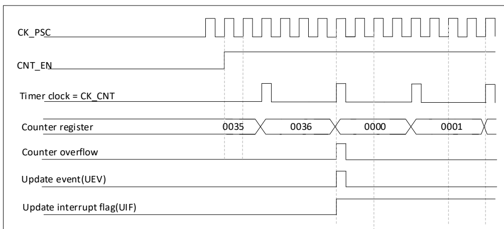
图 17-6 计数器时序图，内部时钟 4 分频
