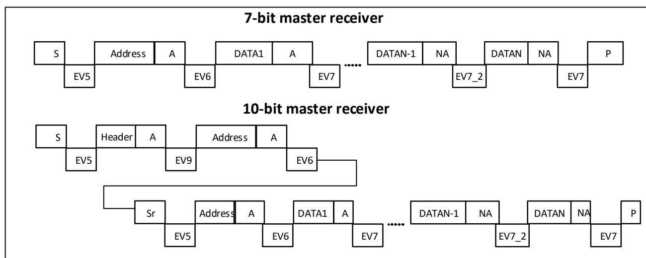
图 29-6 方法 2: 主机接收传输序列 N&gt;2
