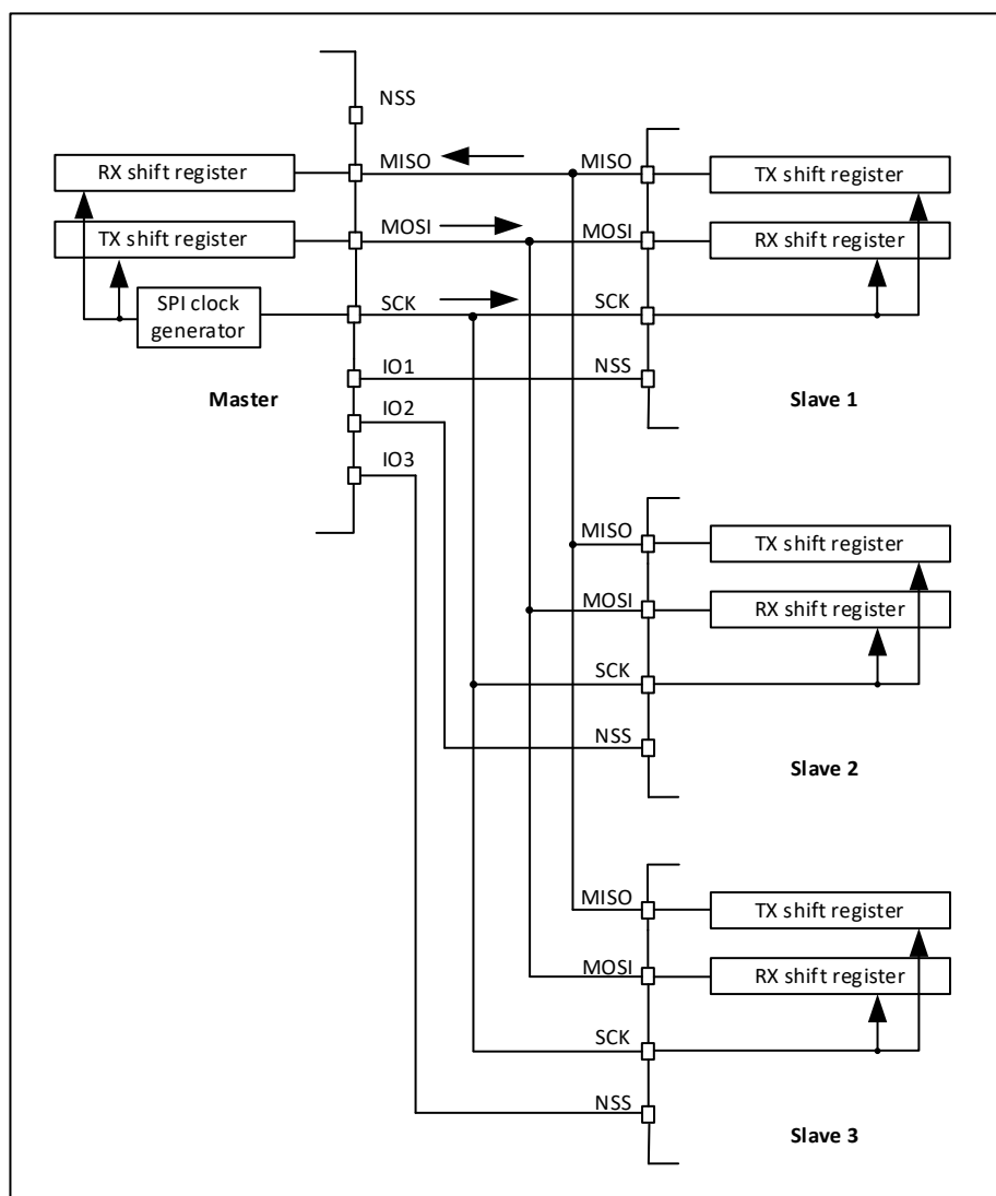
图 33-5 主机选择 3 个从机
