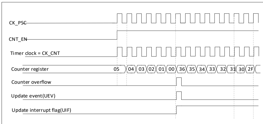
图 17-10 计数器时序图，内部时钟 1 分频
