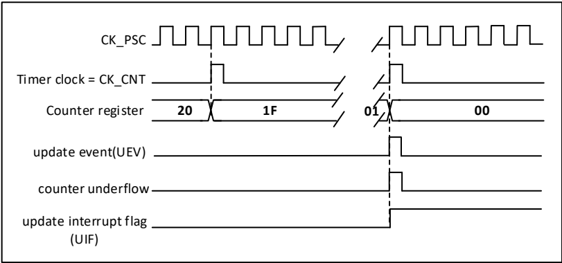
图 18-18 计数器时序图，内部时钟 N 分频
