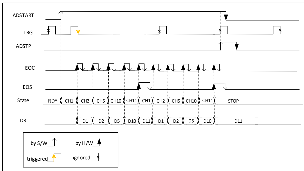
图 12-12 规则连续转换，硬件触发
