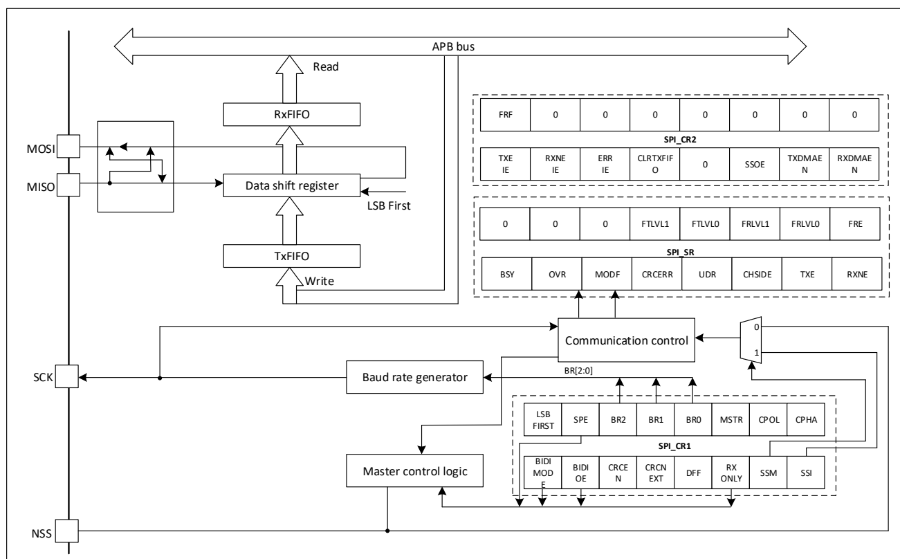
图 33-1 SPI 框图
