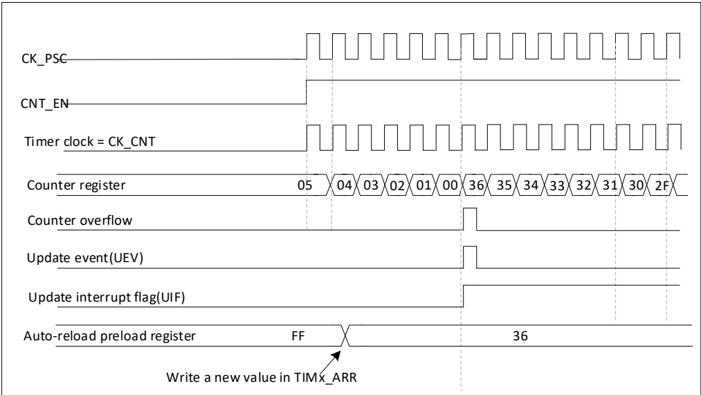
图 17-14 计数器时序图，未使用重复计数器时更新事件
