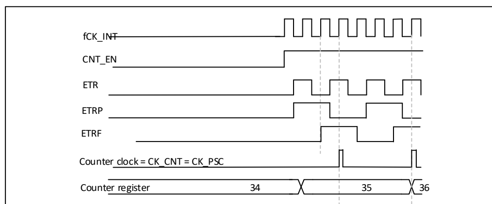
图 18-25 外部时钟模式 2 控制电路时序
