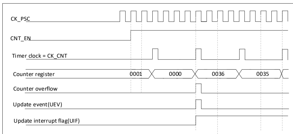
图 17-12 计数器时序图，内部时钟 4 分频
