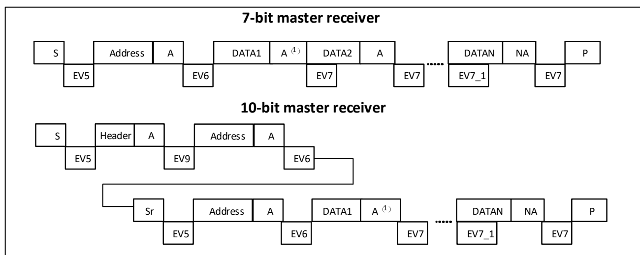
图 29-5 方法 1: 主机接收时的传输序列
