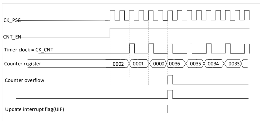
图 17-16 计数器时序图, 内部时钟 2 分频, TIM1_ARR=0x36
