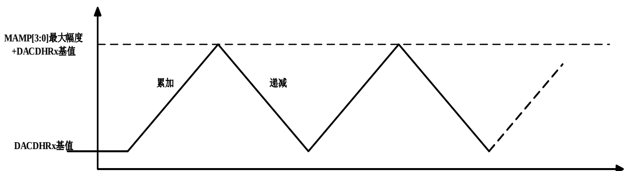
图 13-7 DAC 三角波生成
