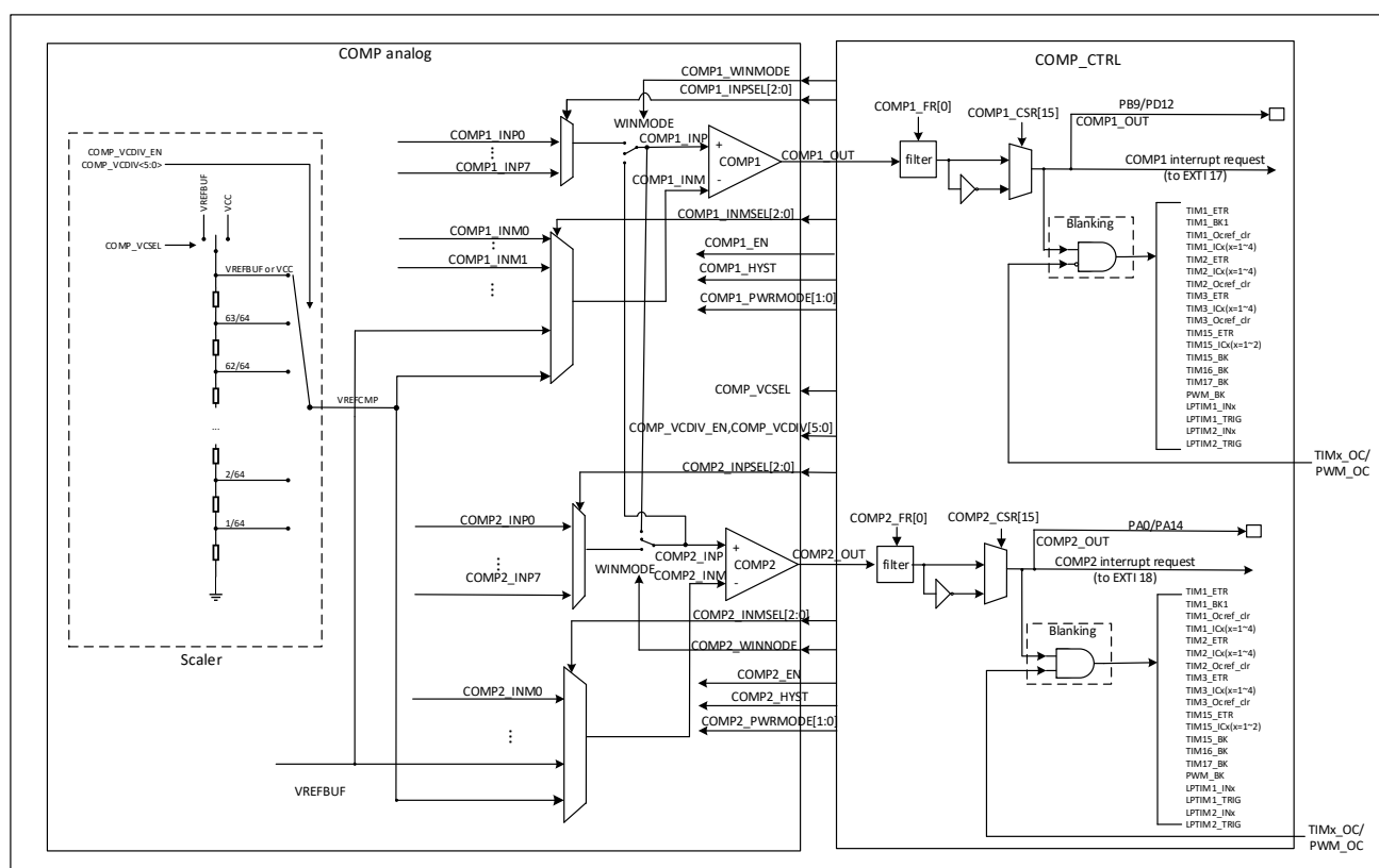
图 14-1 COMP 框图
