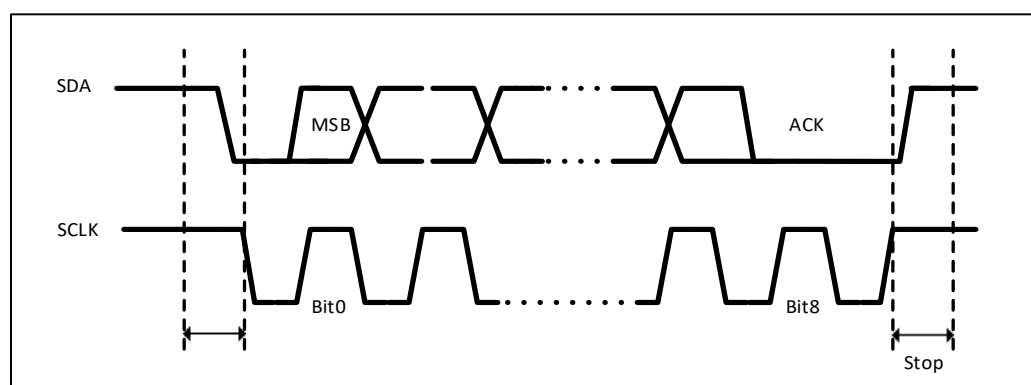
图 29-1 I2C 总线协议
