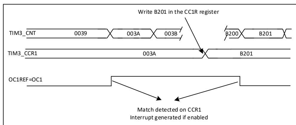
图 18-30 输出比较模式, 翻转 OC1
