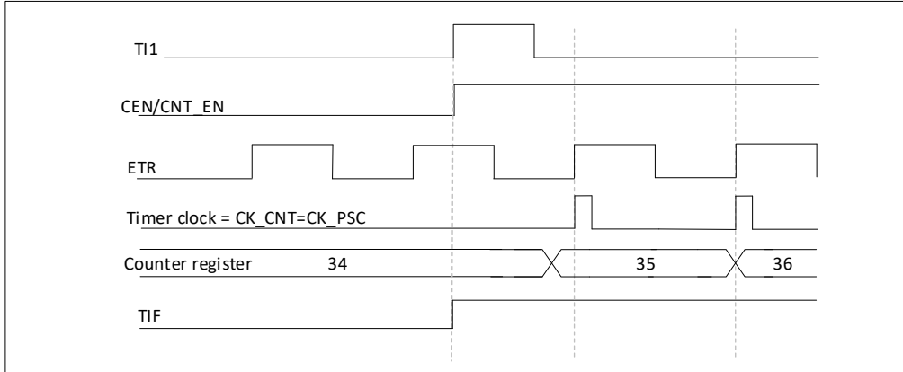
图 17-51 外部时钟模式 2+触发模式下的控制电路
