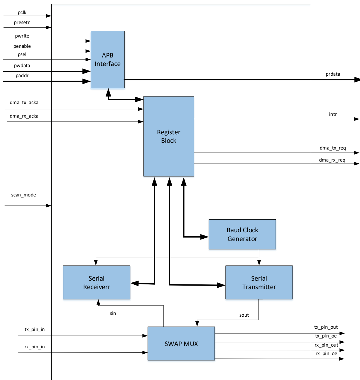
图 31-1 UART 框图
