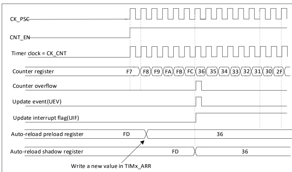
图 17-20 计数器时序图，ARPE=1 时的更新事件(计数器上溢)
