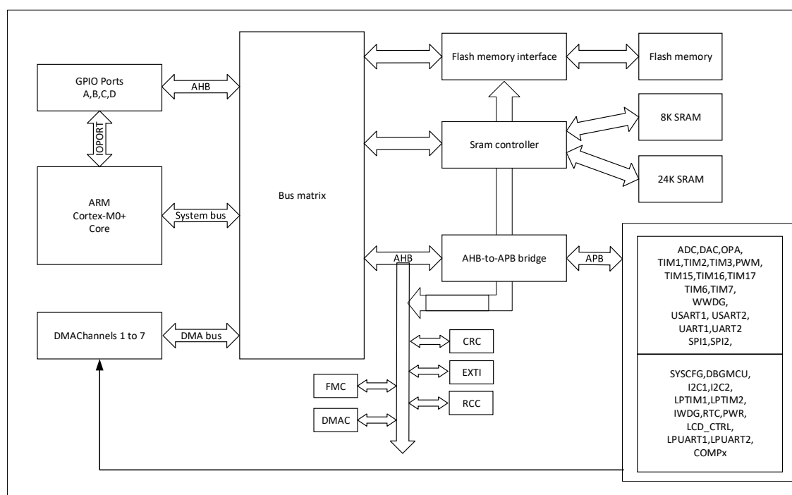
图 3-1 系统总线架构
