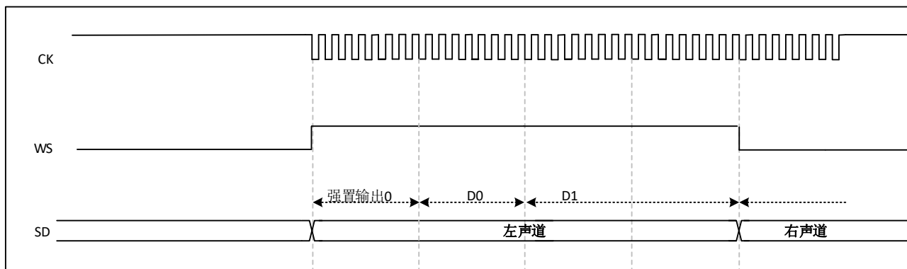
图 33-25 I2S LSB 对齐标准(24 位帧, CKPOL=0)
