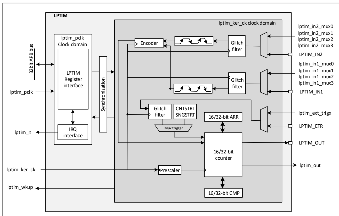
图 24-1 LPTIM 框图
