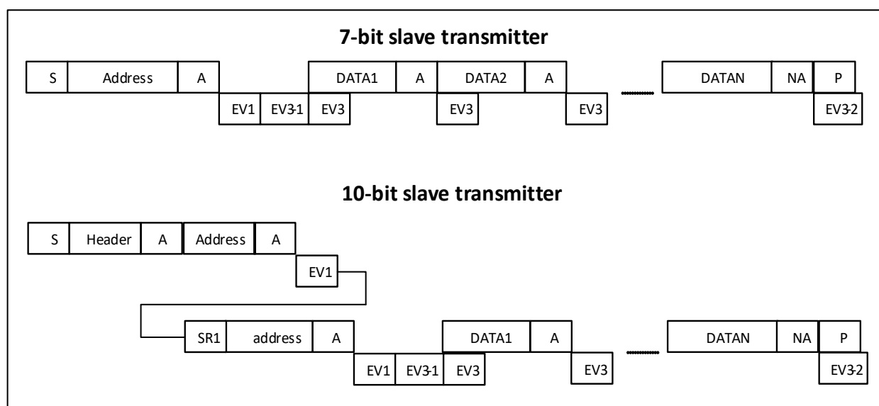
图 29-2 从机发送序列图
