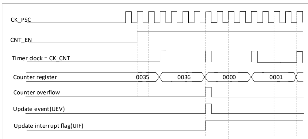
图 19-6 计数器时序图, 内部时钟 4 分频
