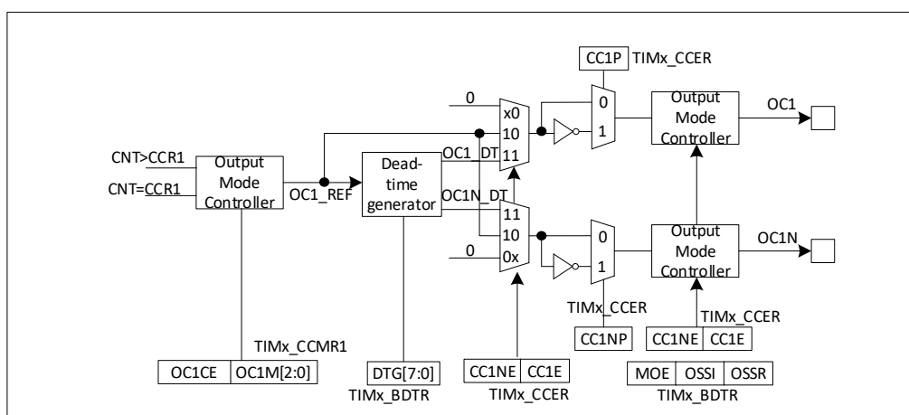
图 19-18 捕获/比较通道的输出阶段 (通道 1)
