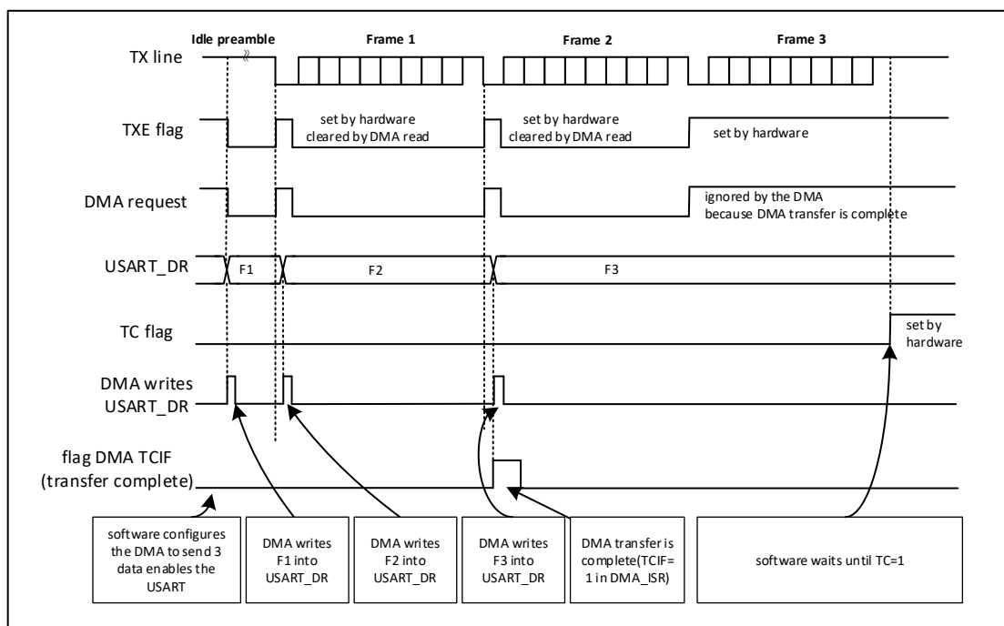
图 30-13 使用 DMA 发送
