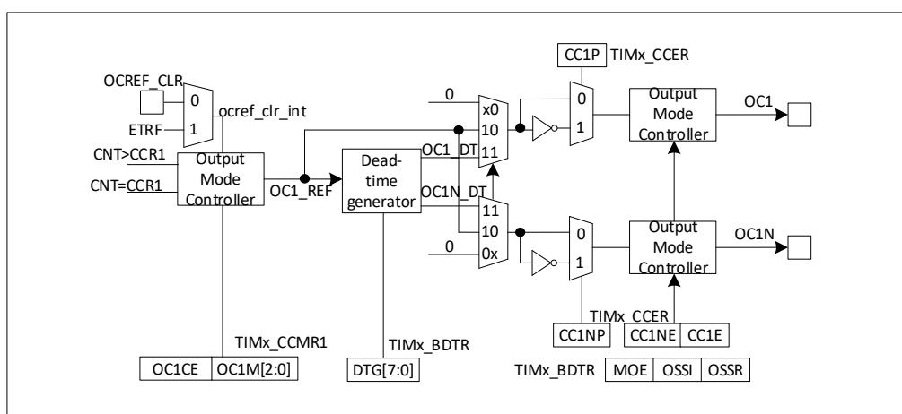
图 17-30 捕获/比较通道的输出阶段（通道 1 到 3）
