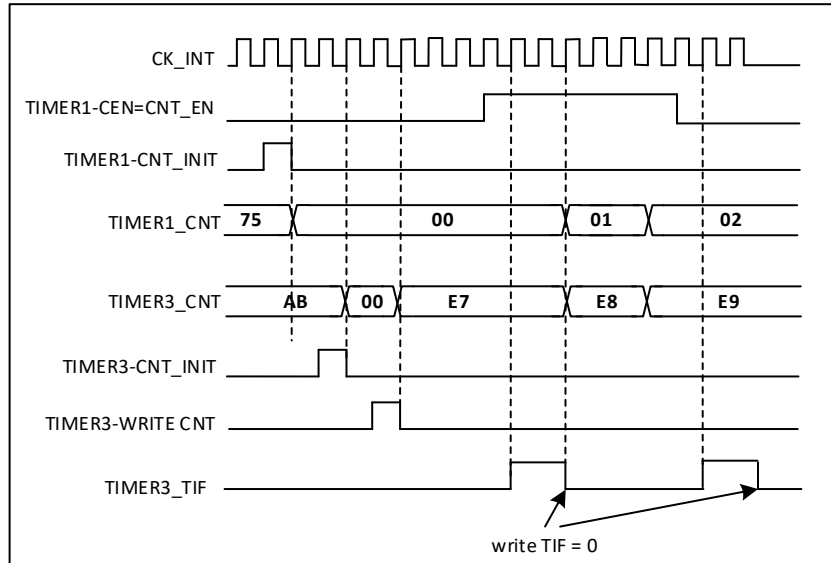
图 18-43 使用 TIM1 的使能信号对 TIM3 实施门控控制
