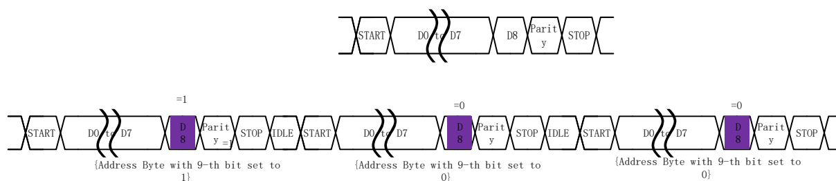
图 31-5 9位字符
