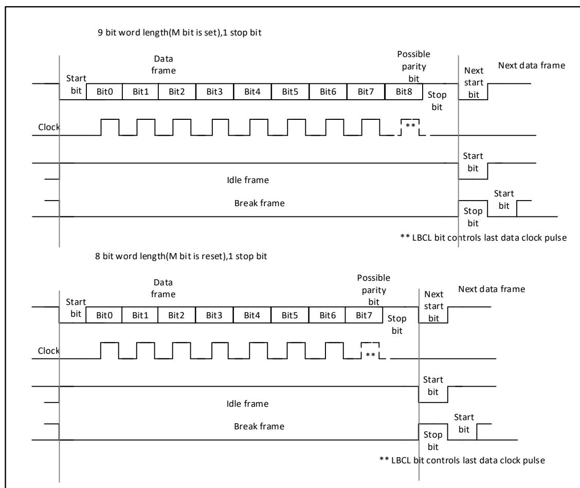
图 30-2 字长编程
