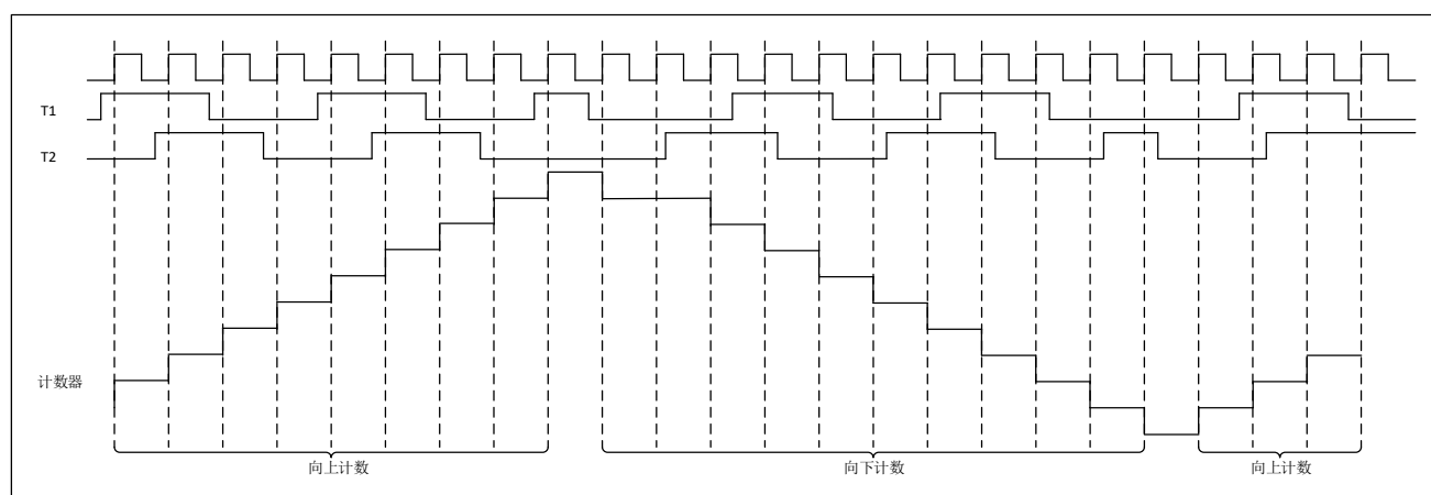
图 24-6 LPTIM 计数模式
