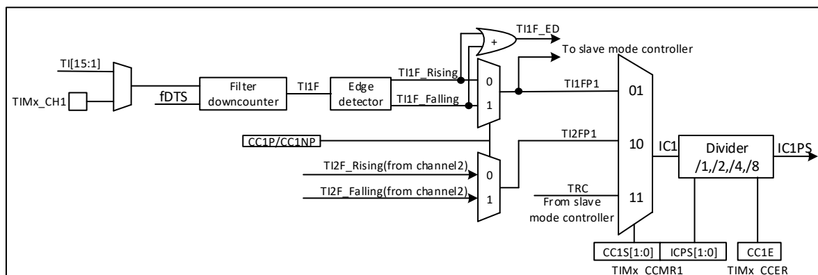
图 18-26 捕获/比较通道(示例:通道 1 输入阶段)
