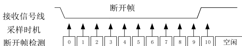
图 30-18 LIN 模式下的断开帧长度不够的情况
