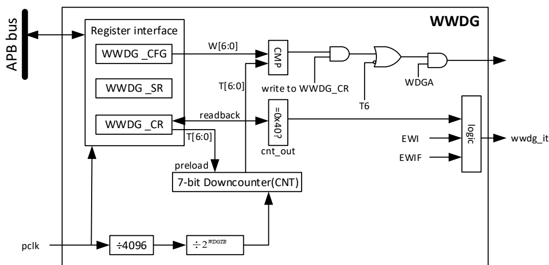
图 26-1 window watchdog 框图
