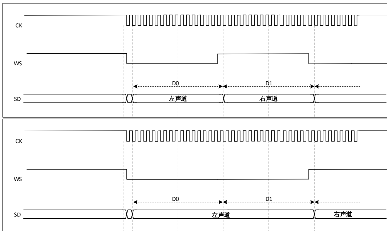
图 33-13 I2S 飞利浦协议波形 (16/32 位全精度, CKPOL=1)
