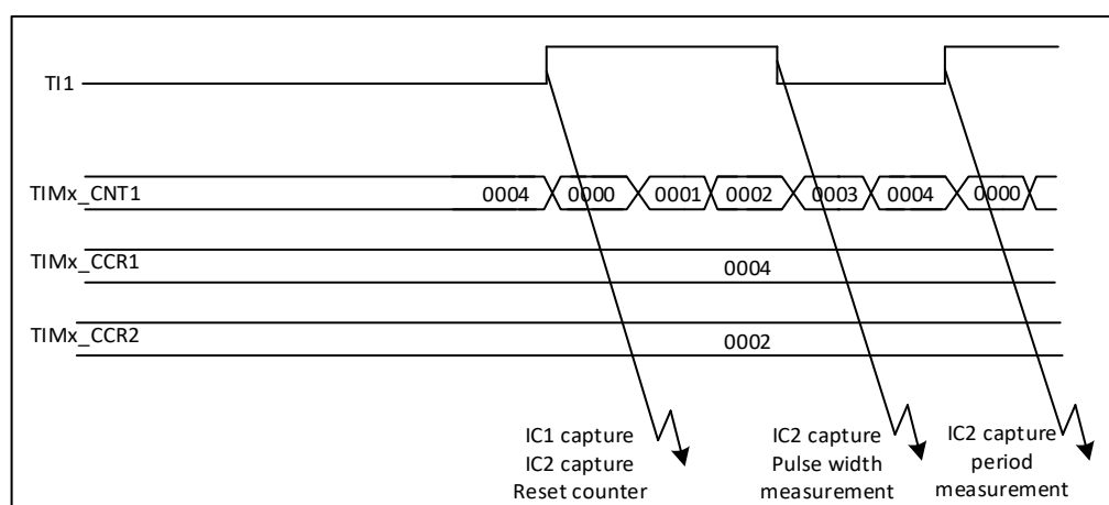
图 18-29 PWM 输入模式时序
