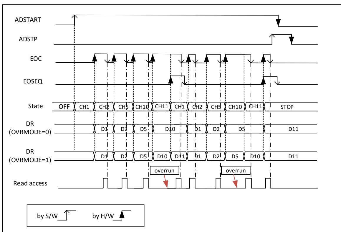
图 12-17 过载
