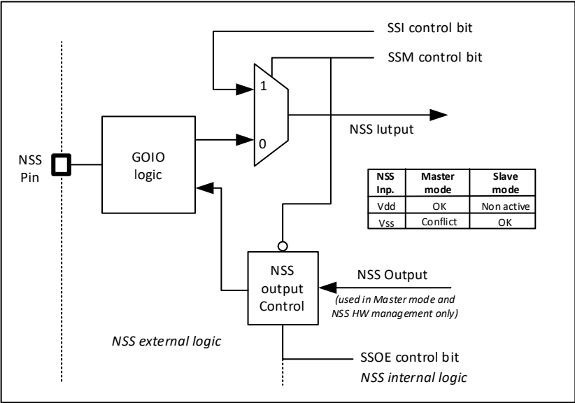
图 33-7 硬件/软件从模式选择管理
