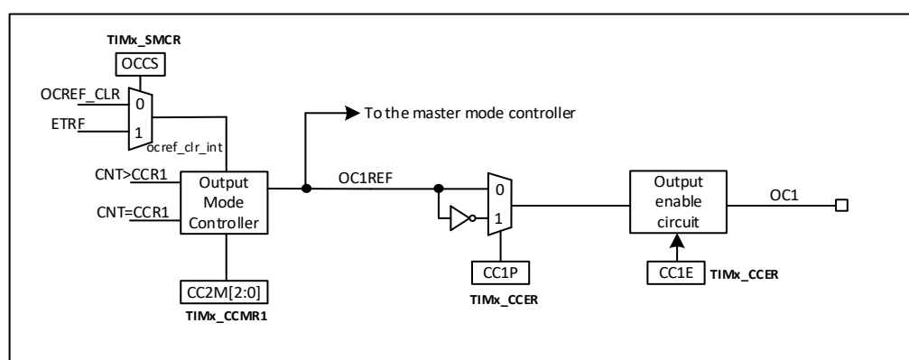
图 18-28 捕获/比较通道的输出阶段 (通道 1)
