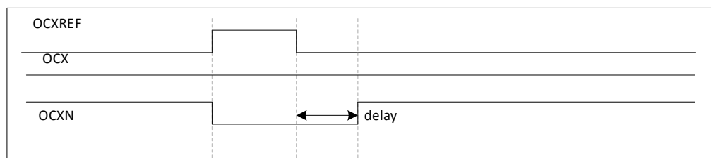
图 19-24 延迟时间大于正脉冲宽度的死区波形
