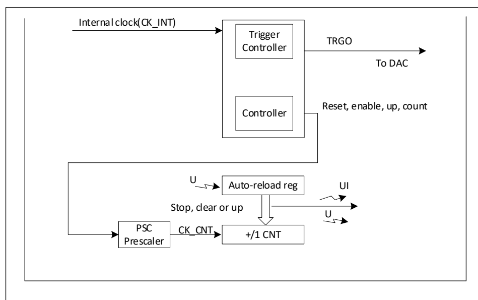
图 21-1 通用框图
