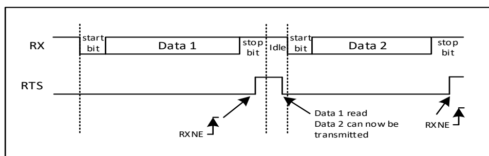
图 32-9 RTS 流控制
