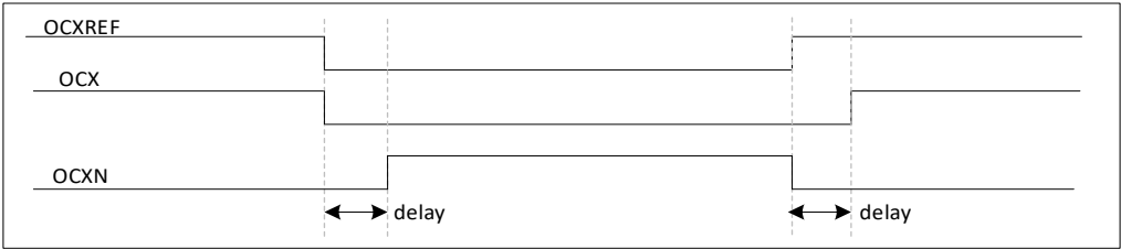
图 20-17 带死区插入的互补输出
