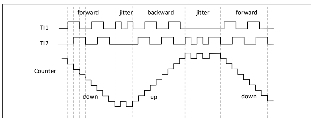
图 18-36 TI1FP1 极性反相时的编码器接口模式
