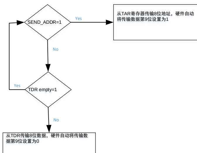
图 31-6 自动地址传输流程图
