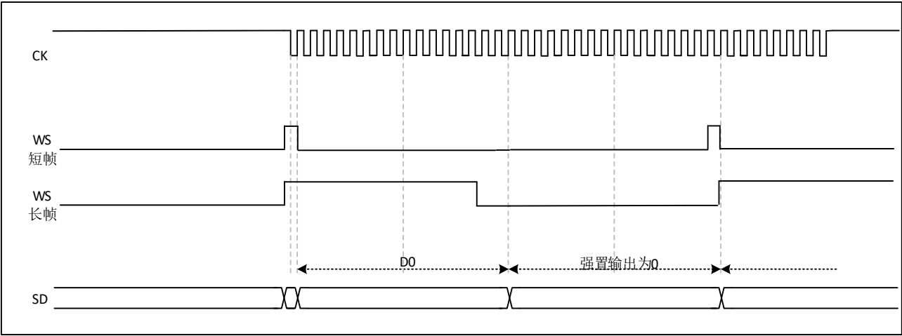
图 33-32 I2S PCM 标准 (16 位扩展到 32 位, CKPOL=1)
