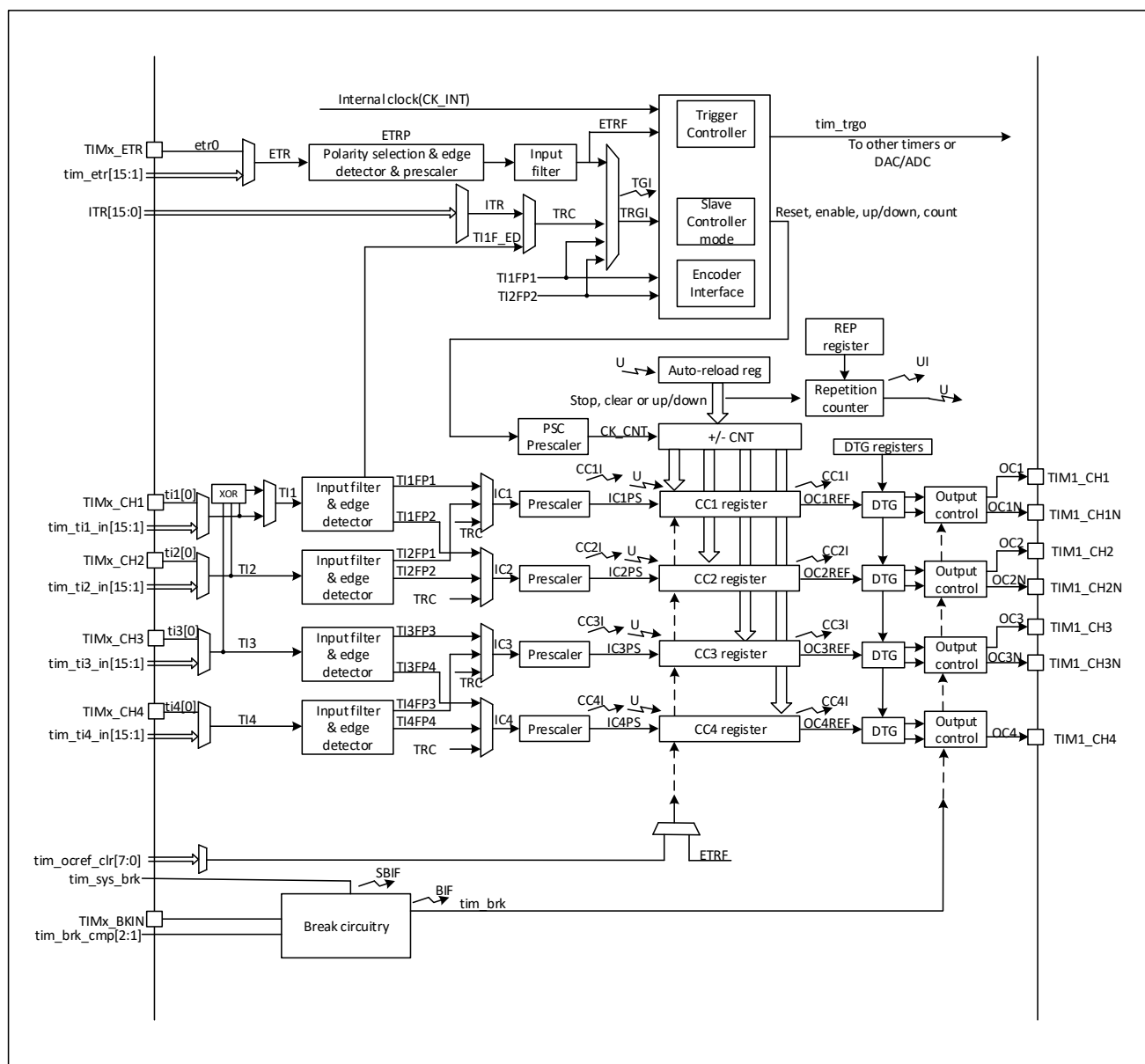
图 17-1 高级控制定时器框图
