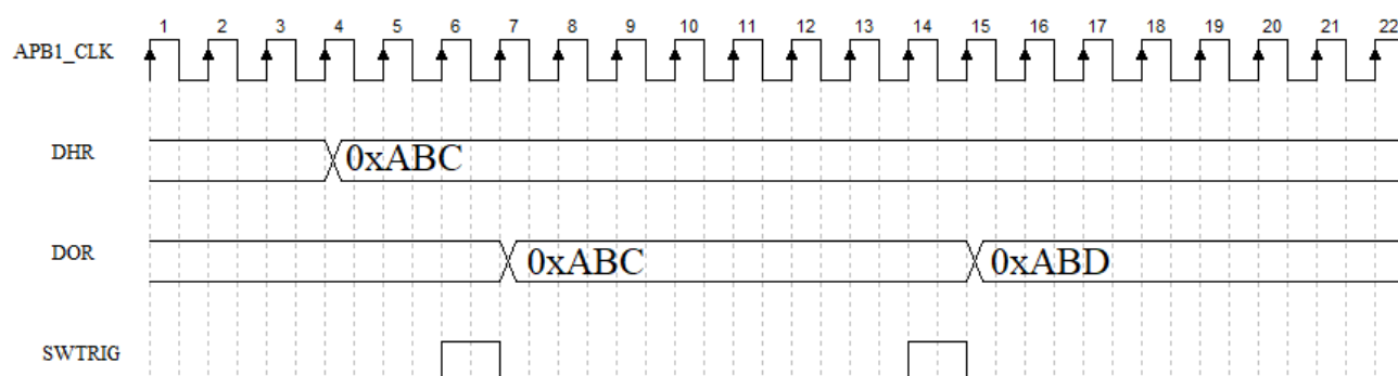
图 13-8 带三角生成的 DAC 转换(使能软件触发)
