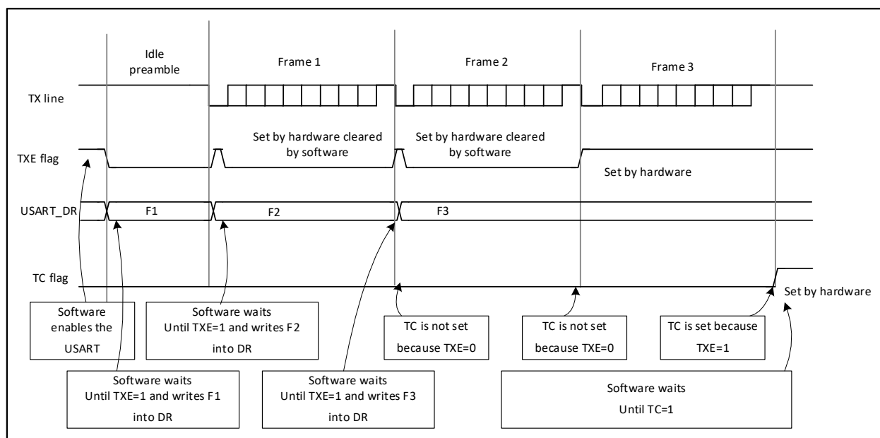
图 30-4 发送时的 TC/TXE 行为
