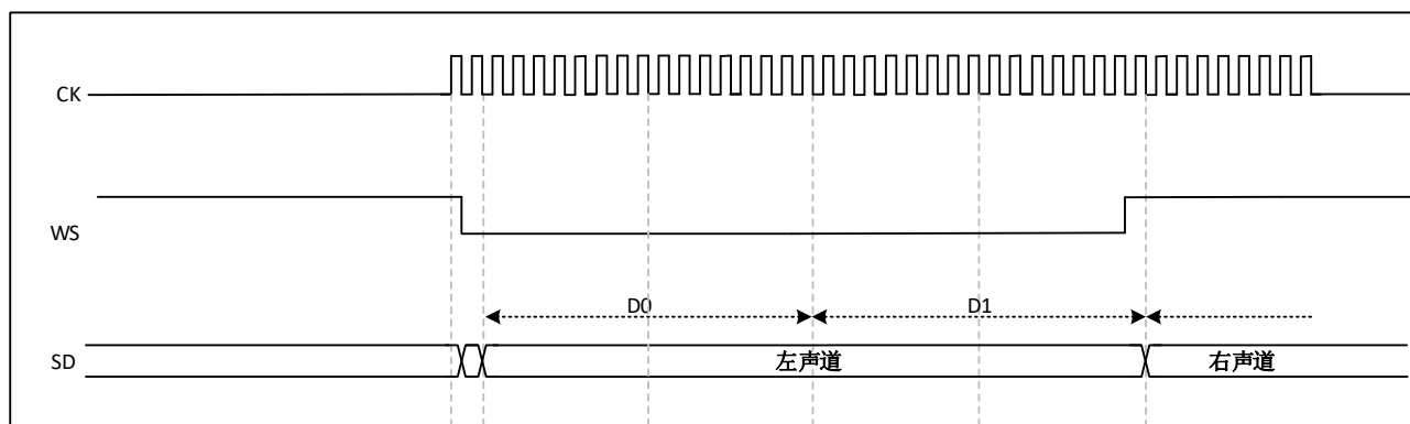
图 33-12 I2S 飞利浦协议波形 (16/32 位全精度, CKPOL=0)
