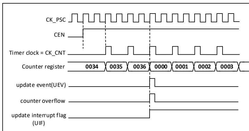
图 18-5 计数器时序图，内部时钟 2 分频
