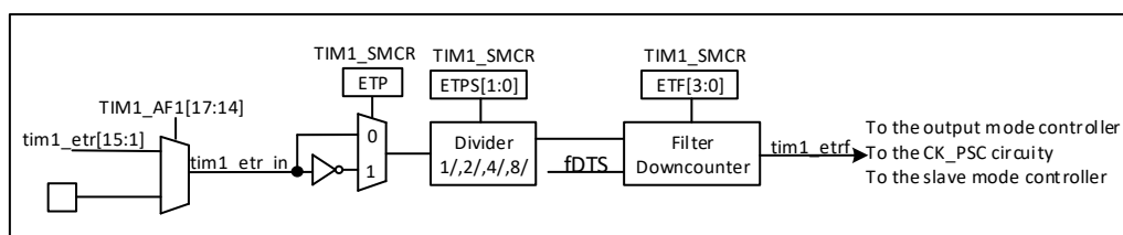
图 17-22 外部触发输入
