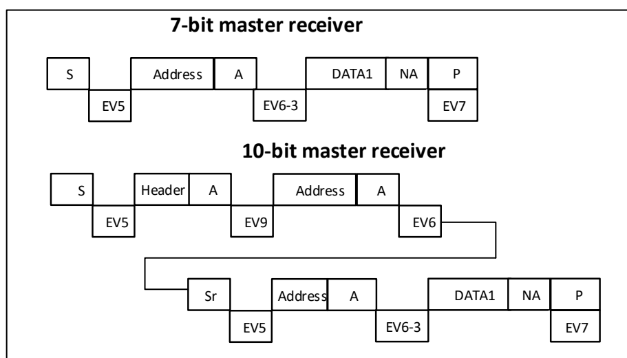
图 29-8 Method 2: 主机接收时的传输时序 N=1
