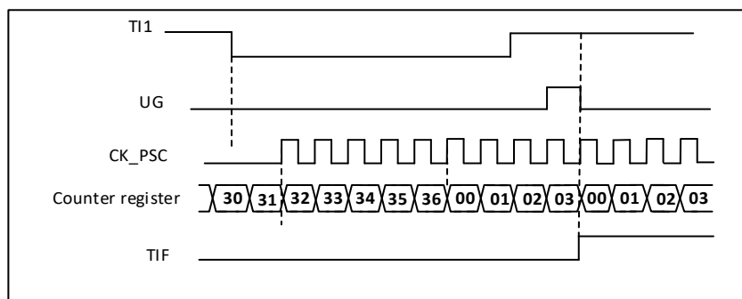
图 19-28 复位模式下的控制电路
