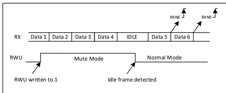
图 30-7 使用空闲帧检测的静默模式
