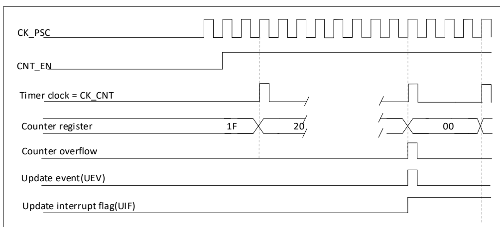
图 20-7 计数器时序图，内部时钟 N 分频
