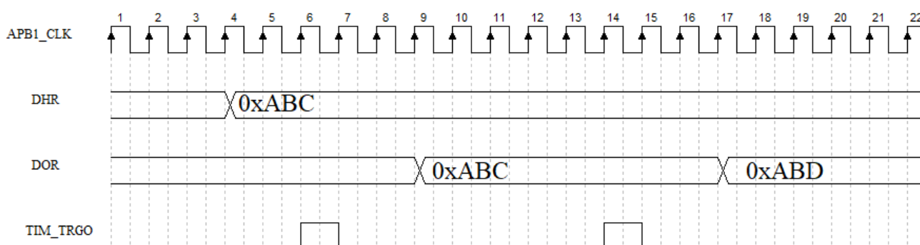
图 13-9 带三角生成的 DAC 转换(使能硬件触发)
