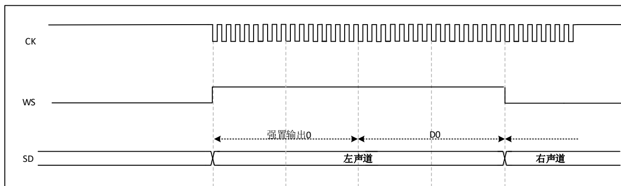
图 33-28 I2S LSB 对齐标准(16 位扩展到 32 位, CKPOL=1)
