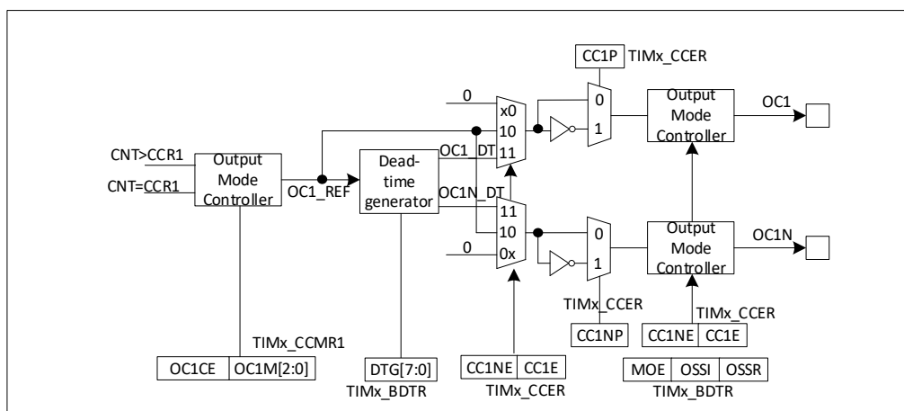
图 20-14 捕获/比较通道的输出阶段 (通道 1)
