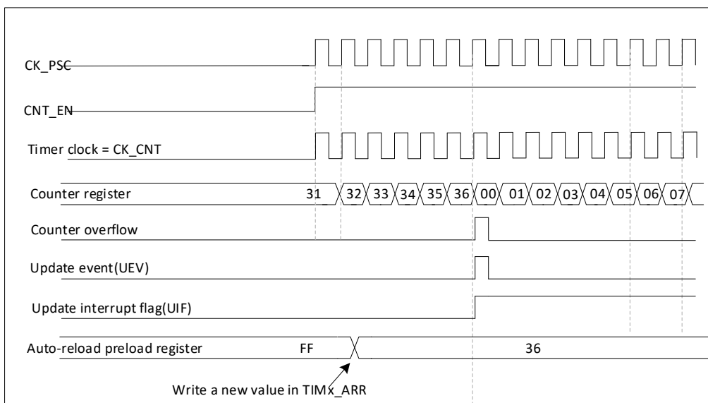
图 19-8 计数器时序图, ARPE=0 时更新事件 (TIM15_ARR 未预装载)
