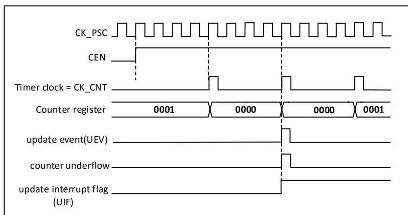
图 18-12 计数器时序图，内部时钟 4 分频
