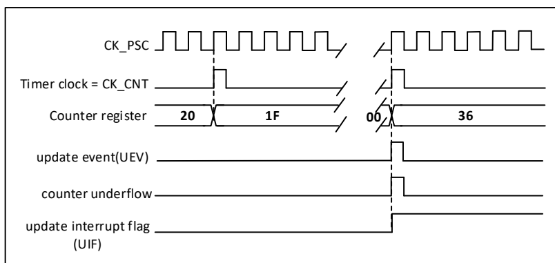
图 18-13 计数器时序图，内部时钟 N 分频
