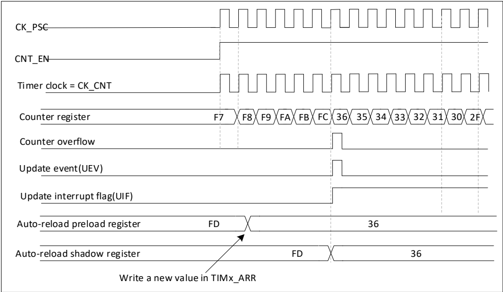
图 18-20 计数器时序图，ARPE=1 时的更新事件（计数器上溢）
