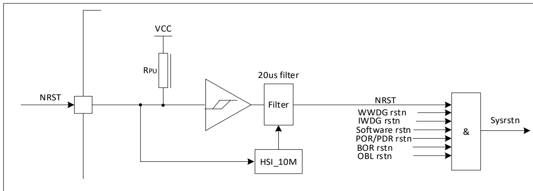
图 6-1 复位电路
