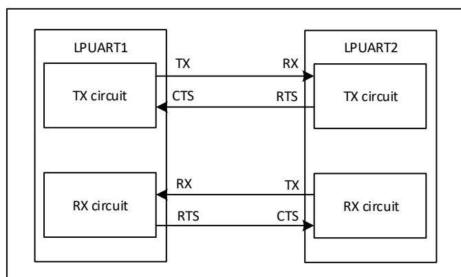
图 32-8 硬件流控制
