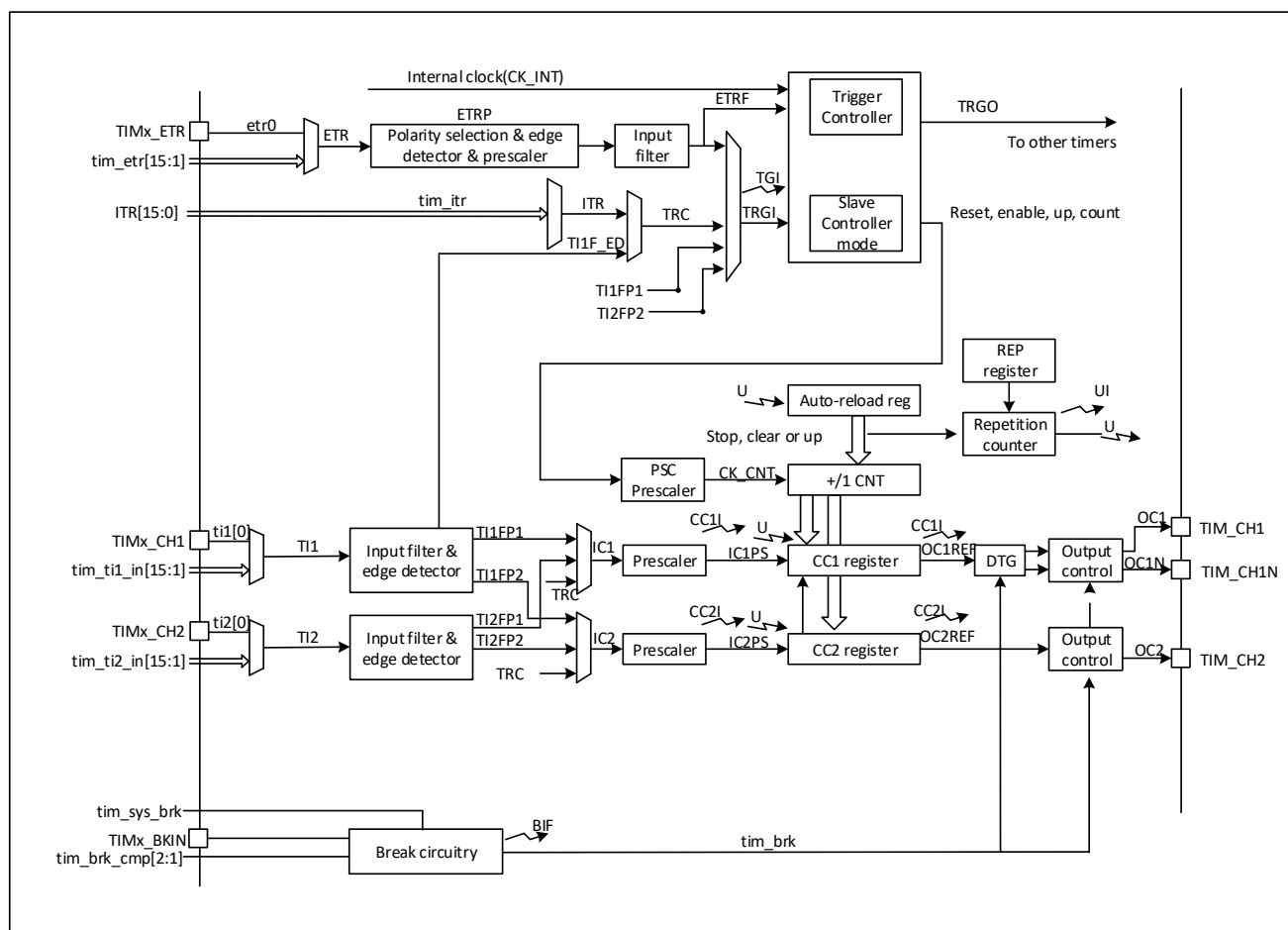
图 19-1 TIM15 框图
