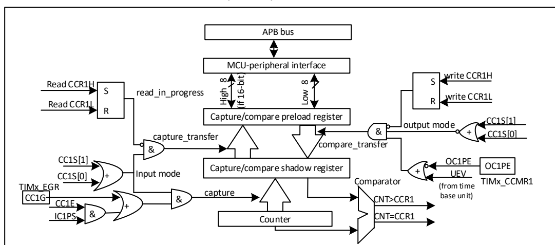
图 18-27 捕获/比较通道 1 主电路
