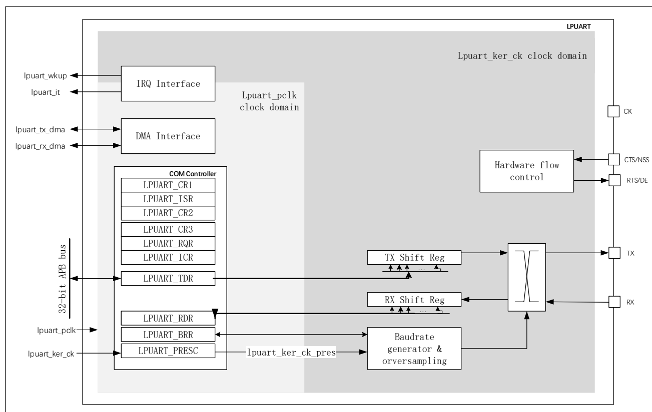
图 32-1 LPUART 框图
