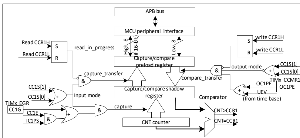
图 19-17 捕获/比较通道 1 主电路
