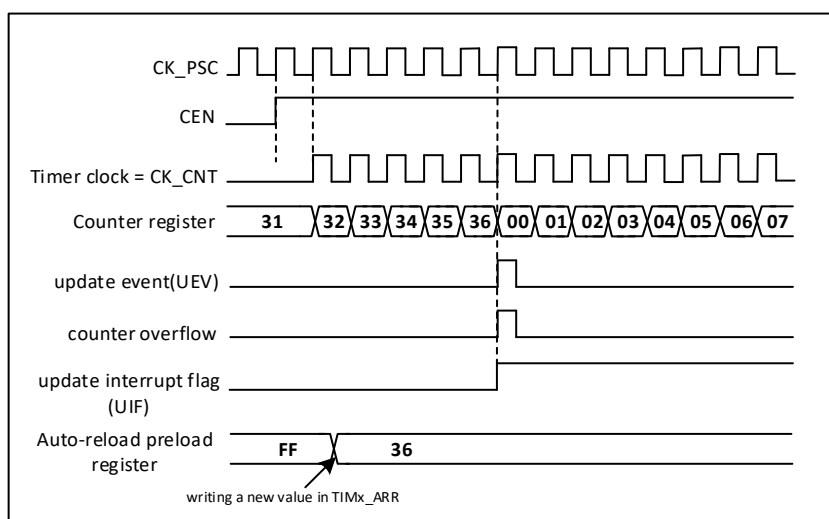
图 18-8 计数器时序图, ARPE=0 时更新事件 (TIMx_ARR 未预装载)
