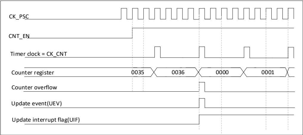
图 21-6 计数器时序图，内部时钟 4 分频
