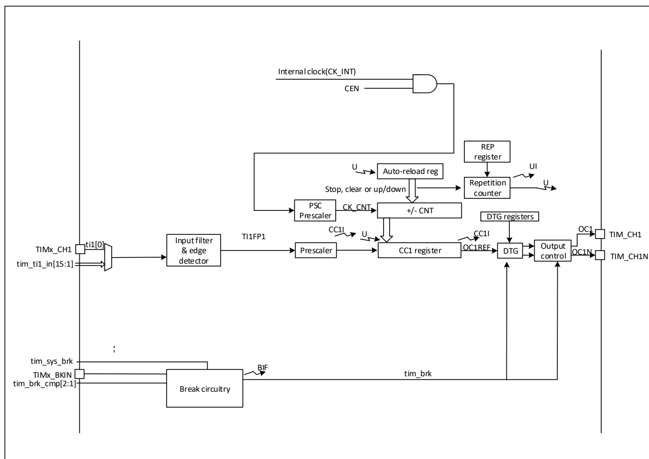
图 20-1 TIM16 和 TIM17 框图
