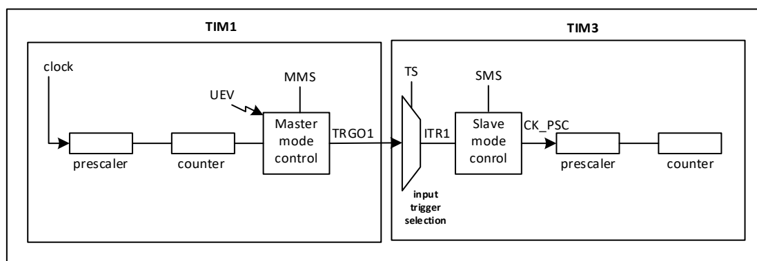
图 18-41 主/从定时器示例
