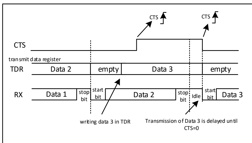
图 32-10 CTS 流控制
