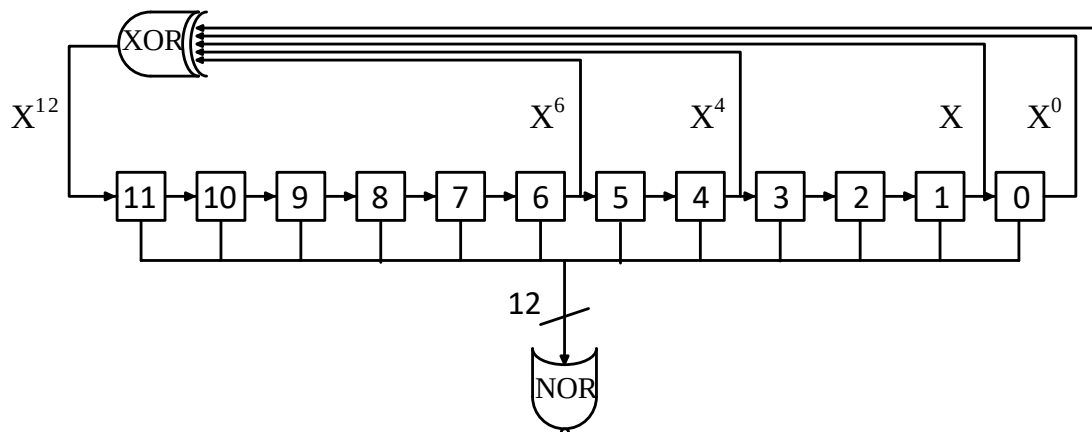
图 13-4 DAC LFSR 寄存器算法
