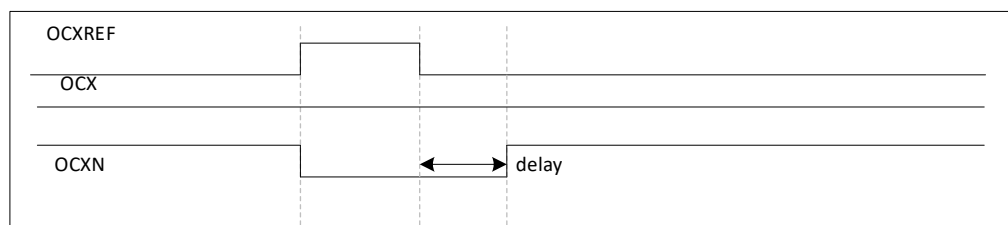
图 17-38 延迟时间大于正脉冲宽度的死区波形
