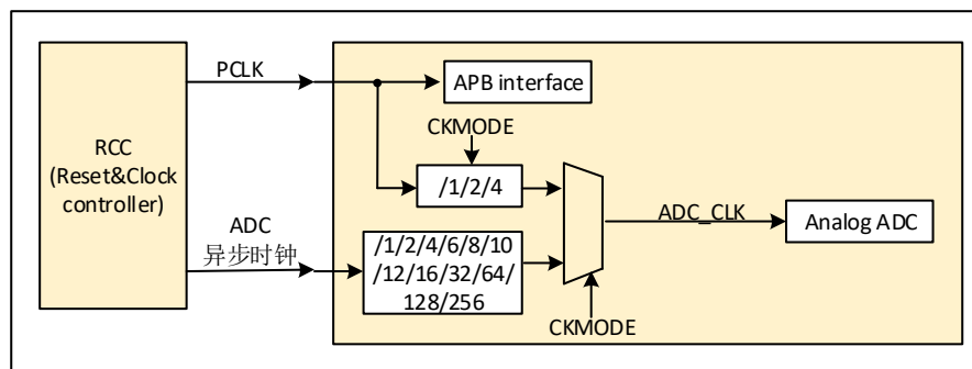
图 12-4 ADC 时钟结构
