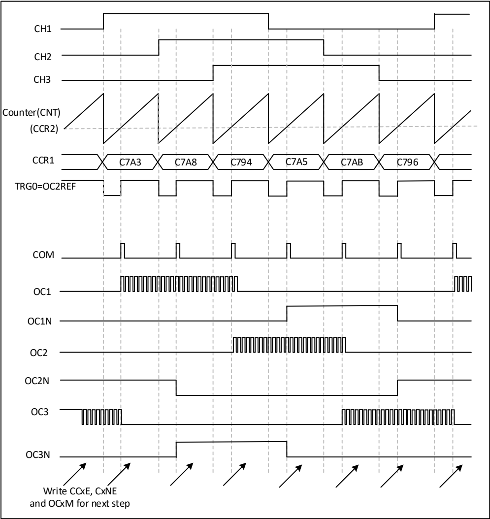
图 17-47 霍尔传感器示例
