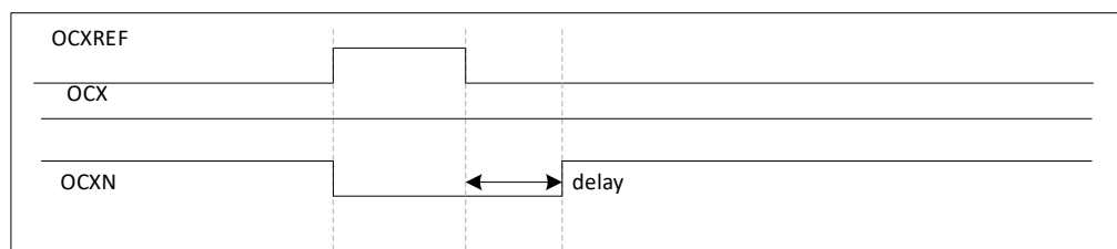
图 20-19 延迟时间大于正脉冲宽度的死区波形
