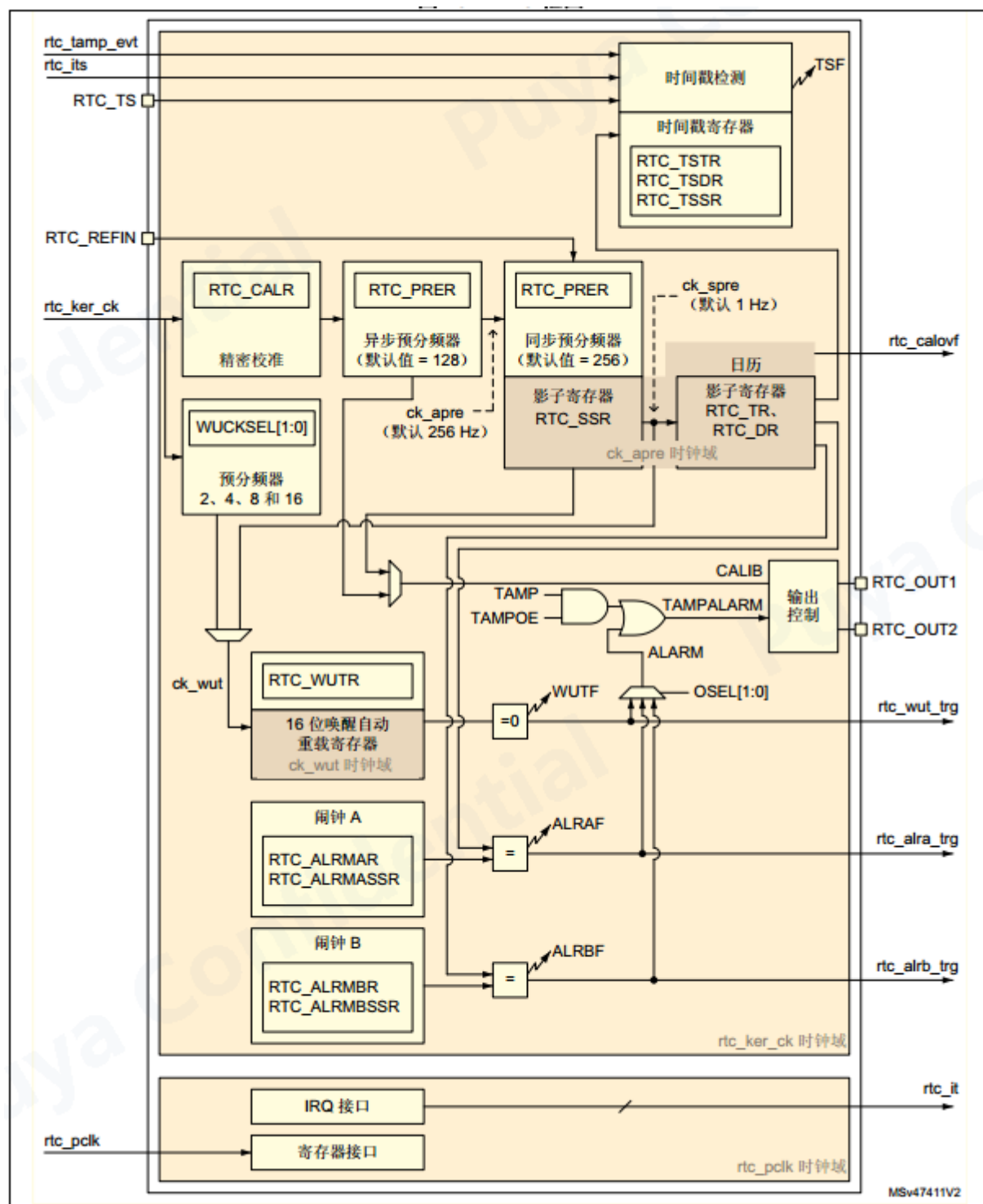
图 27-1 RTC 框图
