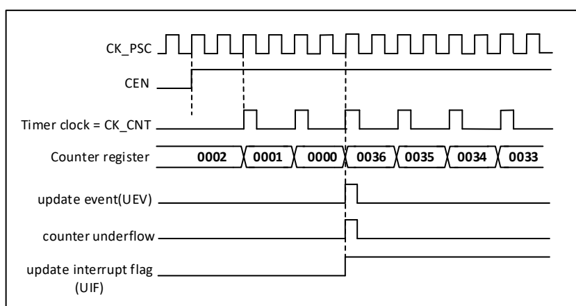
图 18-11 计数器时序图，内部时钟 2 分频
