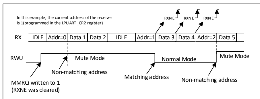
图 32-5 用地址标志检测的静默模式
