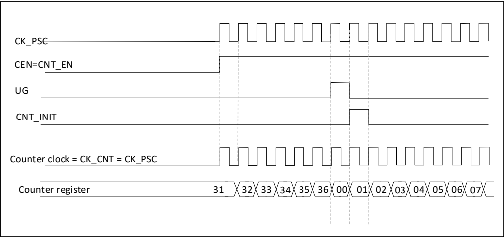
图 19-11 正常模式下的控制电路，内部时钟 1 分频
