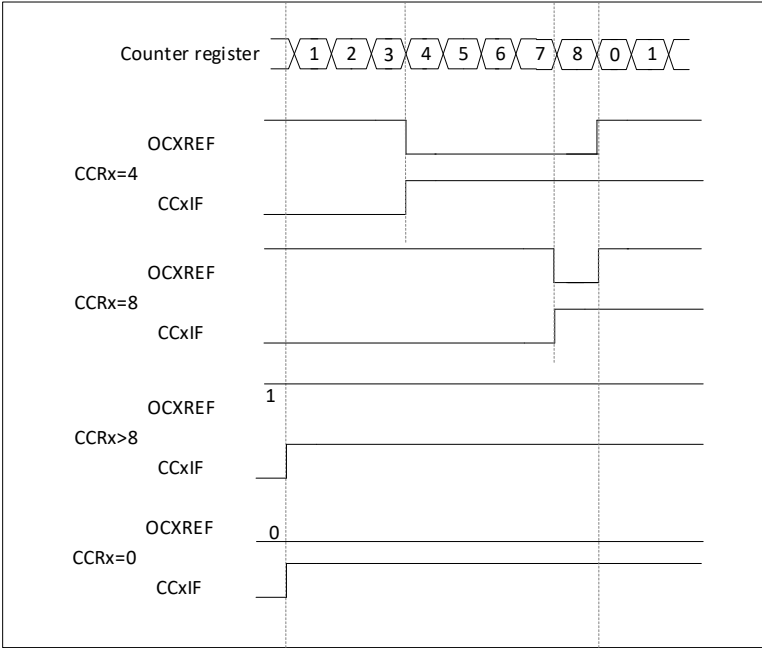
图 20-16 边沿对齐方式 PWM 输出波形 (ARR=8)
