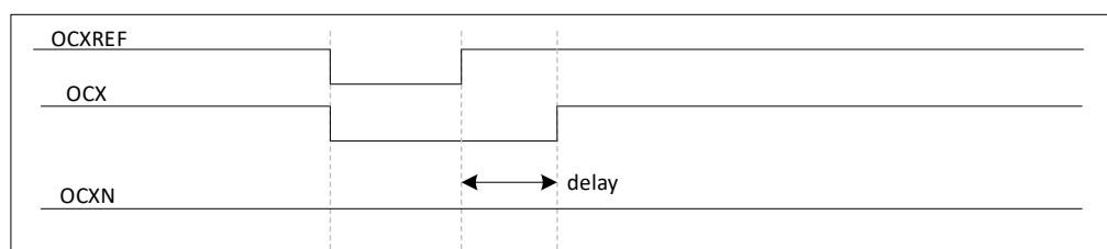
图 19-23 延迟时间大于负脉冲宽度的死区波形
