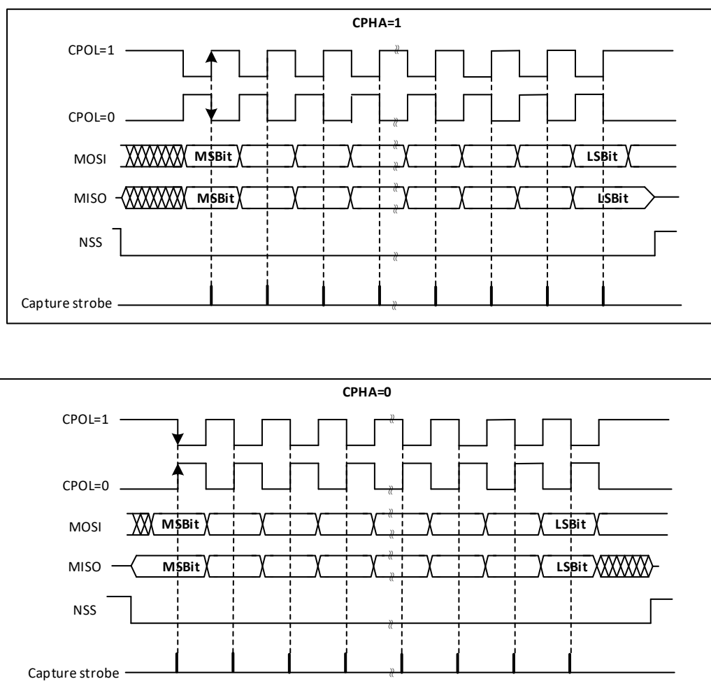
图 33-8 时钟/数据时序图
