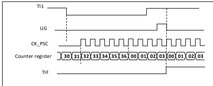
图 18-37 复位模式下的控制电路
