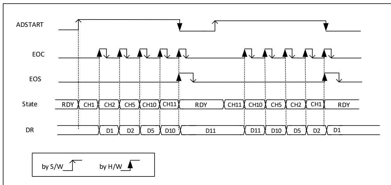
图 12-9 规则单次模式, 软件触发
