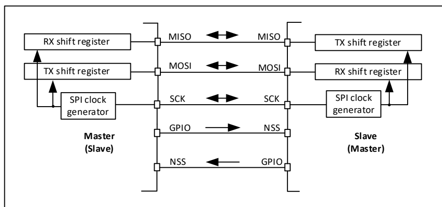
图 33-6 多主机应用
