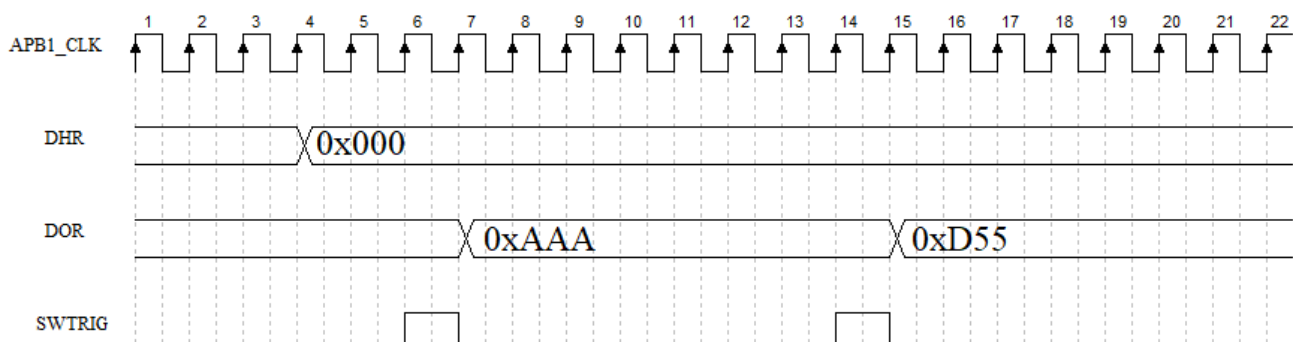
图 13-4 DAC LFSR 寄存器算法
