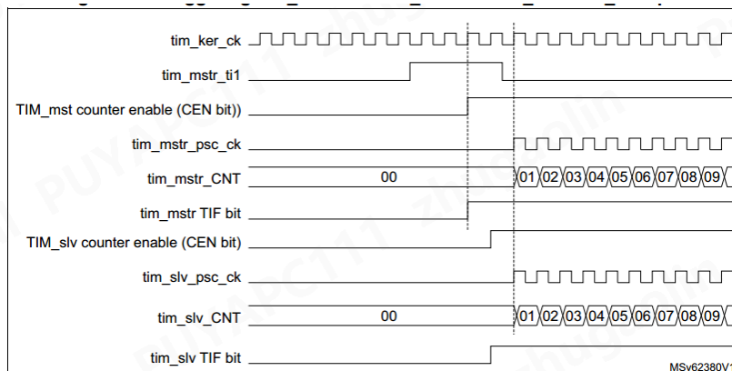
图 18-46 TIM1 的 TI1 触发 TIM1 和 TIM3
