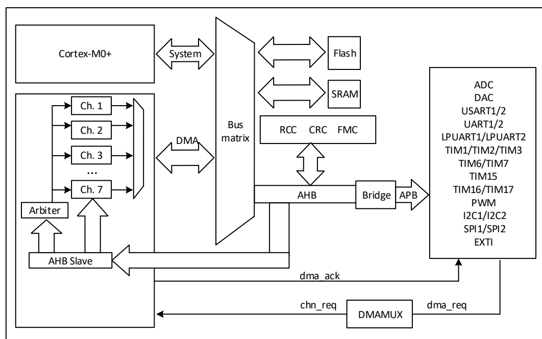
图 9-1 DMA 框图
