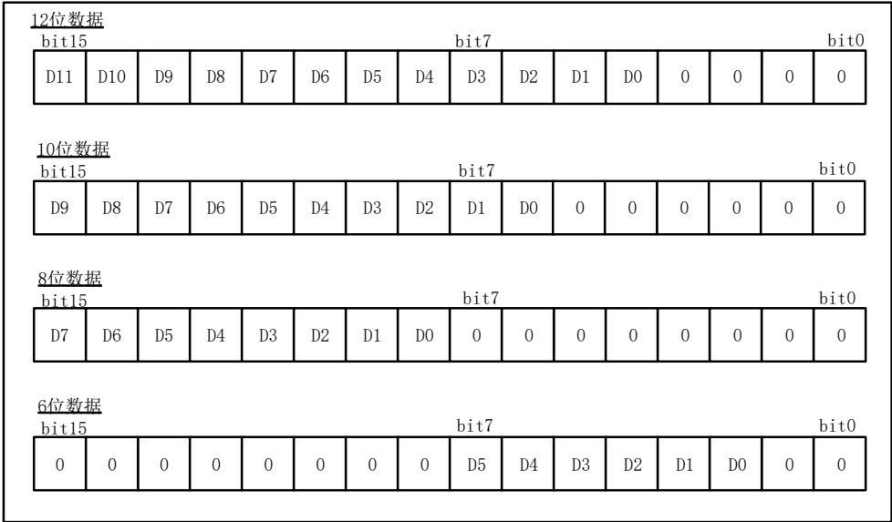
图 12-15 左对齐 (offset 未使能, 无符号数)
