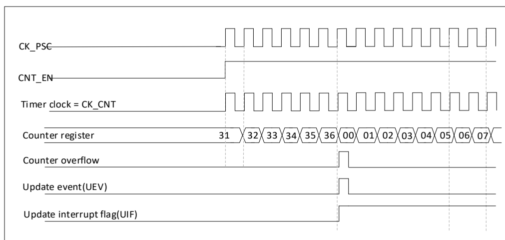
图 21-4 计数器时序图, 内部时钟 1 分频
