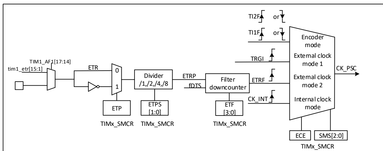
图 17-26 外部触发输入模块
