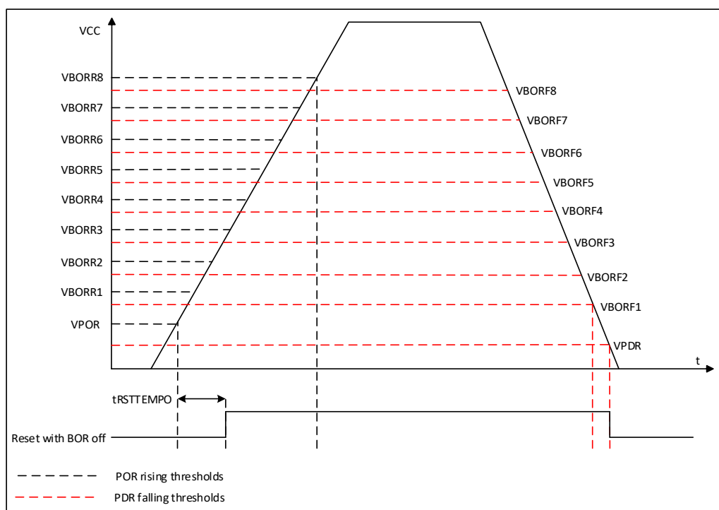
图 5-1 POR, PDR 阈值
