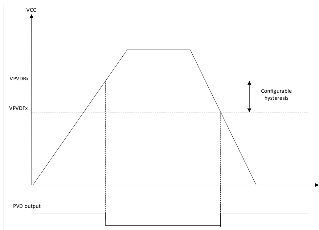
图 5-2 PVD 阈值
