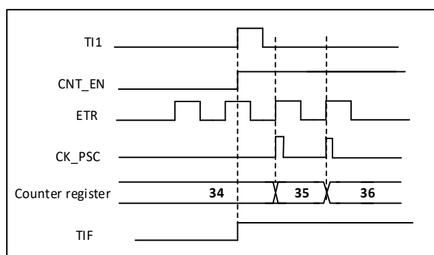
图 19-31 外部时钟模式 2+触发模式下的控制电路
