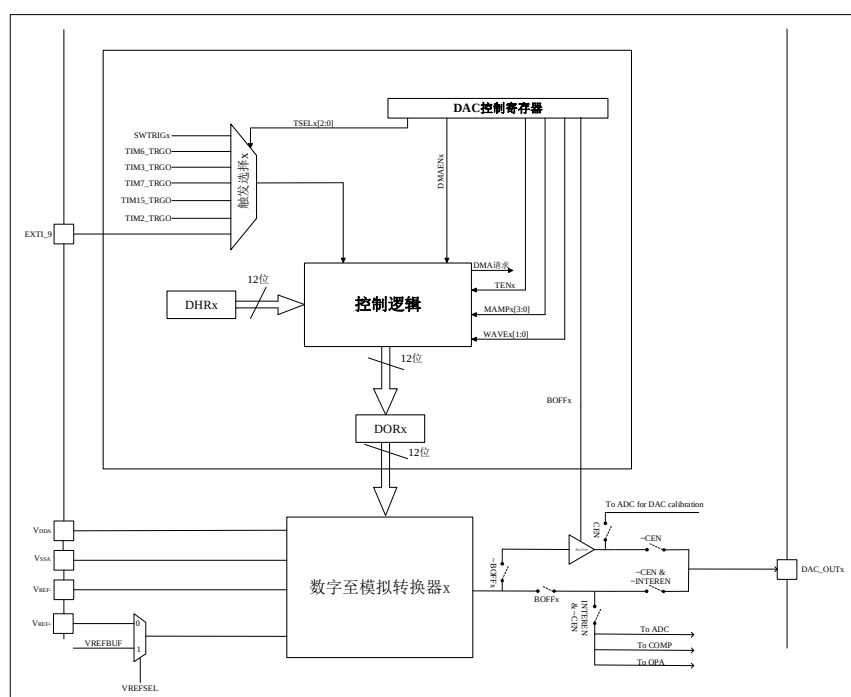
图 13-1 DAC 框图
