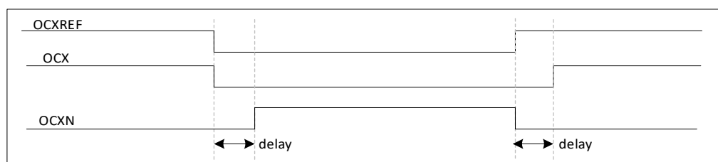
图 17-36 带死区插入的互补输出
