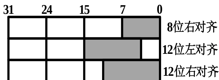
图 13-2 单 DAC 通道模式的数据寄存器
