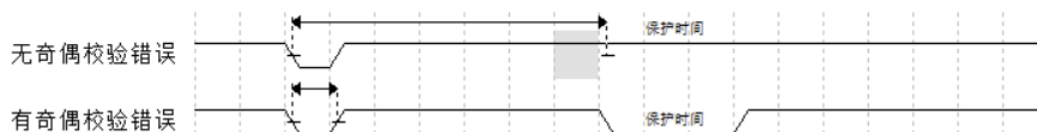
图 30-21 ISO7816-3 异步协议
