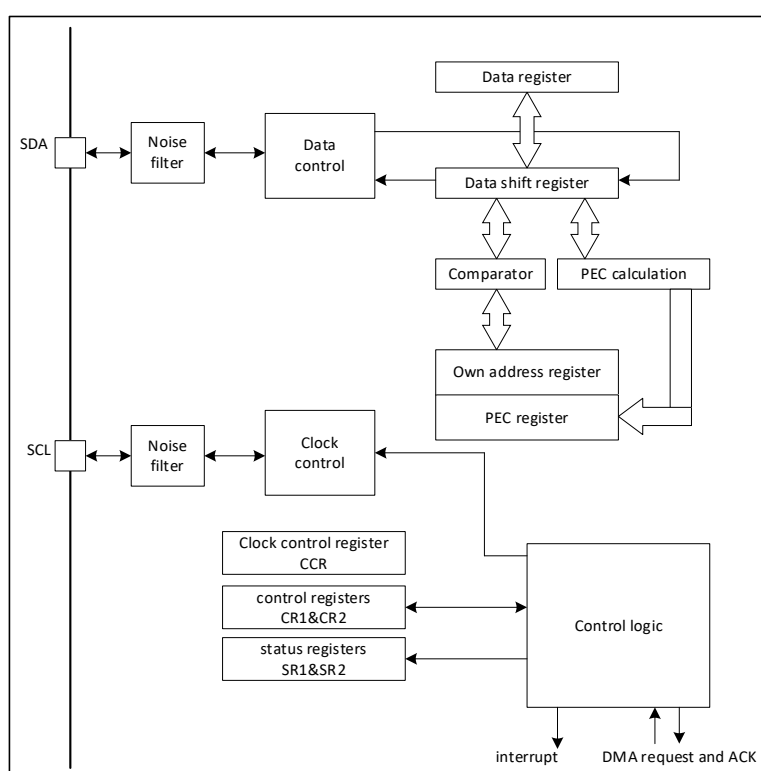
图 29-1 I 2 C 框图
