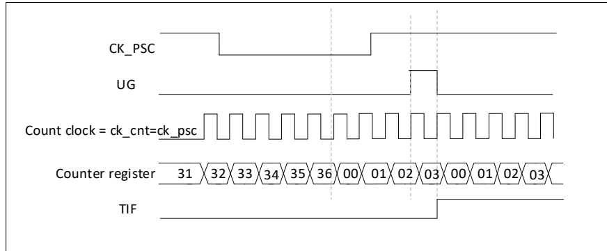
图 17-48 复位模式下的控制电路
