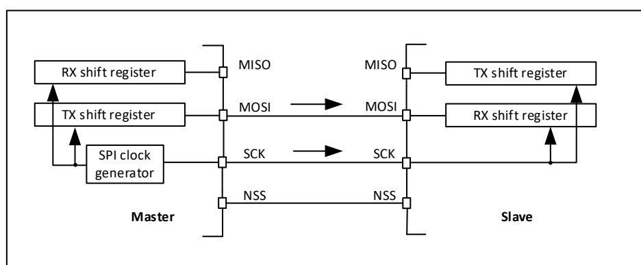
图 33-4 单工单主/从机应用 (主机只发送/从机只接收模式)
