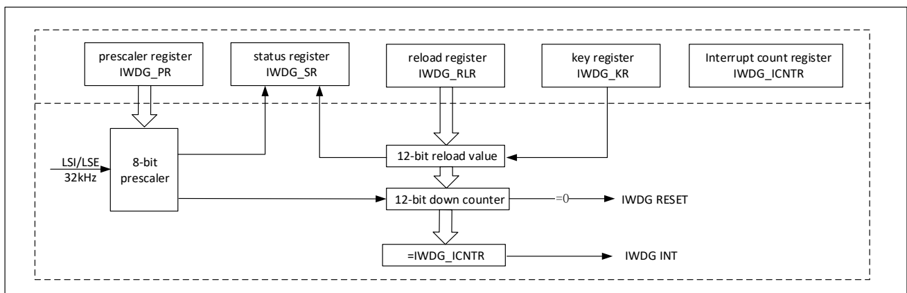
图 25-1 Independent watchdog 框图
