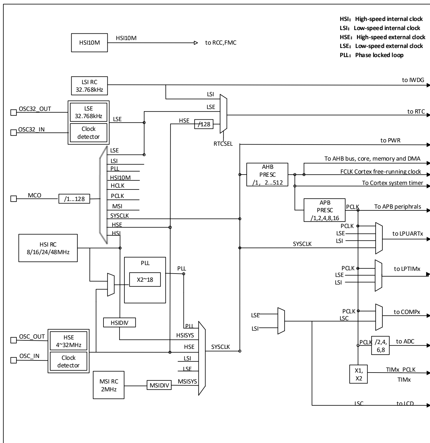
图 6-2 时钟结构
