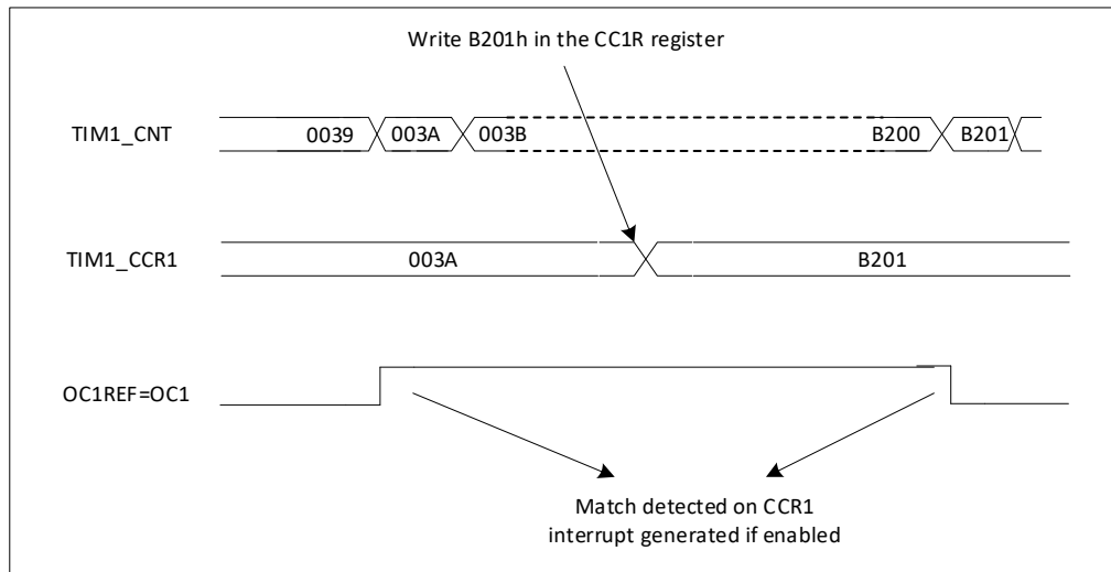
图 20-15 输出比较模式, 翻转 OC1
