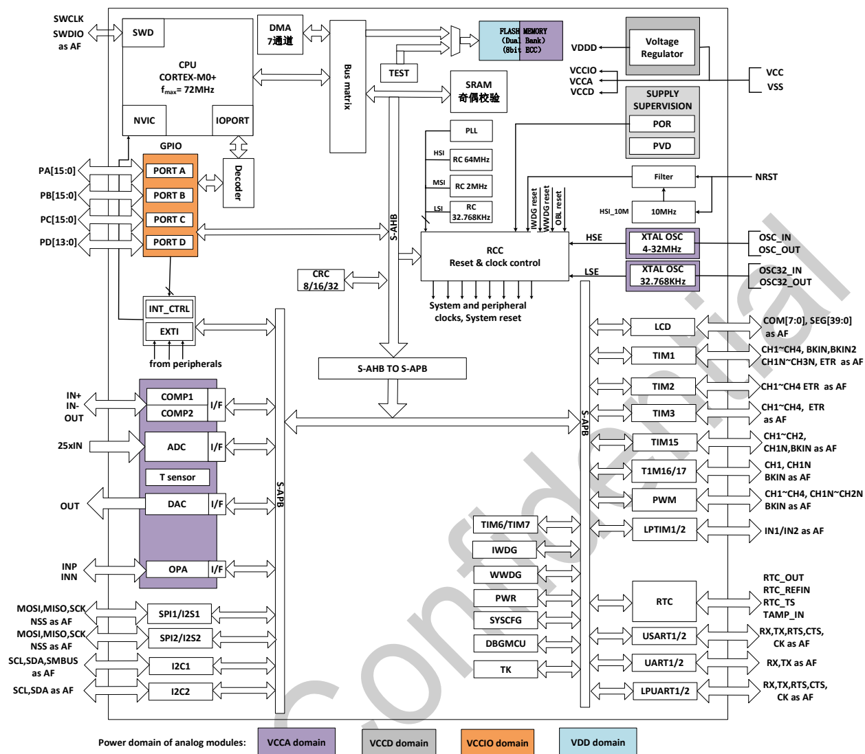
图 1-1 功能模块
