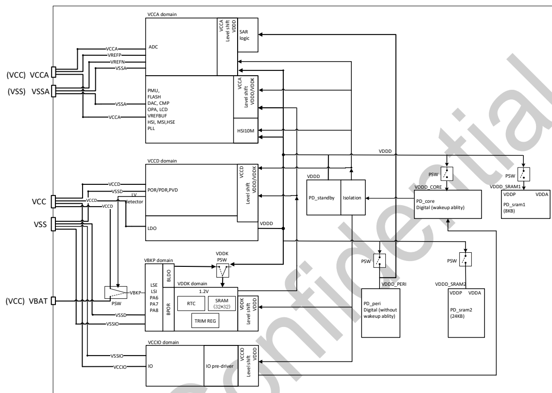
图 2-2 电源框图
