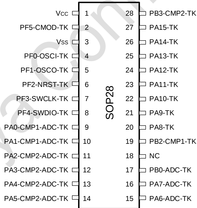
图 3-6 SOP28 Pinout4 PY32T020G4xS7-B (Top view)
