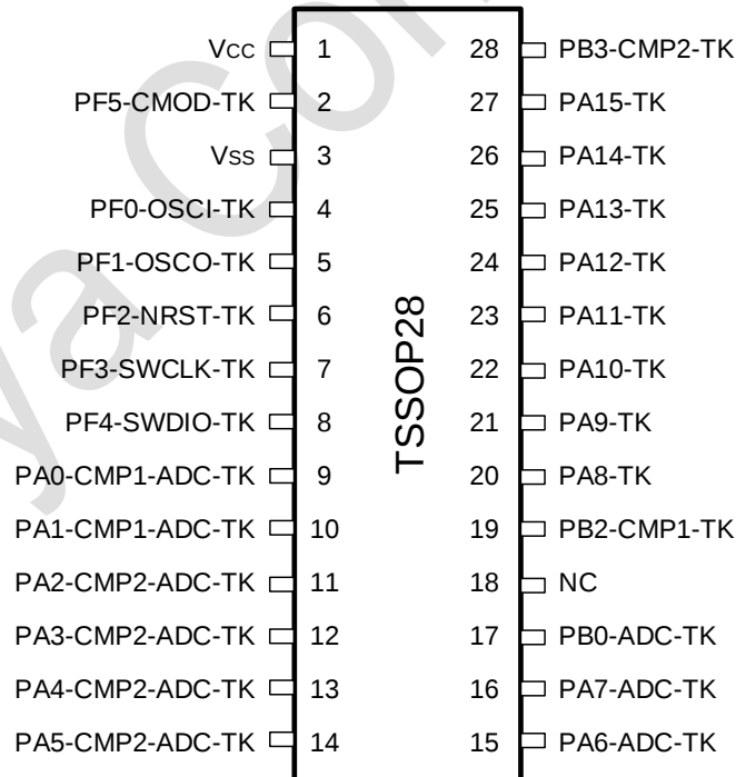
图 3-2 TSSOP28 Pinout4 PY32T020G4xP7-B (Top view)
