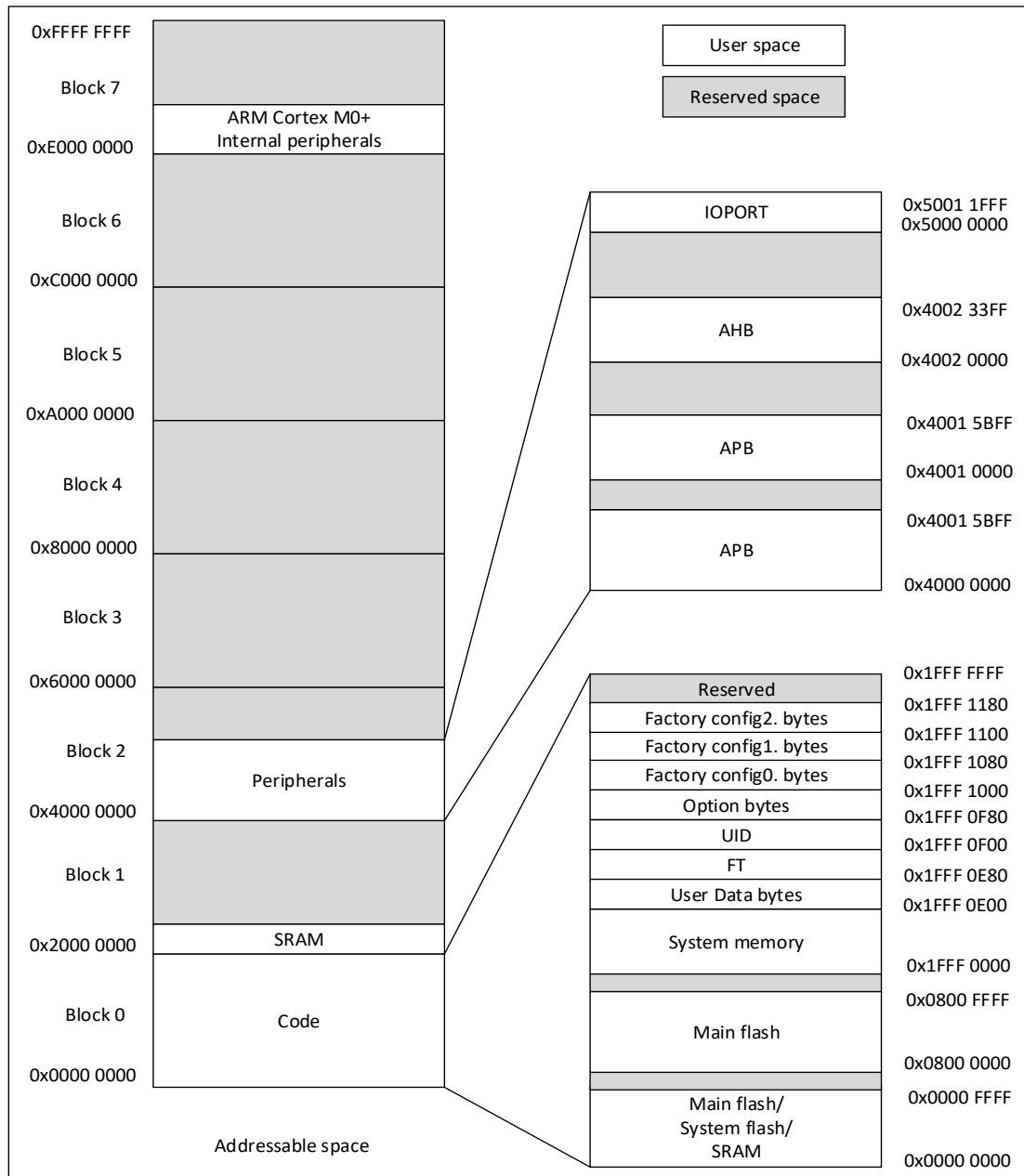
图 4-1 存储器映射
