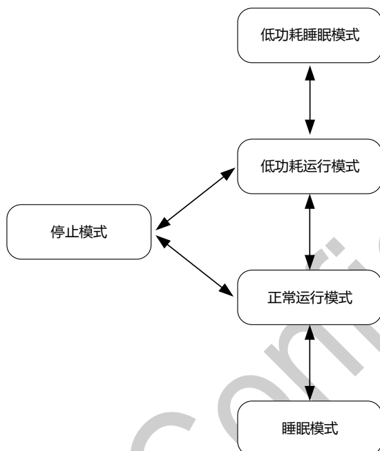
图 2-6 低功耗模式
