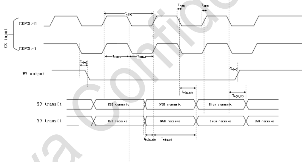
图 5-7 I 2 S 主模式时序图 (Philips 协议)
