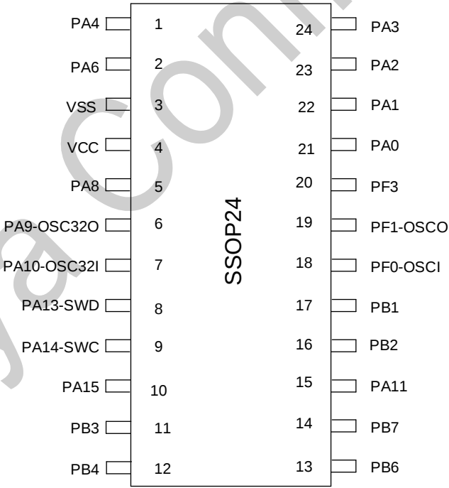
图 3-4 SSOP24 Pinout3 PY32F032E3xM7 / PY32F032E3xM7-B (Top view)
