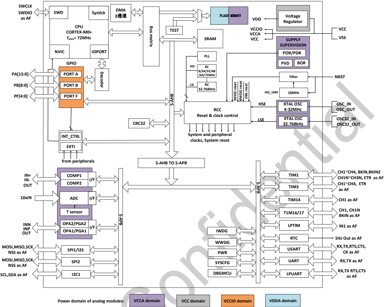
图 1-1 功能模块
