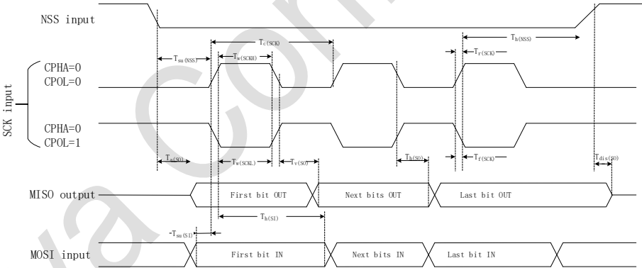
图 5-5 SPI 时序图-从模式且 CPHA = 0
