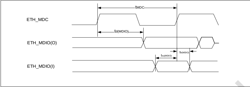
图 5-11 SMI 时序图
