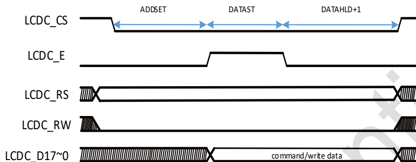
图 5-16 6800 模式写时序图
