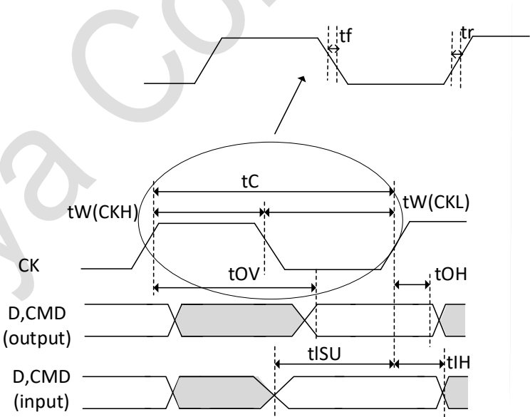
图 5-18 SDIO 高速模式
