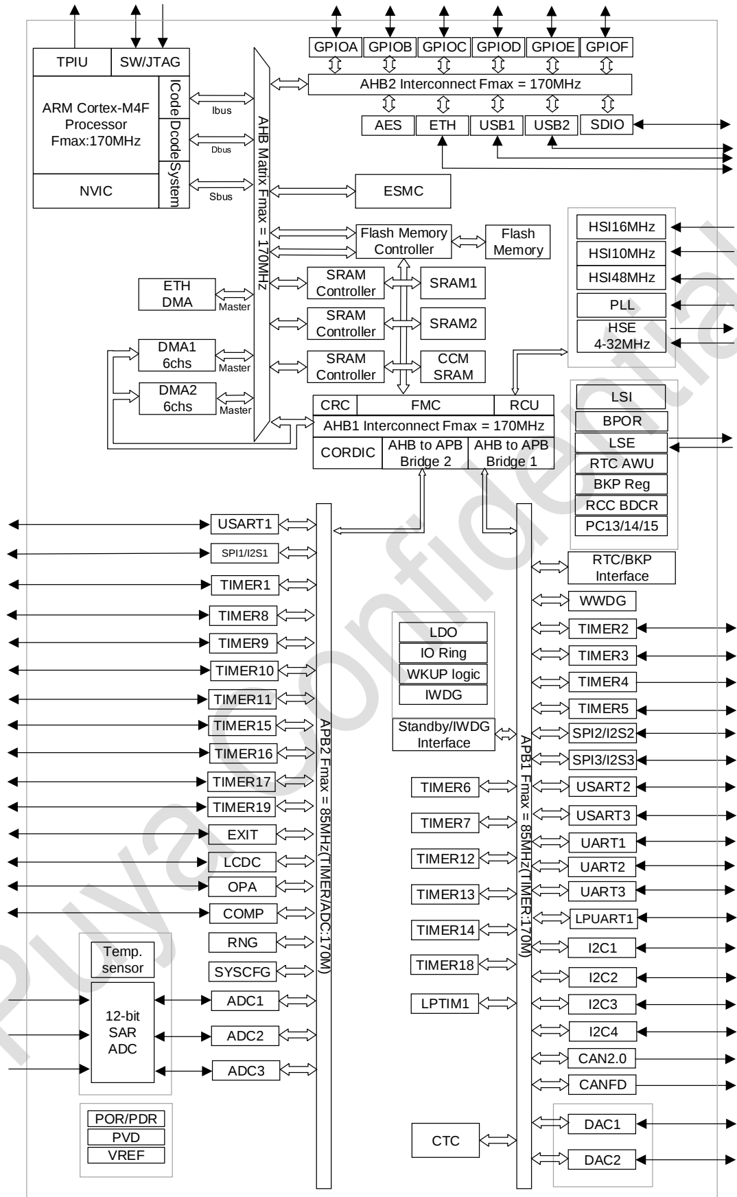
图 1-1 功能模块
