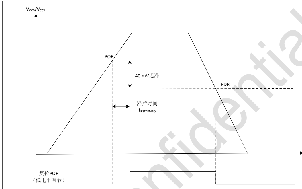
图 2-3 POR/PDR 阈值
