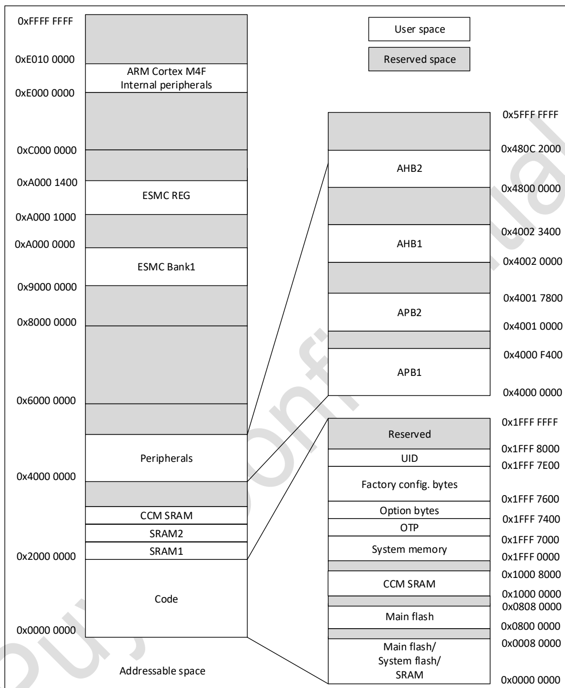
图 4-1 存储器映射
