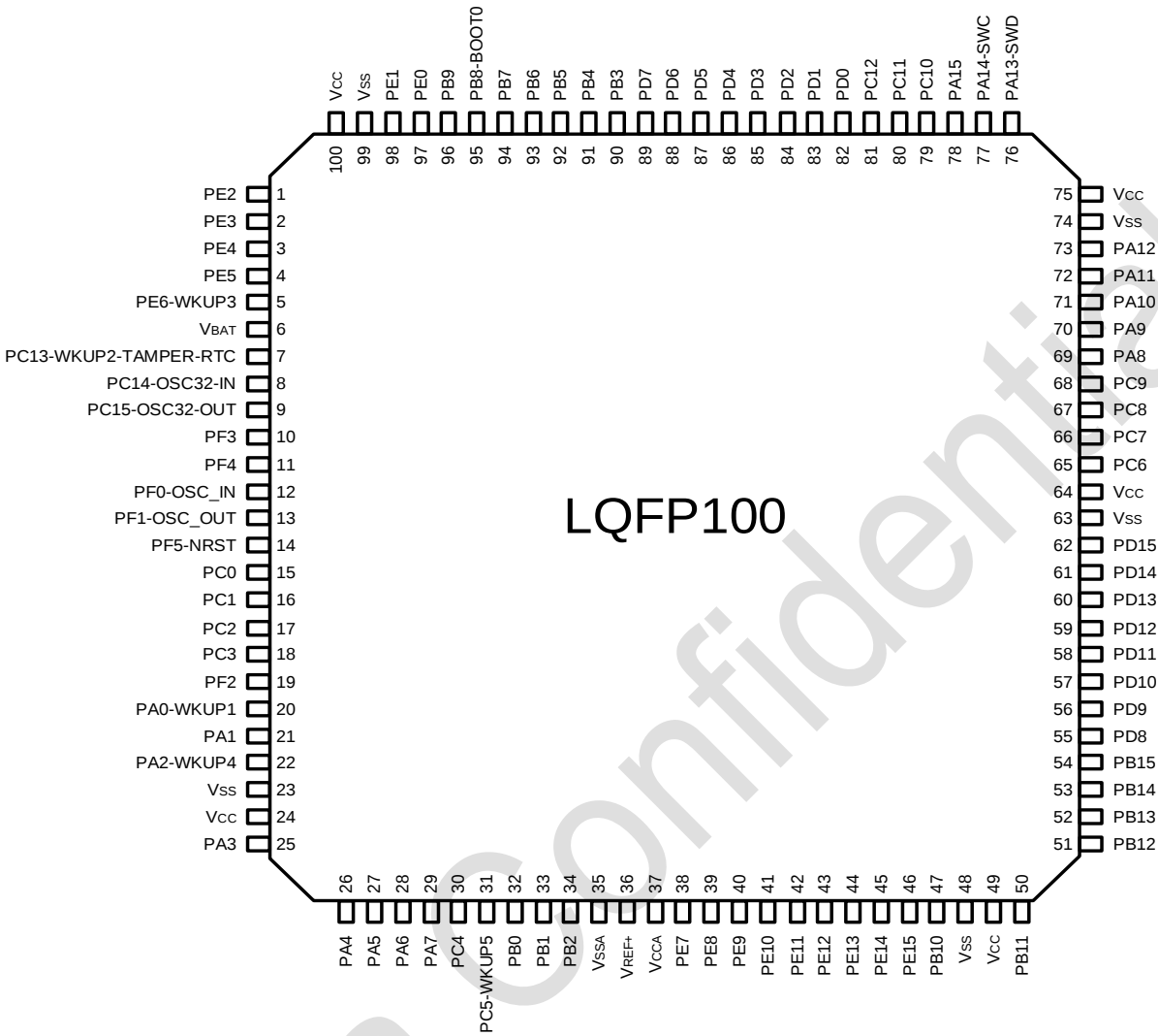
图 3-1 LQFP100 Pinout1 PY32E407V1ET7 (Top view)
