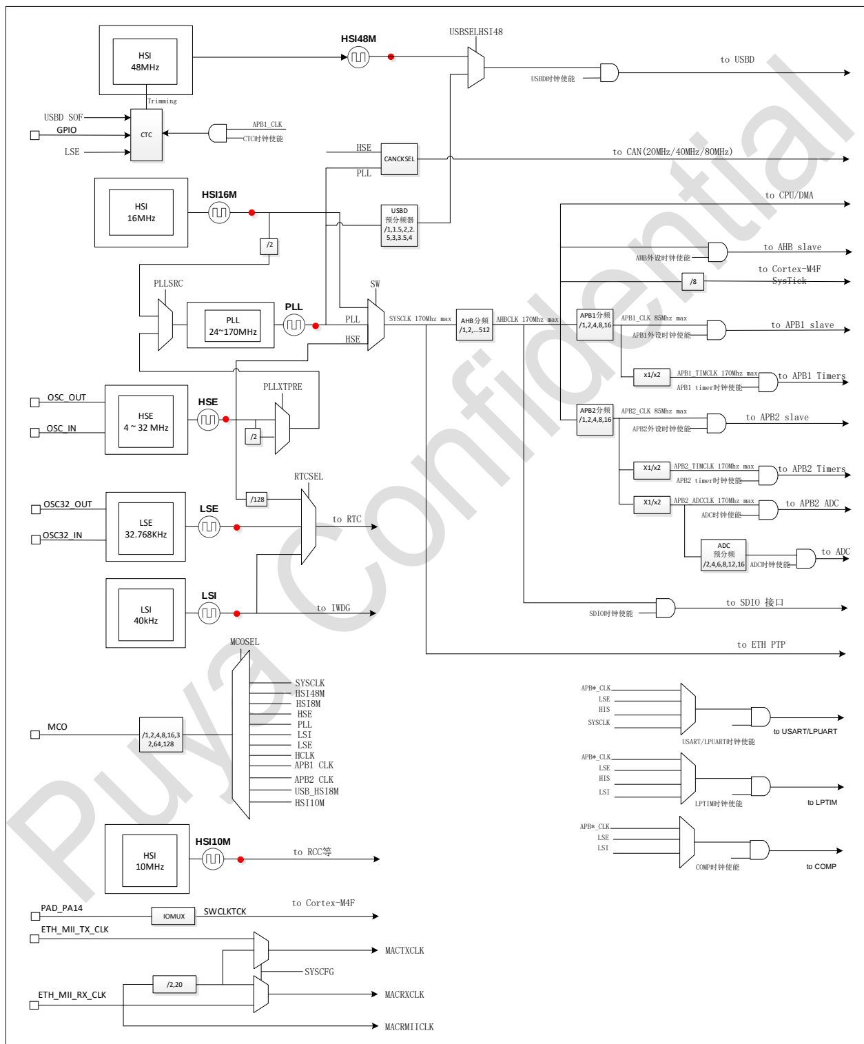
图 2-1 系统时钟结构图
