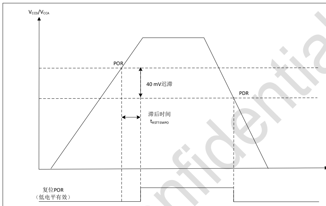
图 2-3 POR/PDR 阈值
