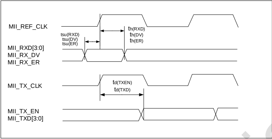
图 5-12 MII 时序图
