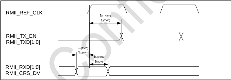
图 5-11 RMII 时序图
