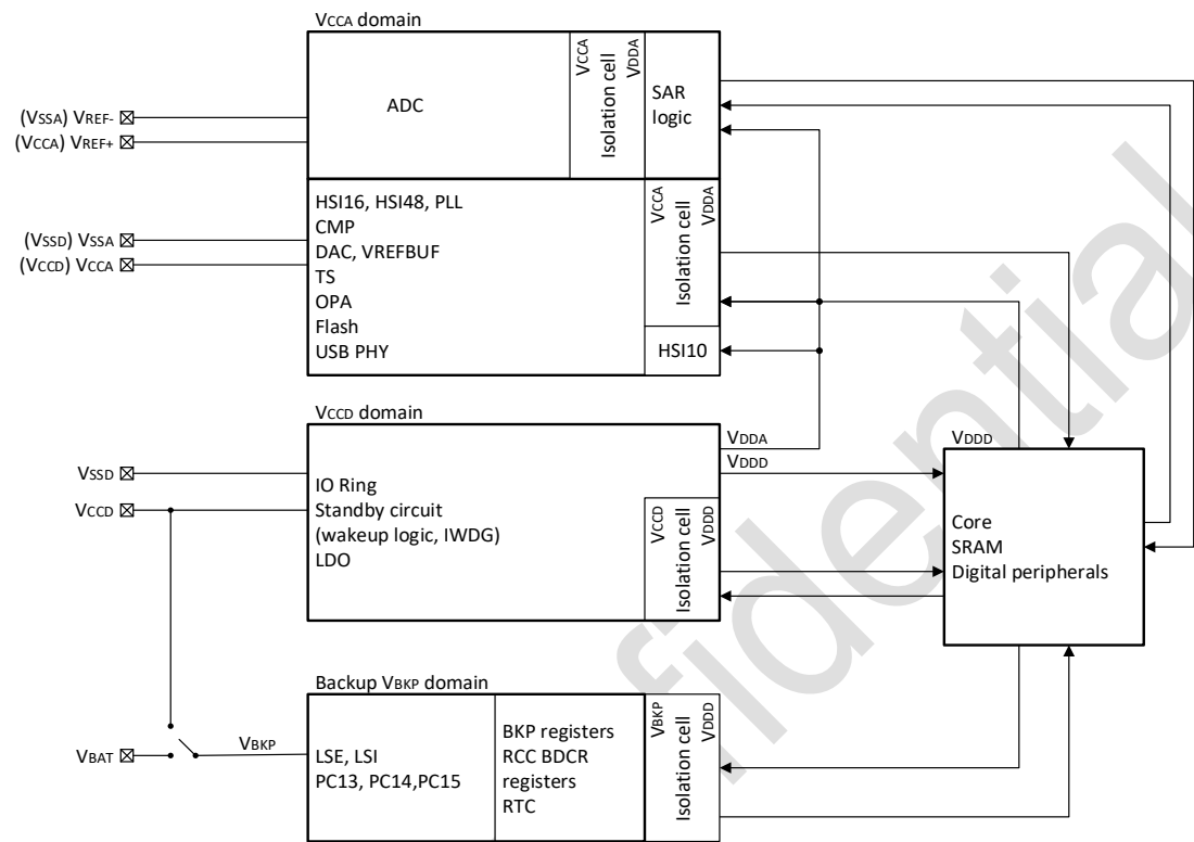
图 2-2 电源框图
