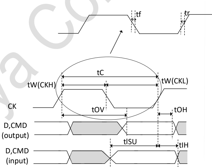
图 5-17 SDIO 高速模式
