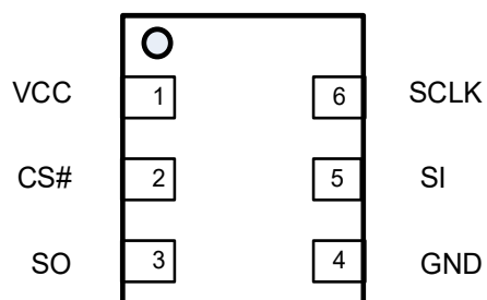
6-Pad USON(1.2x1.2mm)
