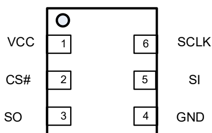
6-Pad USON(1.2x1.2mm)
