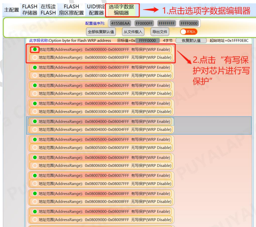
图 15-2 轩微操作 Option 写保护
